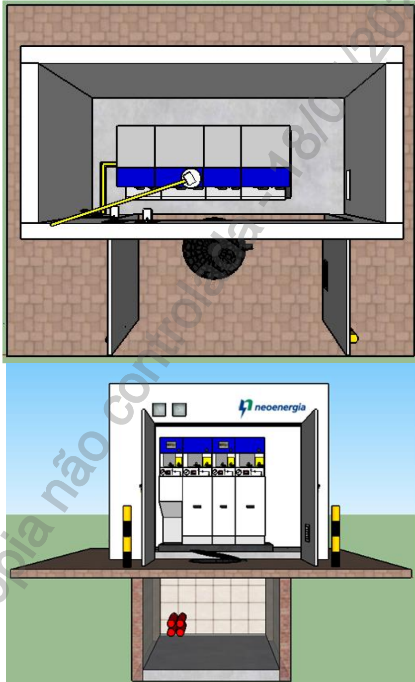
Desenho 14 - Câmara de Manobra - 5/7 (CM-R-RE+2P/ CM-R-RE+3P/CM-A-3L/ CM-A-4L)
