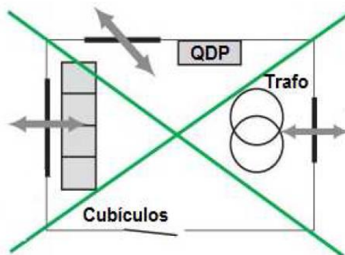
Figura 3 – Aberturas de Ventilação Natural Sem Cruzamento
