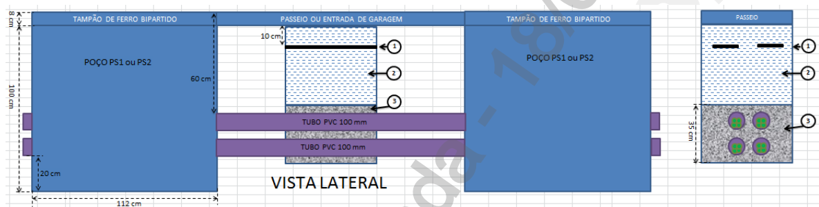
Eletrودuto de PVC em passeio ou entrada de garagem
