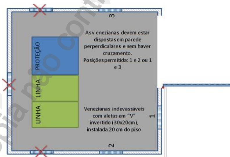
Figura 8 – Posição das Venezianas
