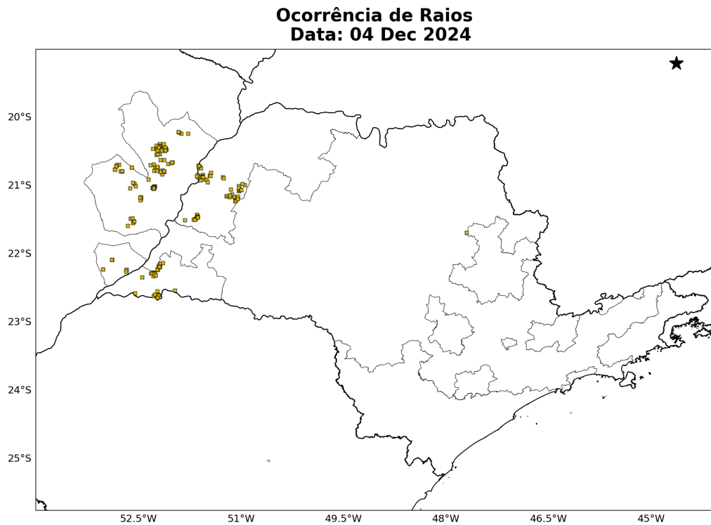
Figura 7: Densidade de descargas atmosféricas nuvem-solo detectadas pelo sistema Earth Networks para o dia 04 dezembro sobre a área de concessão da Neoenergia-Elektro.
