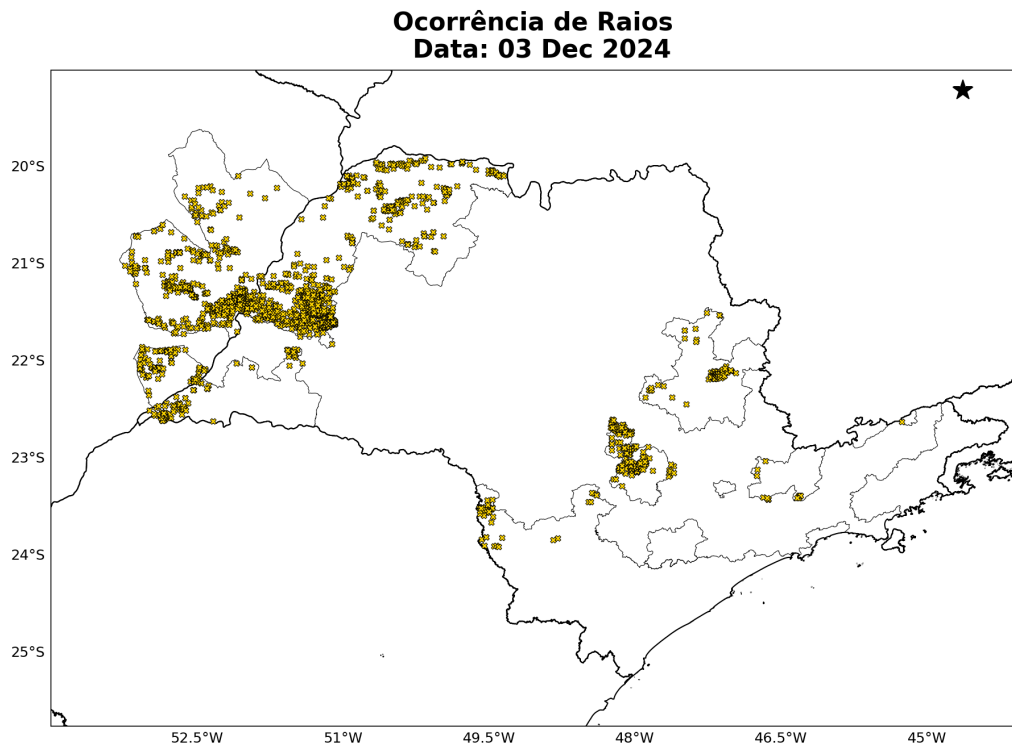
Figura 6: Densidade de descargas atmosféricas nuvem-solo detectadas pelo sistema Earth Networks para o dia 03 dezembro sobre a área de concessão da Neoenergia-Elektro.
