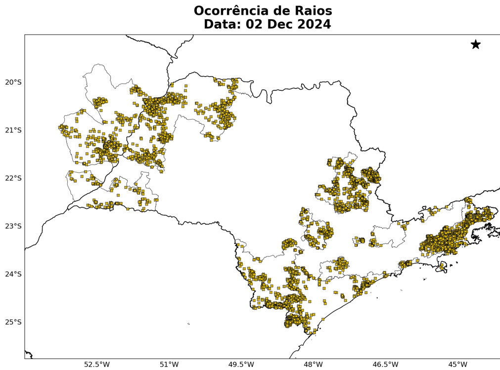
Figura 5: Densidade de descargas atmosféricas nuvem-solo detectadas pelo sistema Earth Networks para o dia 02 dezembro sobre a área de concessão da Neoenergia-Elektro.
