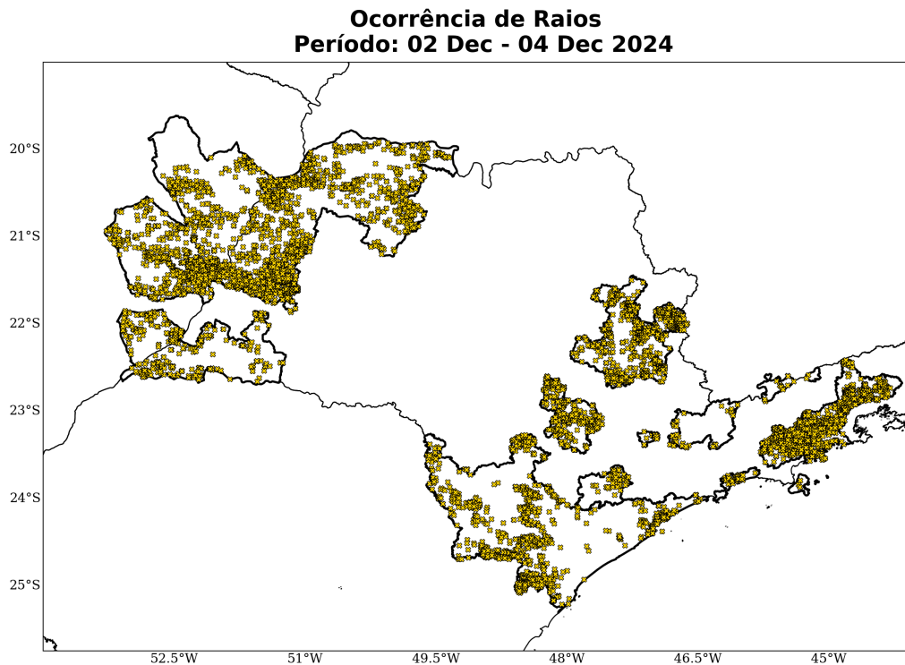
Figura 8: Densidade de descargas atmosféricas nuvem-solo detectadas pelo sistema Earth Networks para o período 02 a 04 de dezembro de 2024 sobre a área de concessão da Neoenergia-Elektro.
