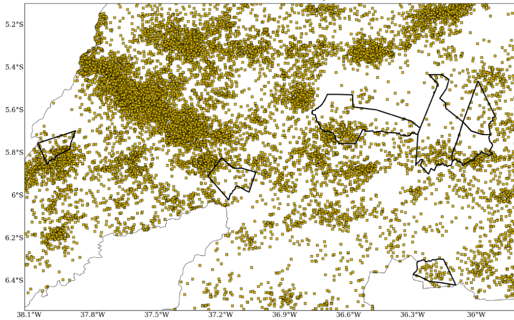
Figura 4 - Densidade de descargas atmosféricas nuvem-solo detectadas pelo sistema Earth Networks para o período de 28 de março a 04 de abril de 2024 sobre o município de Severiano Melo e seus arredores.
