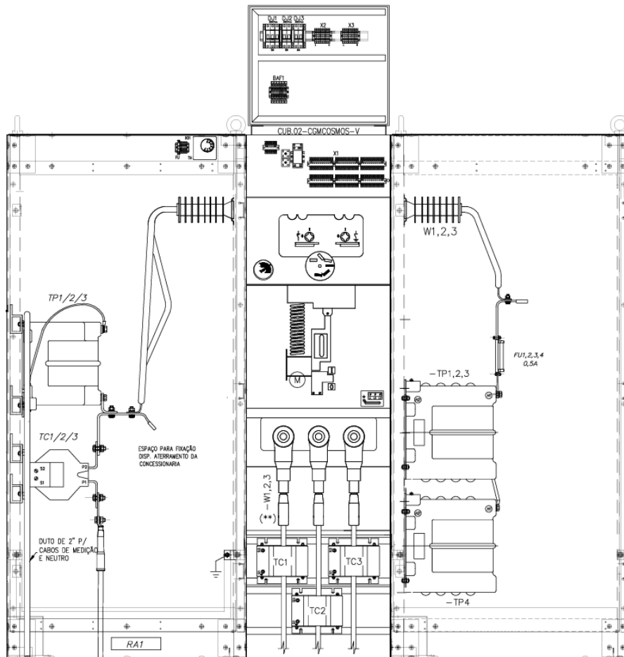
Figura 37 – Medição e Proteção até 300 kVA com Transformadores Auxiliares
