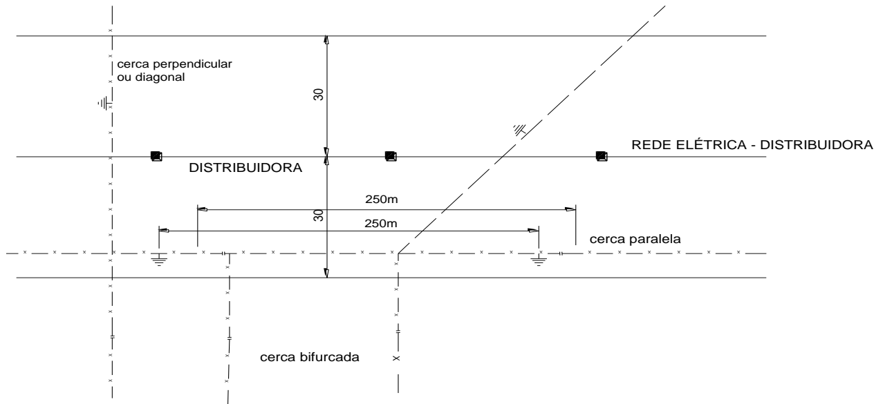
Figura 10 – Seccionamento de Cerca
