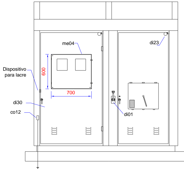
Figura 27 – Conjunto Blindado para Medição e Proteção em AT (1/2) Vista de frente (sem portas externas)
