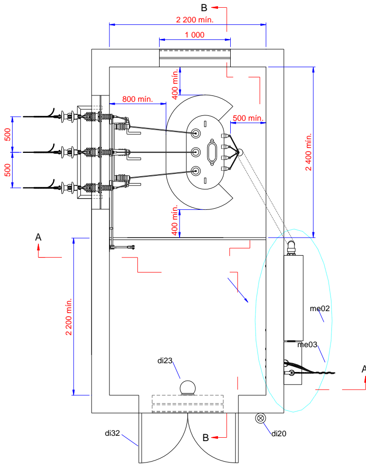
Figura 18 – Subestação Abrigada de Transformação Entrada Aérea – Medição BT (1/3)
