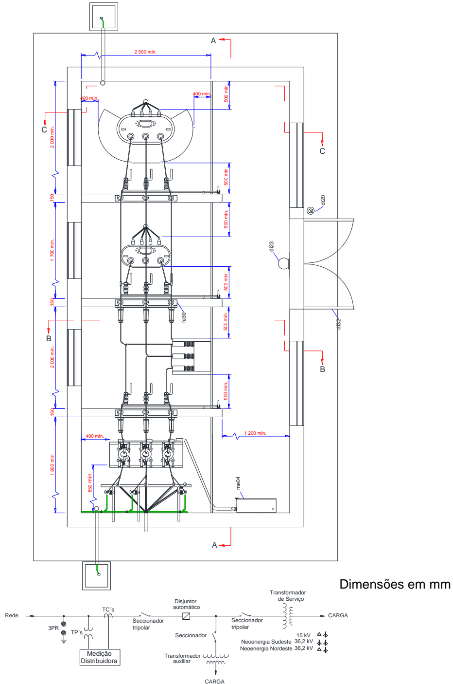
Figura 25 – Subestação Abrigada de Medição, Proteção e Transformação – Entrada Subterrânea – Medição em AT (1/4)
