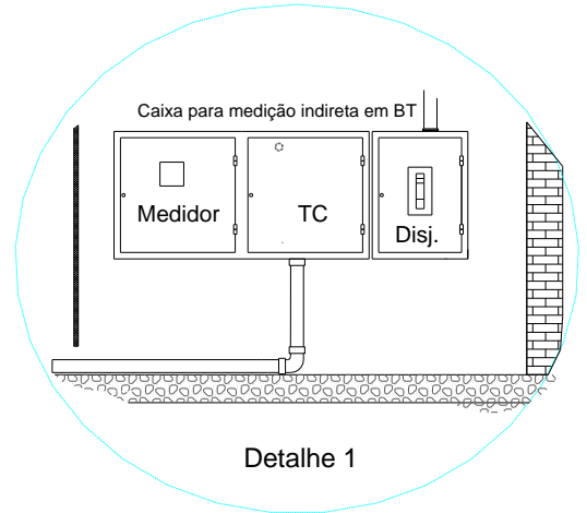
Figura 18 – Subestação Abrigada de Transformação Entrada Aérea – Medição BT (1/3)
