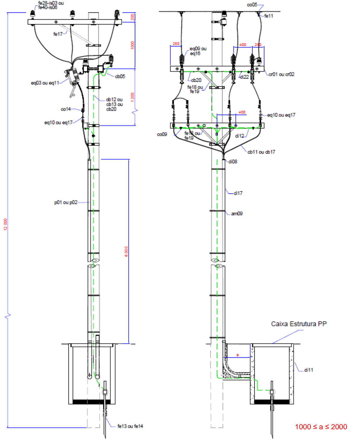
Figura 3 – Ramal de Entrada Subterrâneo – Derivação Rede Convencional
