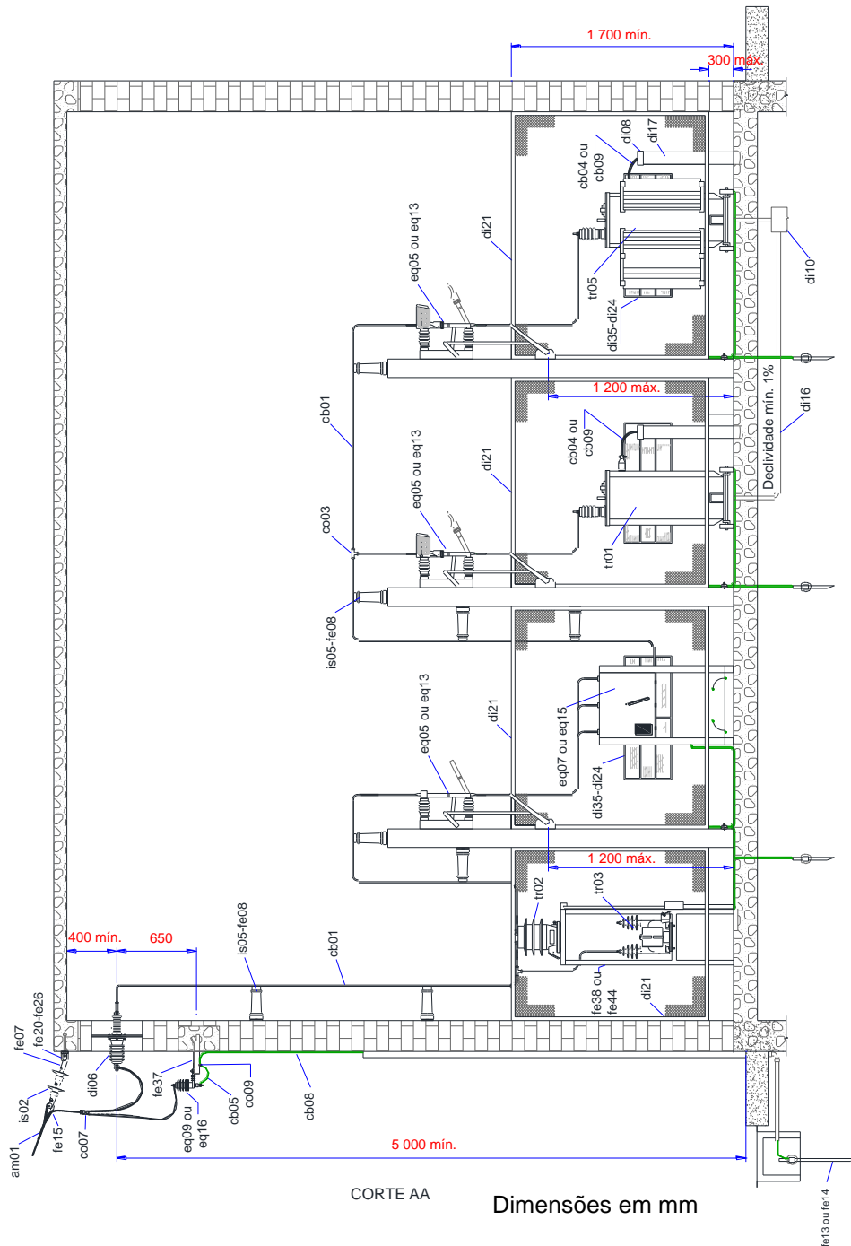
Figura 24 – Subestação Abrigada de Medição, Proteção e Transformação – Entrada Aérea – Medição em AT (2/4)
