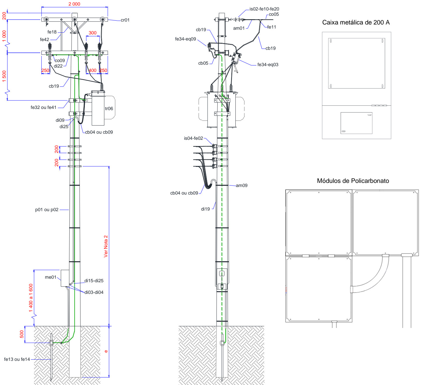
Figura 14 – Posto de Transformação em Poste – 13,8 kV (Medição Direta)
