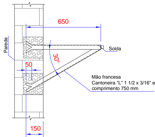
Corte AA
