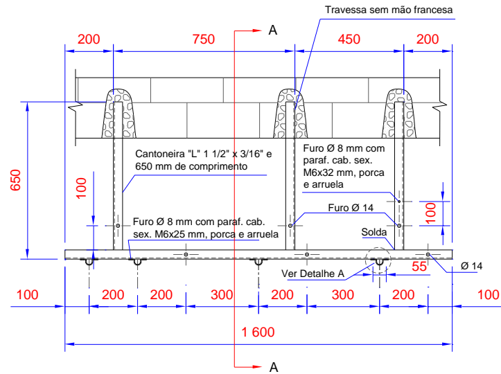
Figura 31 – Suporte para Terminais Poliméricos, Para-raios e Chaves Fusíveis
