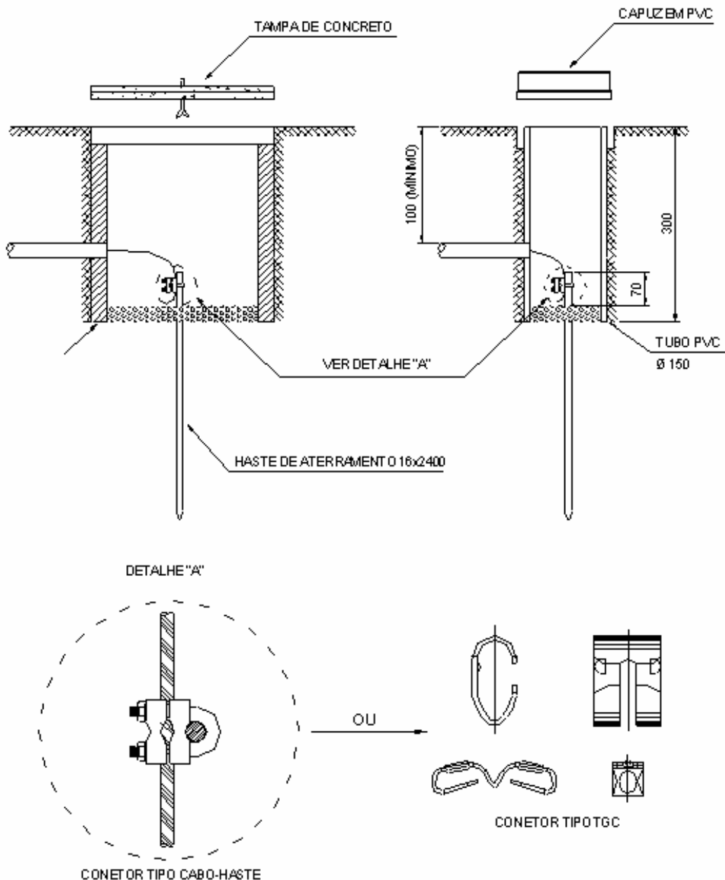
Figura 32 – Detalhamento Aterramento
