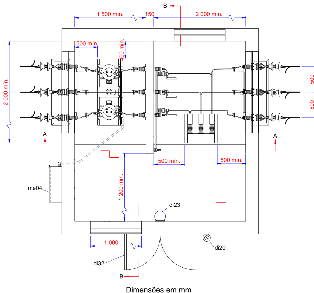
Figura 22 – Subestação Abrigada de Medição e Proteção Entrada Aérea – Medição AT (1/3)
