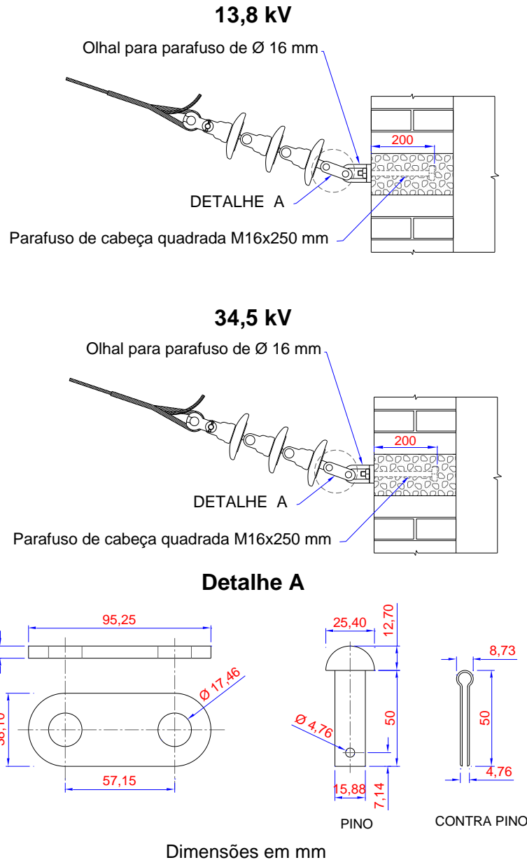
Figura 29 – Detalhes Construtivos em Subestações – Fixação da Cadeia de Isoladores (2/4)
