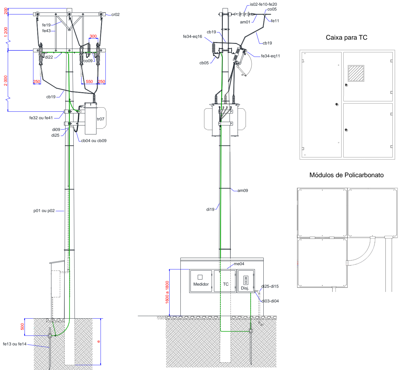
Figura 17 – Posto de Transformação em Poste 36,2 kV (Medição Indireta) (1/2)
