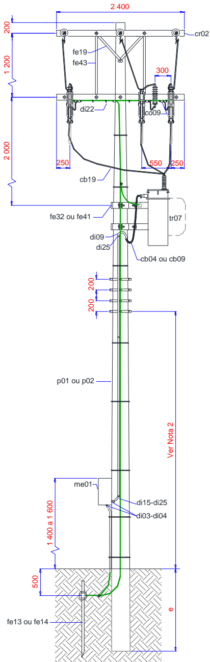
Figura 15 – Posto de Transformação em Poste – 36,2 kV (Medição Direta)
