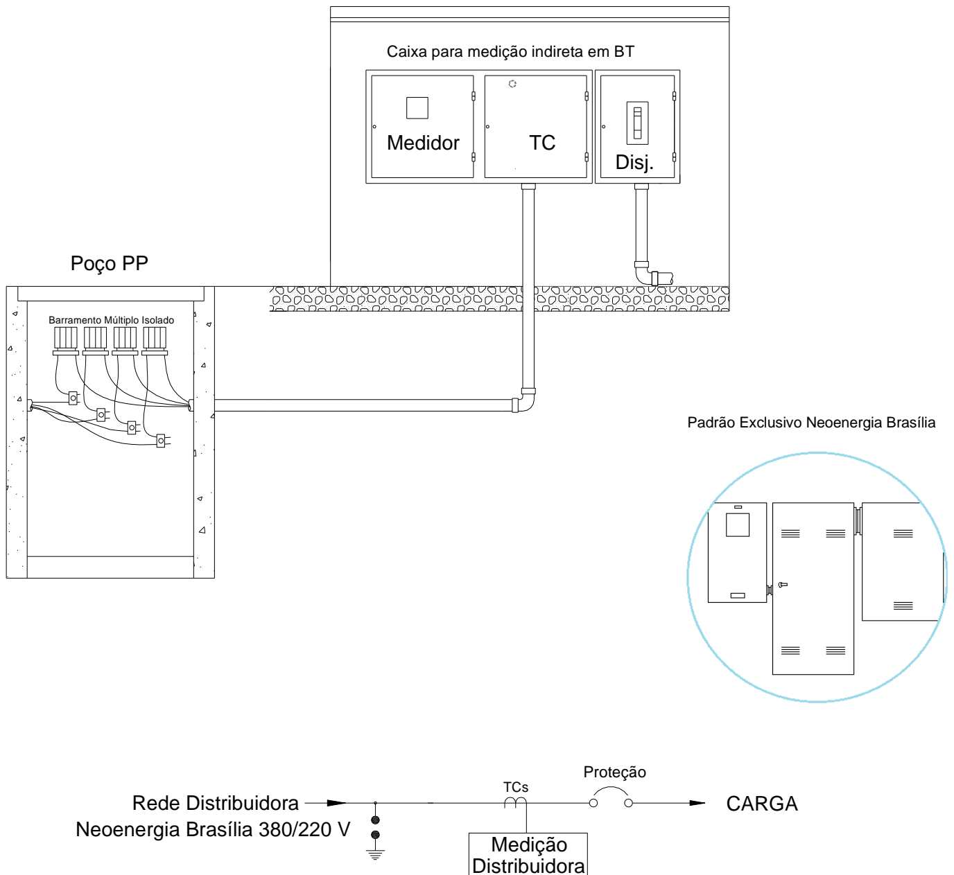
Figura 19 – Padrão de Entrada de Consumidores AS Localizados em Áreas Específicas do Distrito Federal
