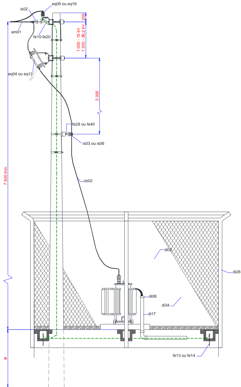
Figura 28 – Subestação ao Tempo Acima de 300 kVA – Entrada Aérea (3/3)
