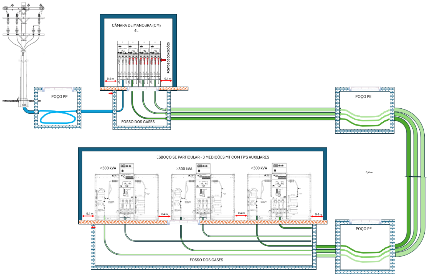
Esquema 6: Câmara de Manobra, Subestação Particular Compartilhada com 3 Clientes com Medição MT e Transformadores Auxiliares
