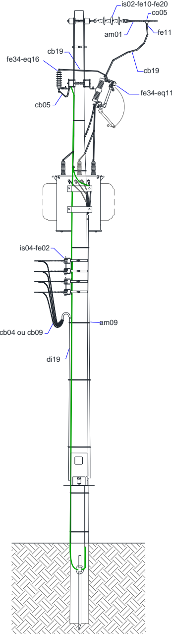
Figura 15 – Posto de Transformação em Poste – 36,2 kV (Medição Direta)
