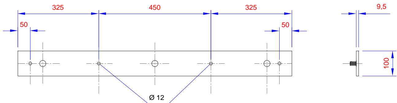
Figura 30 – Suporte para Isolador Pedestal
