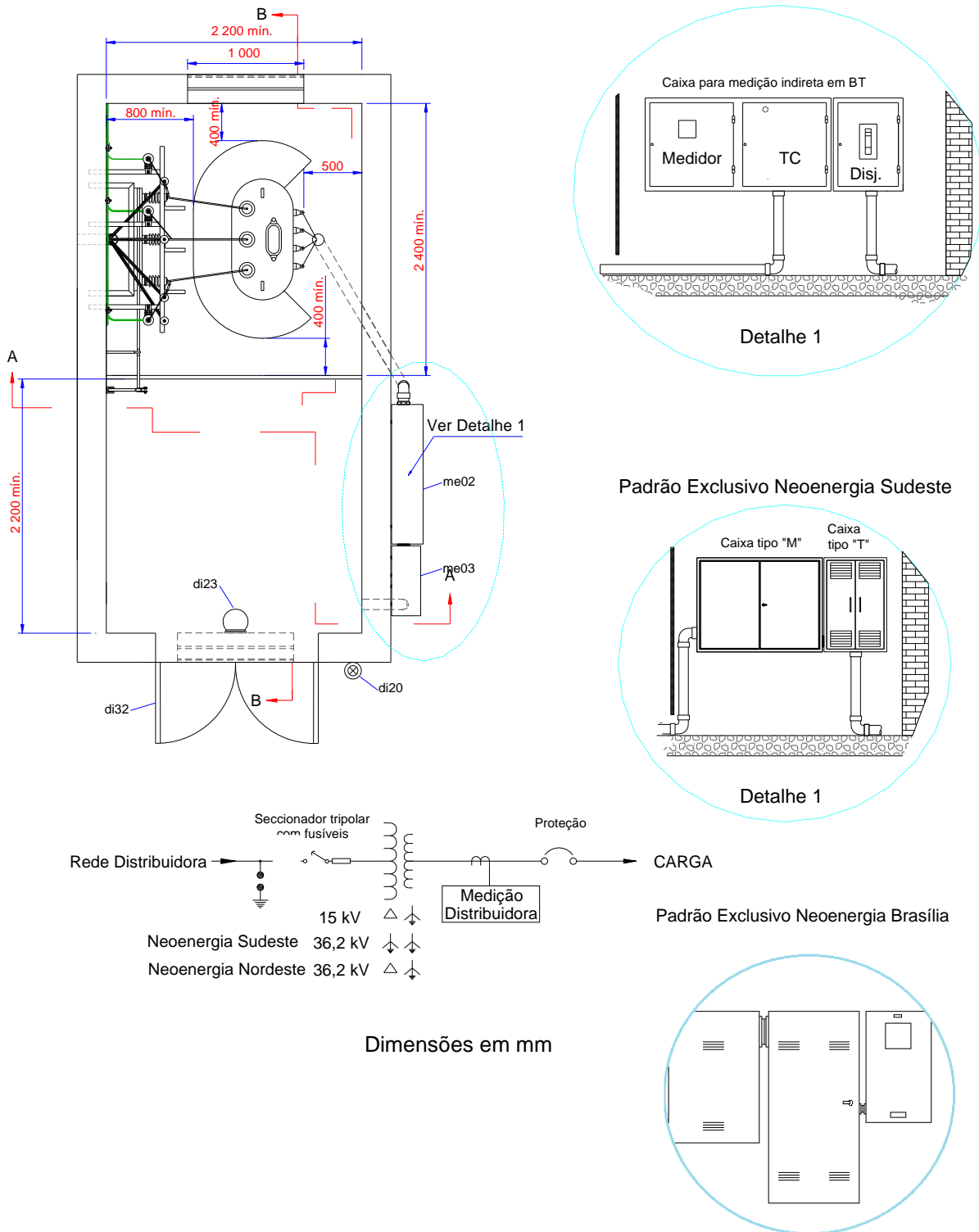
Figura 20 – Subestação Abrigada de Transformação Entrada Subterrânea – Medição BT (1/3)
