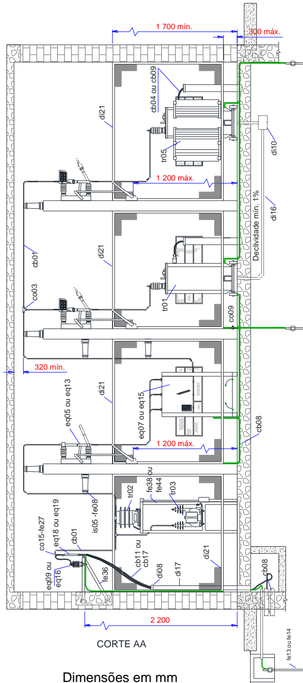
Figura 25 – Subestação Abrigada de Medição, Proteção e Transformação – Entrada Subterrânea – Medição em AT (2/4)
