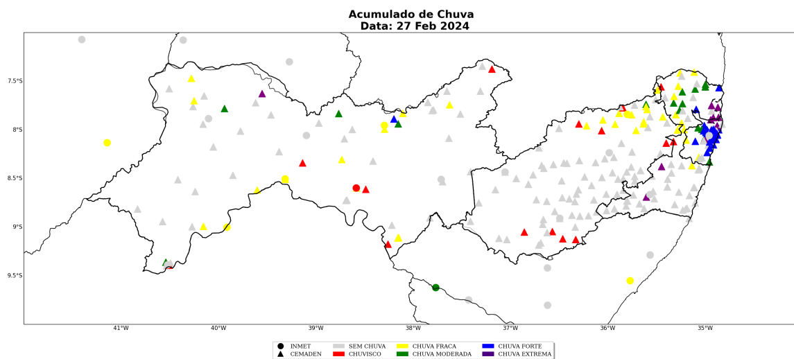
Figura 16: Acumulado diário de precipitação sobre o estado de Pernambuco para o dia 27 de fevereiro, baseado nas estações meteorológicas do INMET e CEMADEN.
