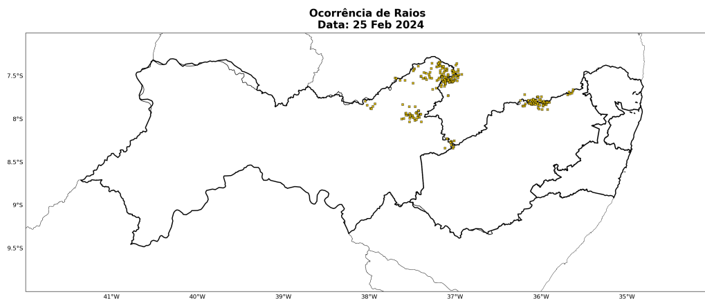
Figura 26: Ocorrência de descargas atmosféricas nuvem-solo detectadas pelo sistema Earth Networks para o dia 25 de fevereiro sobre a área de concessão da Neoenergia - Pernambuco.
