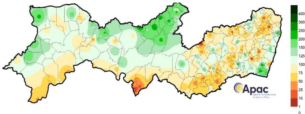
Figura 1 – representação da precipitação de março
