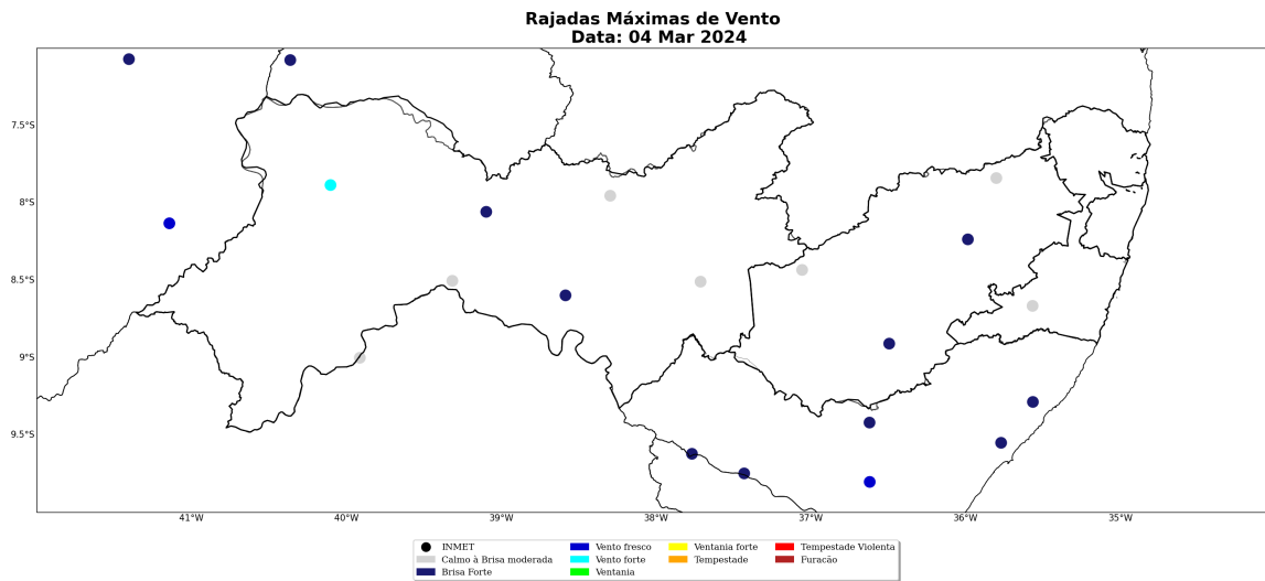
Figura 45: Rajada de vento sobre o estado de Pernambuco para o dia 04 de março, baseado nas estações meteorológicas do INMET
