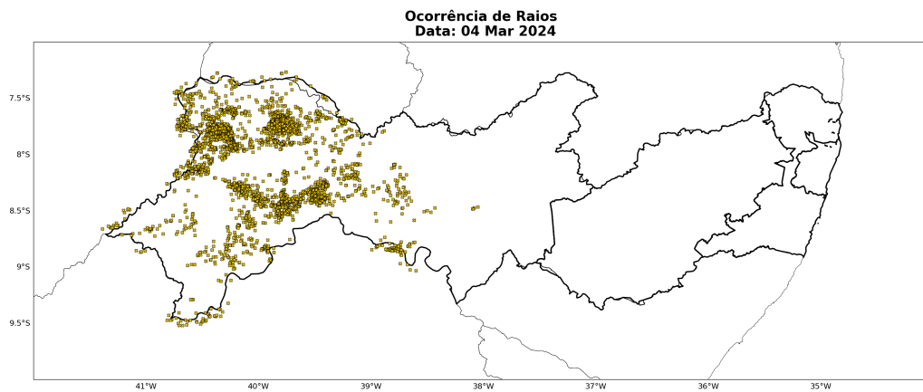
Figura 33: Ocorrência de descargas atmosféricas nuvem-solo detectadas pelo sistema Earth Networks para o dia 04 de março sobre a área de concessão da Neoenergia - Pernambuco.
