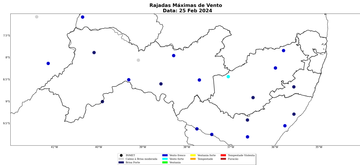
Figura 37: Rajada de vento sobre o estado de Pernambuco para o dia 25 de fevereiro, baseado nas estações meteorológicas do INMET
