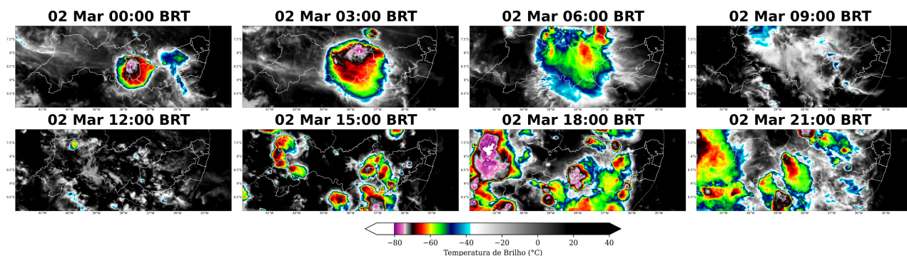
Figura 9: Imagens realçadas do satélite GOES-16 das 00 BRT até 21 BRT (a cada 3 horas) para o dia 02 de março.
