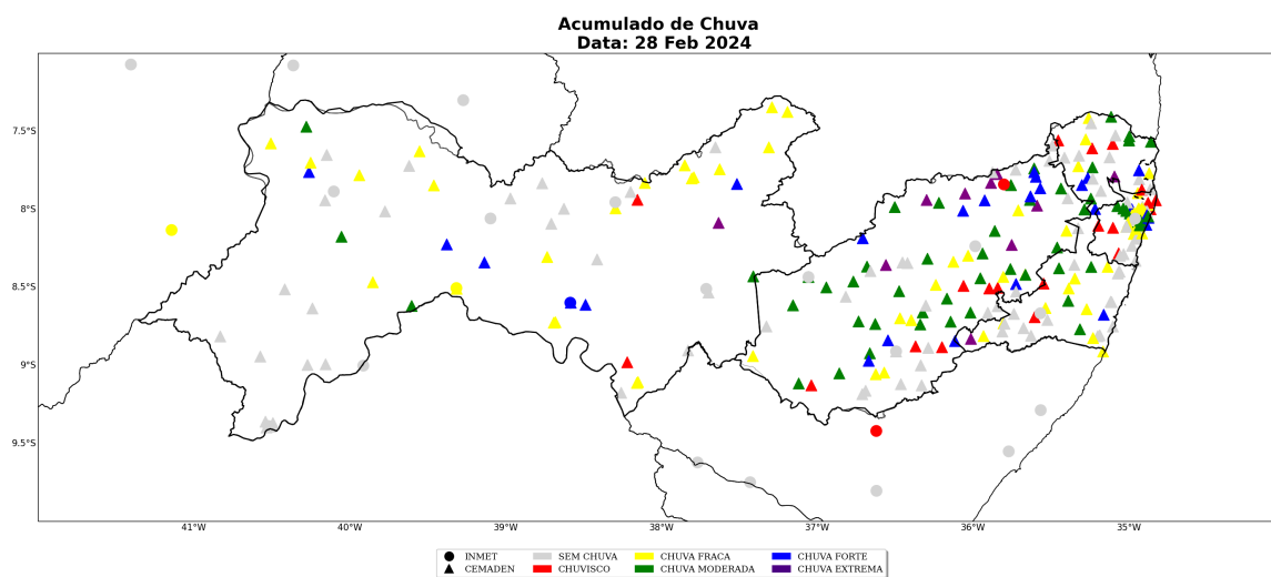
Figura 17: Acumulado diário de precipitação sobre o estado de Pernambuco para o dia 28 de fevereiro, baseado nas estações meteorológicas do INMET e CEMADEN.
