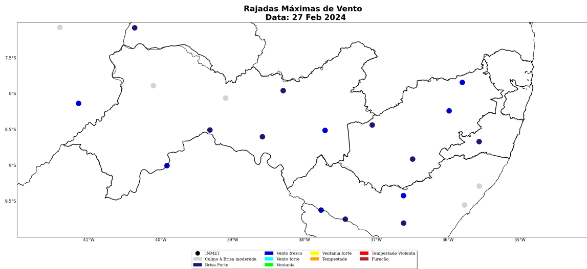
Figura 39: Rajada de vento sobre o estado de Pernambuco para o dia 27 de fevereiro, baseado nas estações meteorológicas do INMET
