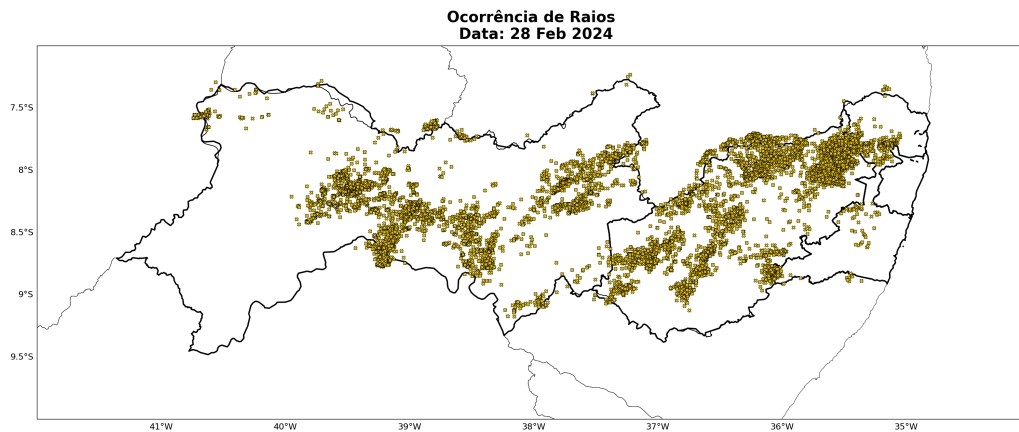
Figura 28: Ocorrência de descargas atmosféricas nuvem-solo detectadas pelo sistema Earth Networks para o dia 28 de fevereiro sobre a área de concessão da Neoenergia - Pernambuco.
