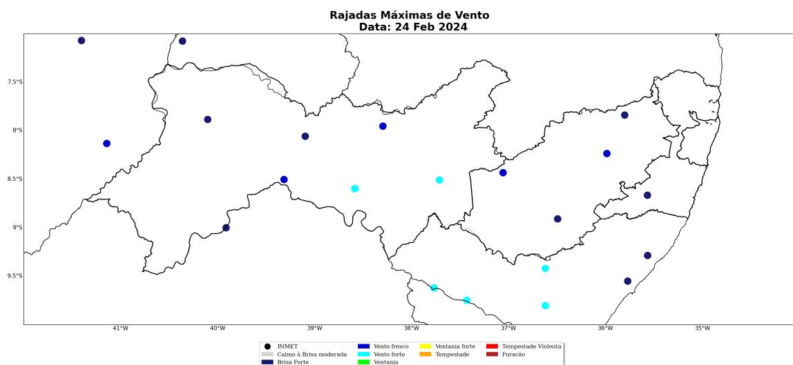
Figura 36: Rajada de vento sobre o estado de Pernambuco para o dia 24 de fevereiro, baseado nas estações meteorológicas do INMET
