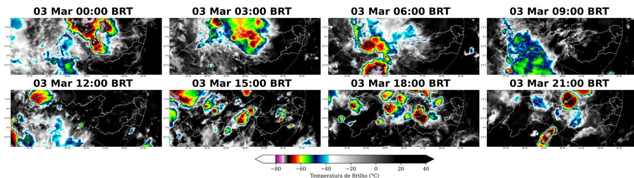
Figura 10: Imagens realçadas do satélite GOES-16 das 00 BRT até 21 BRT (a cada 3 horas) para o dia 03 de março.
