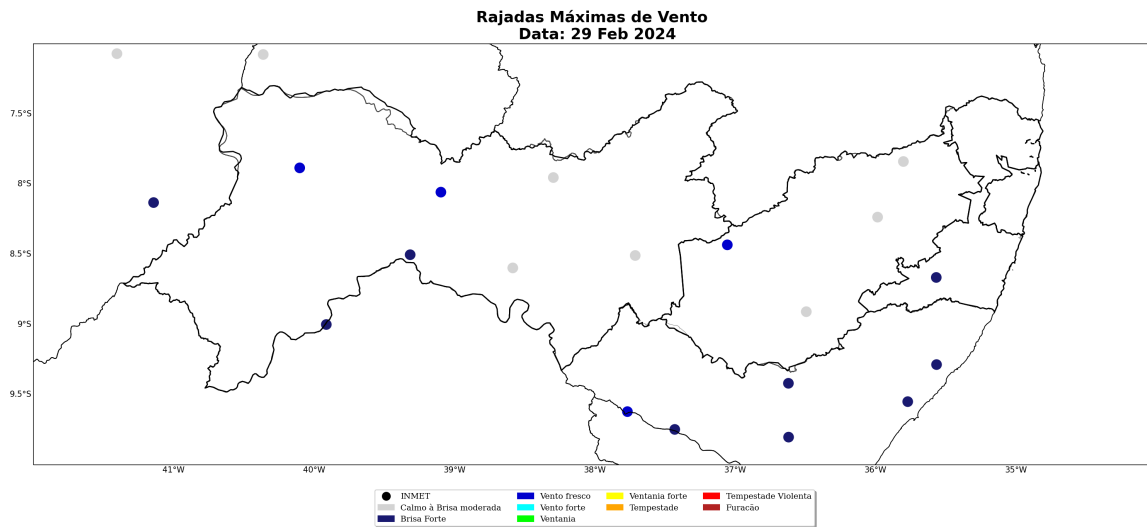
Figura 41: Rajada de vento sobre o estado de Pernambuco para o dia 29 de fevereiro, baseado nas estações meteorológicas do INMET
