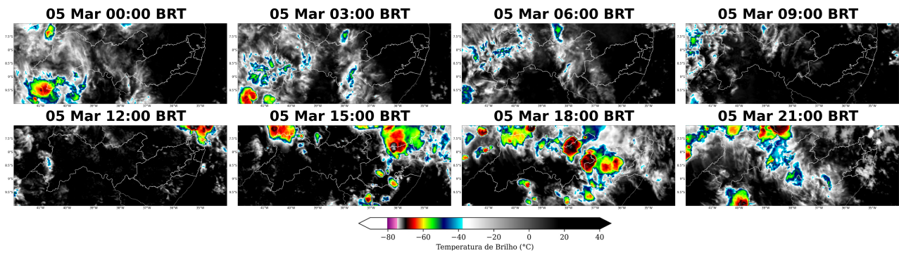
Figura 12: Imagens realçadas do satélite GOES-16 das 00 BRT até 21 BRT (a cada 3 horas) para o dia 05 de março.
