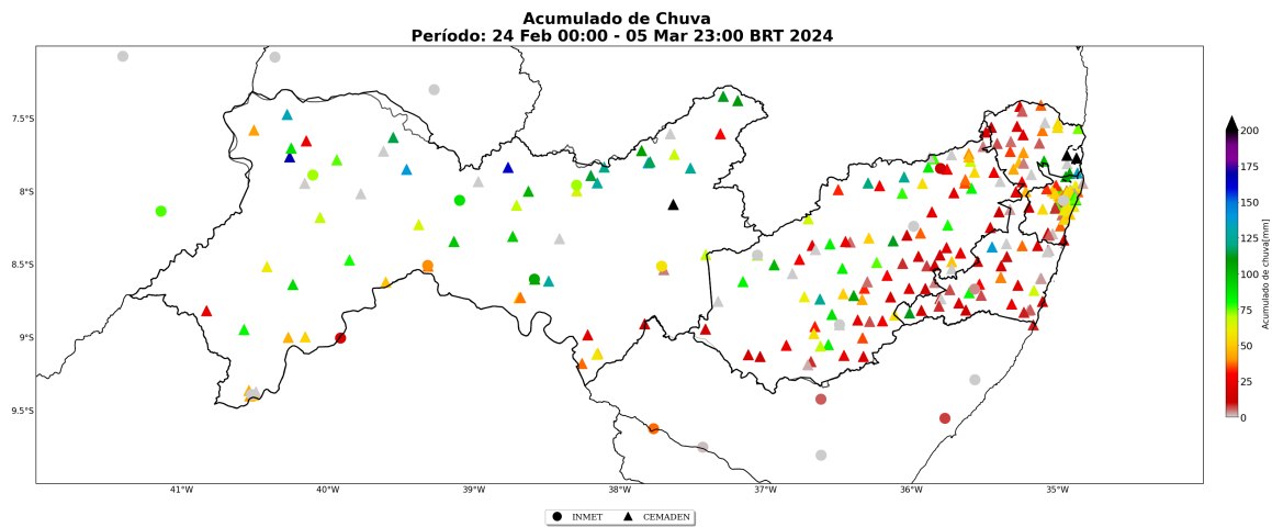
Figura 24: Acumulado de precipitação sobre o estado do Pernambuco para o período do evento (dias 24 de fevereiro a 05 de março de 2024), baseado nas estações meteorológicas do INMET e CEMADEN.
