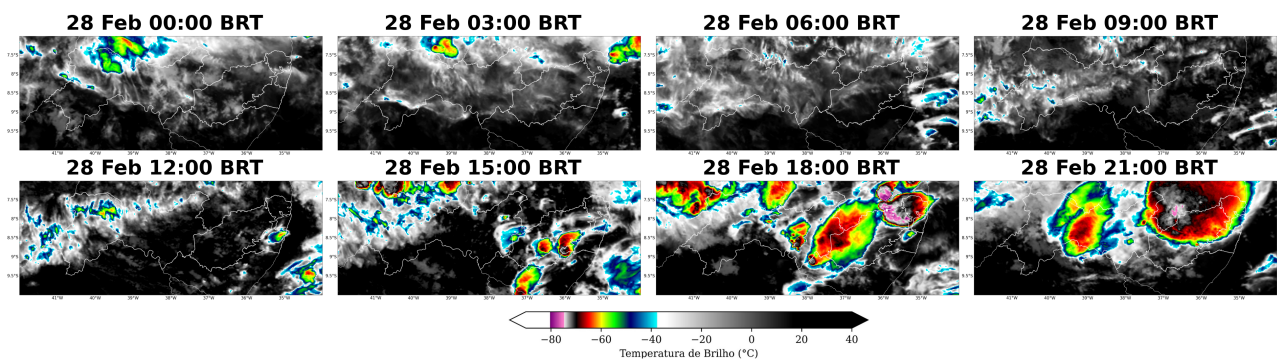
Figura 6: Imagens realçadas do satélite GOES-16 das 00 BRT até 21 BRT (a cada 3 horas) para o dia 28 de fevereiro.
