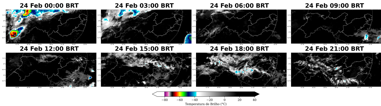
Figura 2: Imagens realçadas do satélite GOES-16 das 00 BRT até 21 BRT (a cada 3 horas) para o dia 24 de fevereiro.
