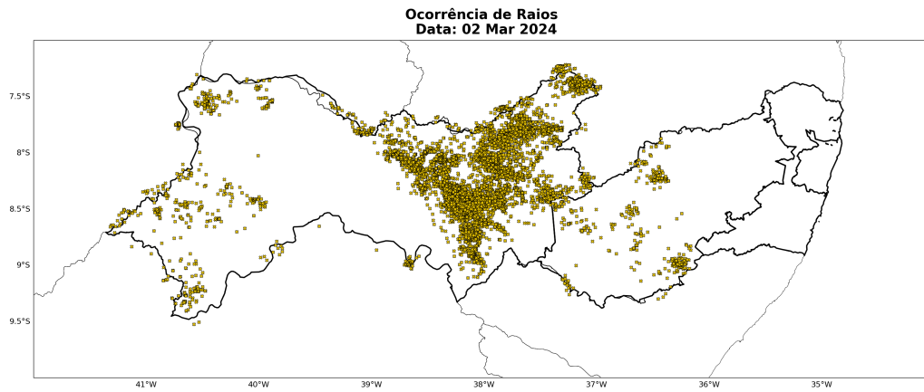
Figura 31: Ocorrência de descargas atmosféricas nuvem-solo detectadas pelo sistema Earth Networks para o dia 02 de março sobre a área de concessão da Neoenergia - Pernambuco.
