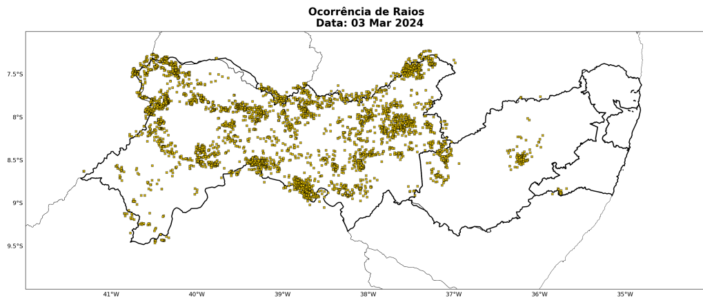
Figura 32: Ocorrência de descargas atmosféricas nuvem-solo detectadas pelo sistema Earth Networks para o dia 03 de março sobre a área de concessão da Neoenergia - Pernambuco.
