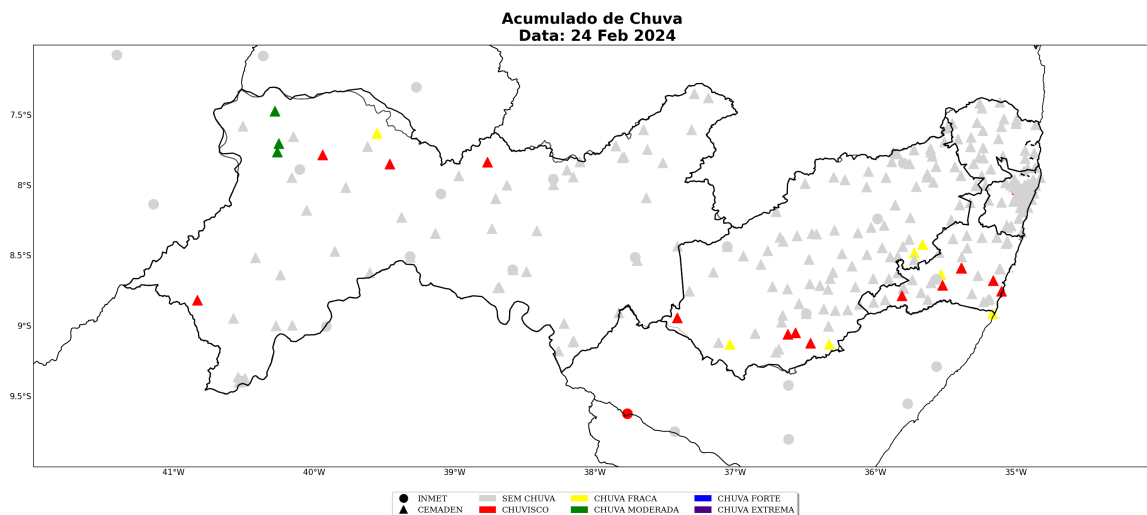
Figura 13: Acumulado diário de precipitação sobre o estado de Pernambuco para o dia 24 de fevereiro, baseado nas estações meteorológicas do INMET e CEMADEN.
