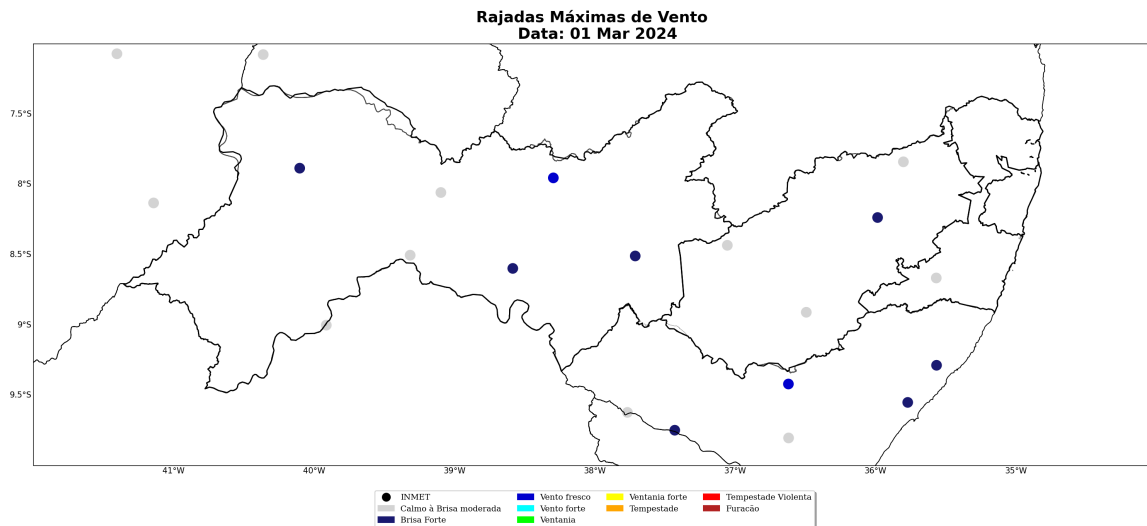
Figura 42: Rajada de vento sobre o estado de Pernambuco para o dia 01 de março, baseado nas estações meteorológicas do INMET
