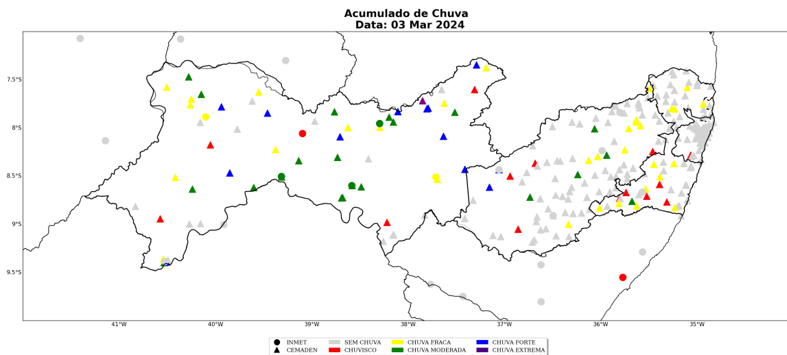
Figura 21: Acumulado diário de precipitação sobre o estado de Pernambuco para o dia 03 de março, baseado nas estações meteorológicas do INMET e CEMADEN.
