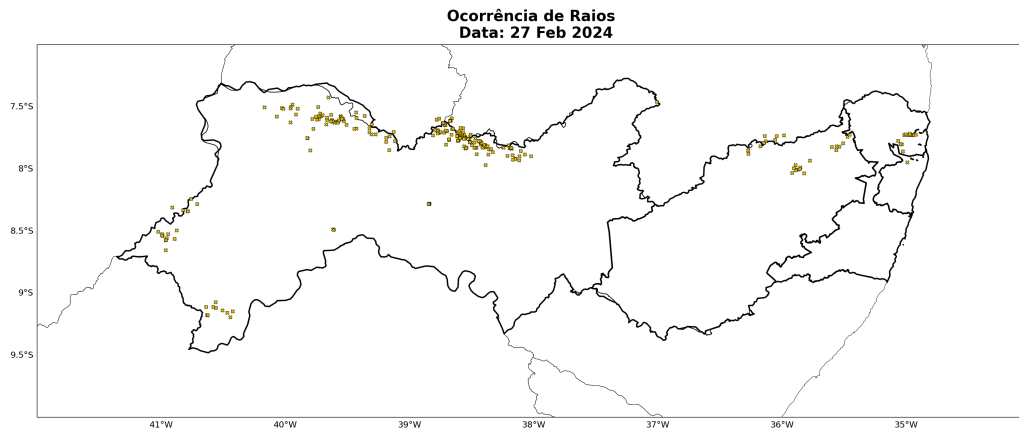
Figura 27: Ocorrência de descargas atmosféricas nuvem-solo detectadas pelo sistema Earth Networks para o dia 27 de fevereiro sobre a área de concessão da Neoenergia - Pernambuco.
