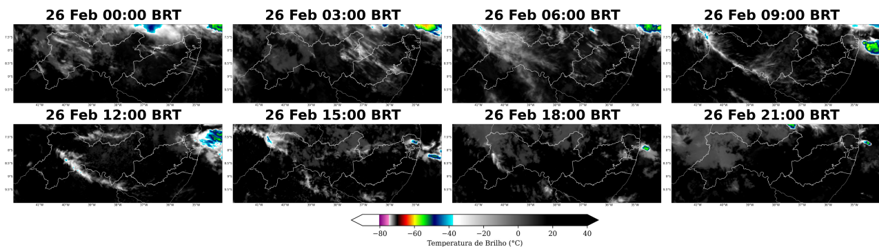
Figura 4: Imagens realçadas do satélite GOES-16 das 00 BRT até 21 BRT (a cada 3 horas) para o dia 26 de fevereiro.
