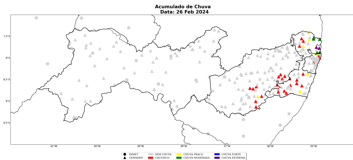
Figura 15: Acumulado diário de precipitação sobre o estado de Pernambuco para o dia 26 de fevereiro, baseado nas estações meteorológicas do INMET e CEMADEN.
