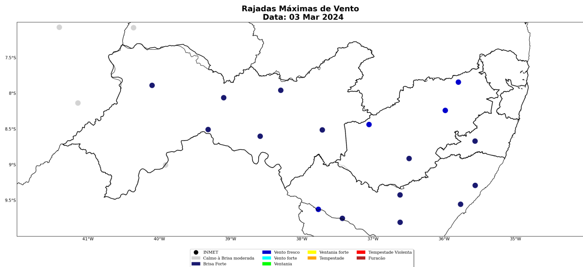
Figura 44: Rajada de vento sobre o estado de Pernambuco para o dia 03 de março, baseado nas estações meteorológicas do INMET
