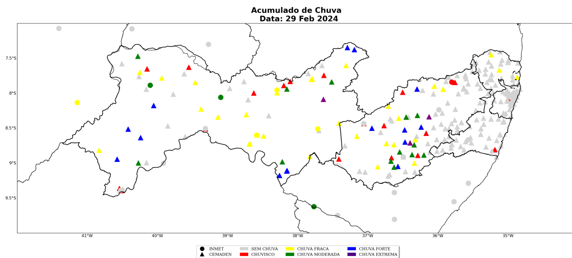
Figura 18: Acumulado diário de precipitação sobre o estado de Pernambuco para o dia 29 de fevereiro, baseado nas estações meteorológicas do INMET e CEMADEN.
