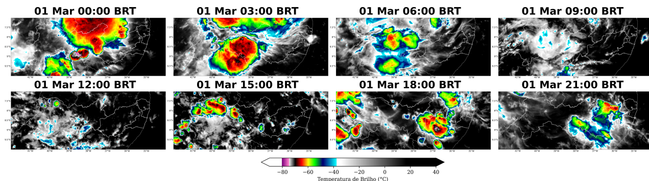
Figura 8: Imagens realçadas do satélite GOES-16 das 00 BRT até 21 BRT (a cada 3 horas) para o dia 01 de março.
