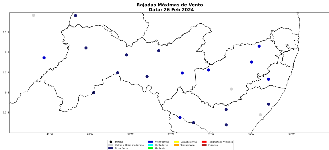
Figura 38: Rajada de vento sobre o estado de Pernambuco para o dia 26 de fevereiro, baseado nas estações meteorológicas do INMET
