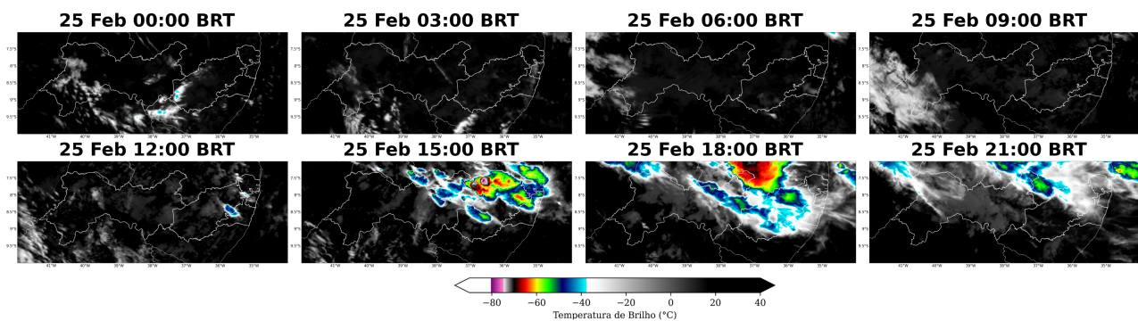
Figura 3: Imagens realçadas do satélite GOES-16 das 00 BRT até 21 BRT (a cada 3 horas) para o dia 25 de fevereiro.
