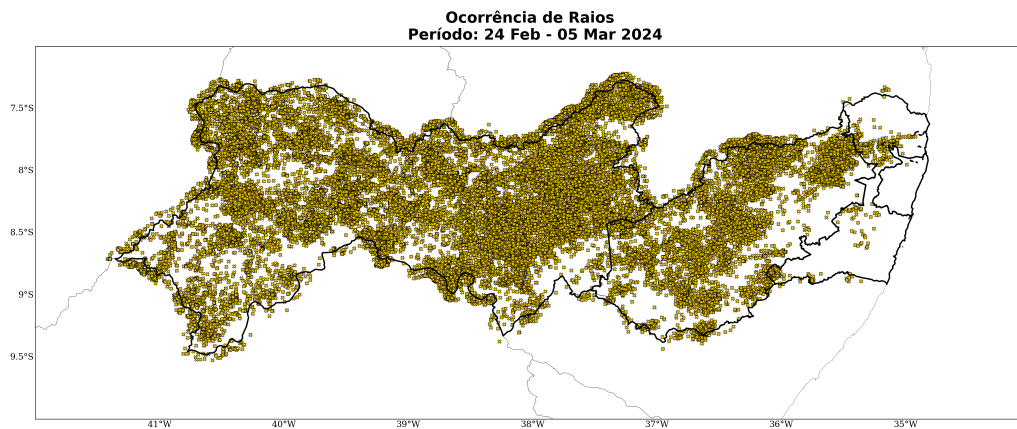
Figura 35: Ocorrência de descargas atmosféricas nuvem-solo detectadas pelo sistema Earth Networks para o período de 24 de fevereiro a 05 de março de 2024 sobre a área de concessão da Neoenergia - Pernambuco.
