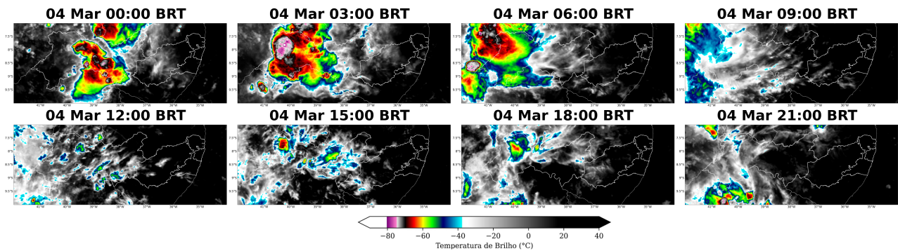
Figura 11: Imagens realçadas do satélite GOES-16 das 00 BRT até 21 BRT (a cada 3 horas) para o dia 04 de março.
