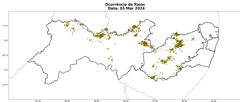
Figura 34: Ocorrência de descargas atmosféricas nuvem-solo detectadas pelo sistema Earth Networks para o dia 05 de março sobre a área de concessão da Neoenergia - Pernambuco.
