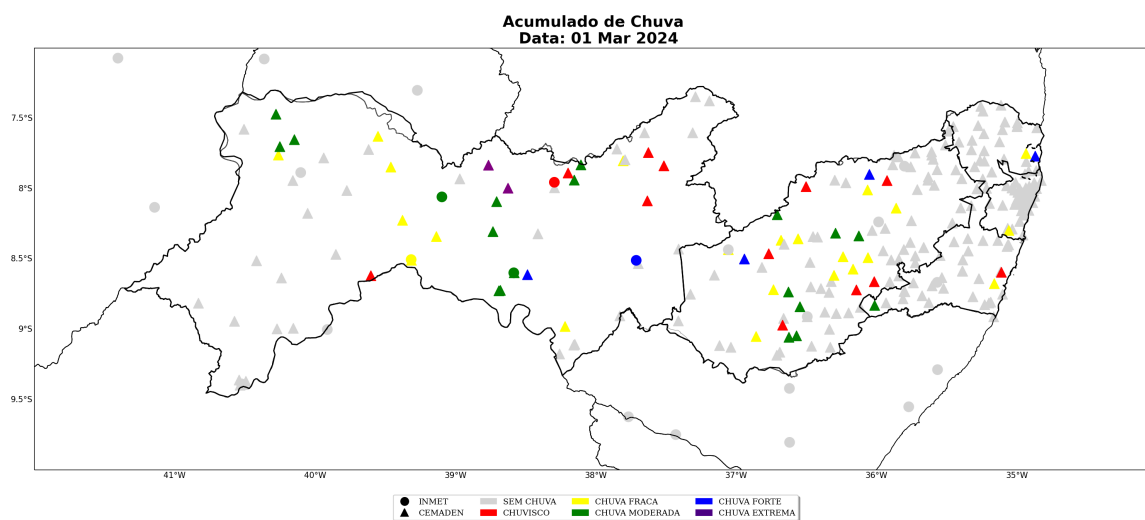
Figura 19: Acumulado diário de precipitação sobre o estado de Pernambuco para o dia 01 de março, baseado nas estações meteorológicas do INMET e CEMADEN.
