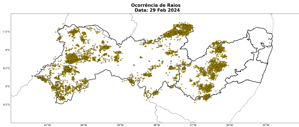
Figura 29: Ocorrência de descargas atmosféricas nuvem-solo detectadas pelo sistema Earth Networks para o dia 29 de fevereiro sobre a área de concessão da Neoenergia - Pernambuco.
