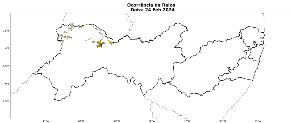
Figura 25: Ocorrência de descargas atmosféricas nuvem-solo detectadas pelo sistema Earth Networks para o dia 24 de fevereiro sobre a área de concessão da Neoenergia - Pernambuco.
