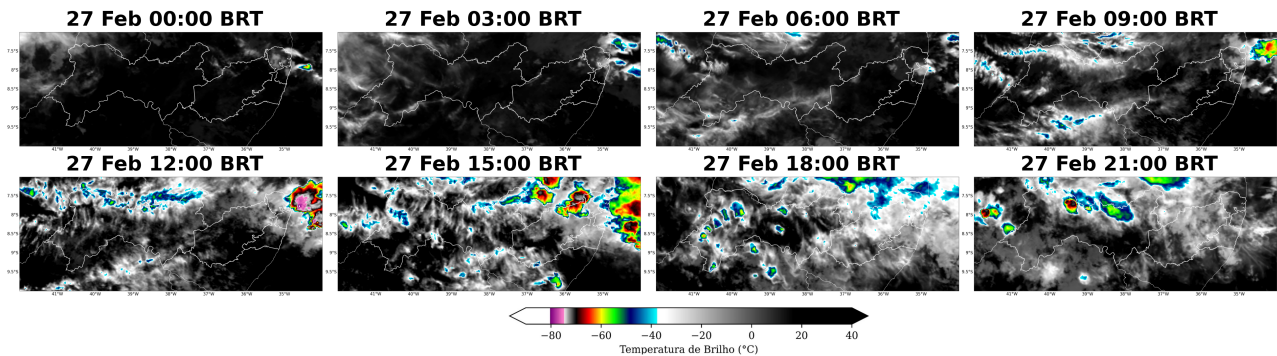
Figura 5: Imagens realçadas do satélite GOES-16 das 00 BRT até 21 BRT (a cada 3 horas) para o dia 27 de fevereiro.
