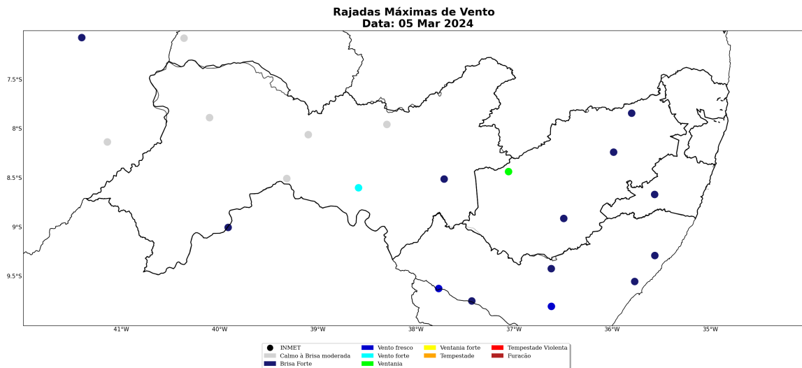
Figura 46: Rajada de vento sobre o estado de Pernambuco para o dia 05 de março, baseado nas estações meteorológicas do INMET
