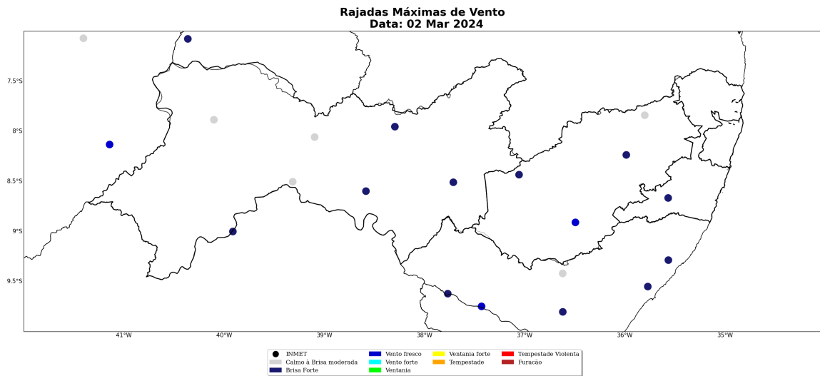
Figura 43: Rajada de vento sobre o estado de Pernambuco para o dia 02 de março, baseado nas estações meteorológicas do INMET
