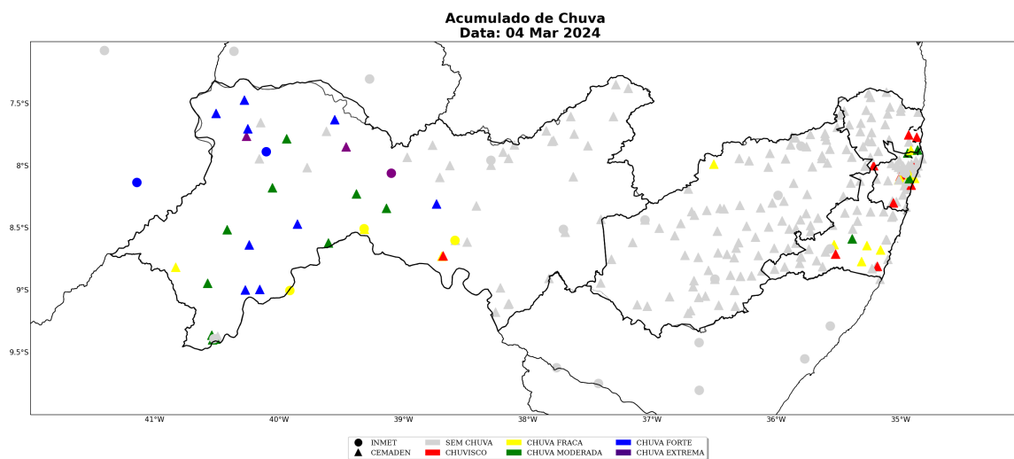
Figura 22: Acumulado diário de precipitação sobre o estado de Pernambuco para o dia 04 de março, baseado nas estações meteorológicas do INMET e CEMADEN.
