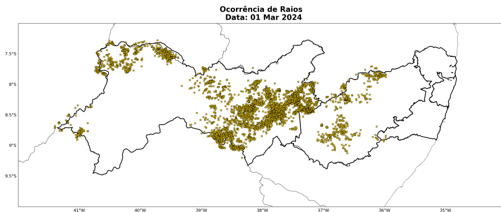
Figura 30: Ocorrência de descargas atmosféricas nuvem-solo detectadas pelo sistema Earth Networks para o dia 01 de março sobre a área de concessão da Neoenergia - Pernambuco.
