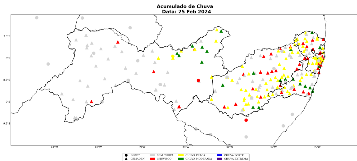
Figura 14: Acumulado diário de precipitação sobre o estado de Pernambuco para o dia 25 de fevereiro, baseado nas estações meteorológicas do INMET e CEMADEN.
