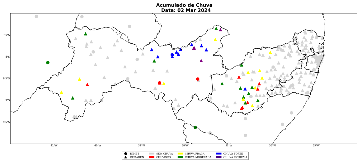
Figura 20: Acumulado diário de precipitação sobre o estado de Pernambuco para o dia 02 de março, baseado nas estações meteorológicas do INMET e CEMADEN.
