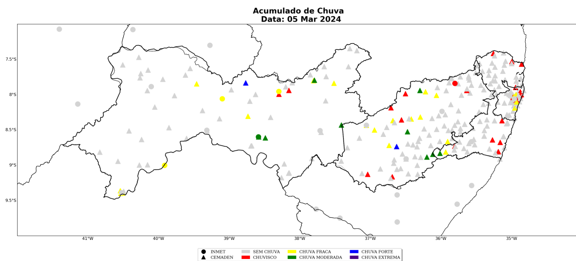
Figura 23: Acumulado diário de precipitação sobre o estado de Pernambuco para o dia 05 de março, baseado nas estações meteorológicas do INMET e CEMADEN.
