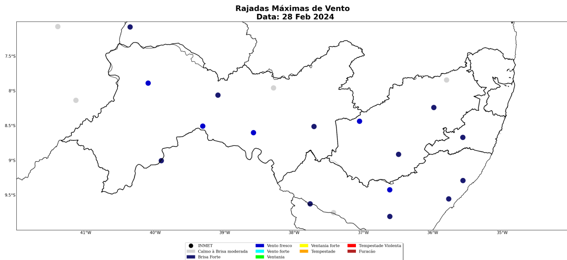
Figura 40: Rajada de vento sobre o estado de Pernambuco para o dia 28 de fevereiro, baseado nas estações meteorológicas do INMET
