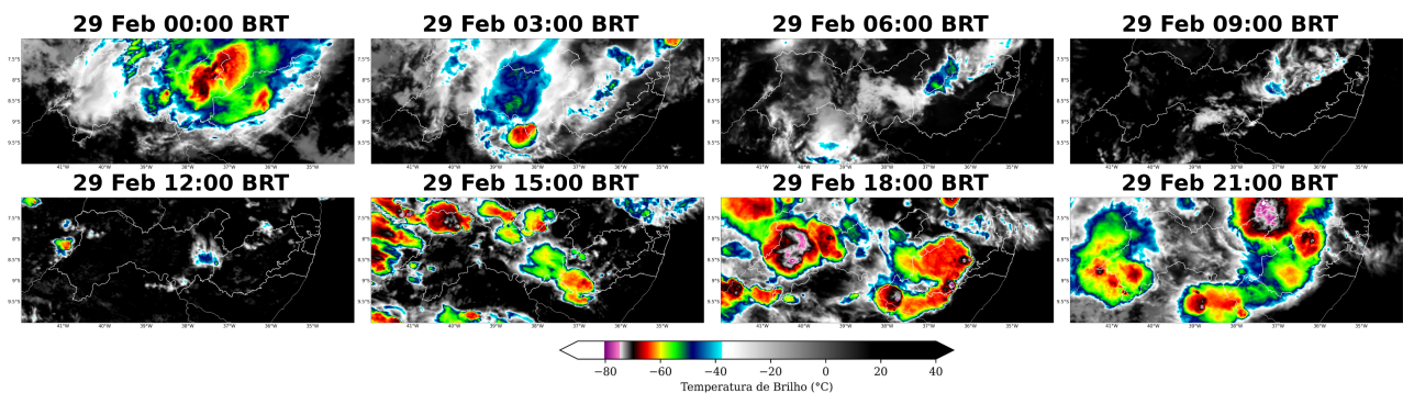
Figura 7: Imagens realçadas do satélite GOES-16 das 00 BRT até 21 BRT (a cada 3 horas) para o dia 29 de fevereiro.
