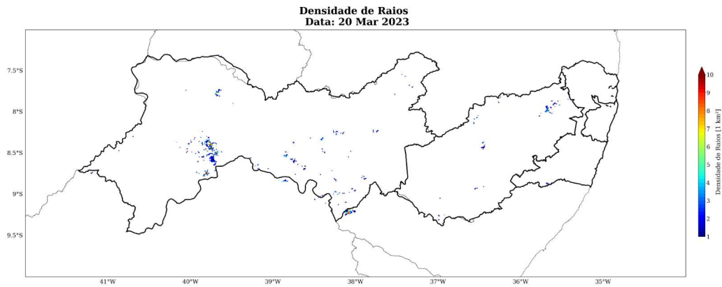
Figura 32: Densidade de descargas atmosféricas nuvem-solo detectadas pelo sistema Earth Networks para o dia 20 de março sobre a área de concessão da Neoenergia - Pernambuco.
