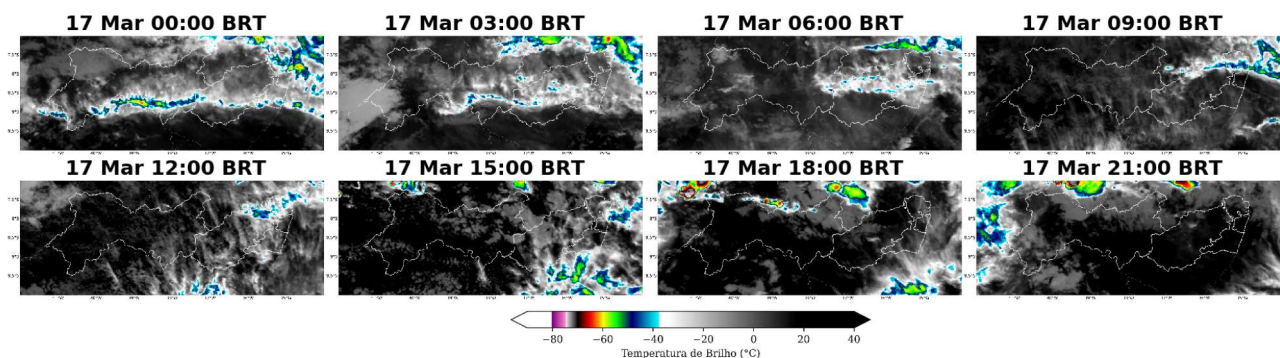
Figura 6: Imagens realçadas do satélite GOES-16 das 00 BRT até 21 BRT (a cada 3 horas) para o dia 17 de março.
