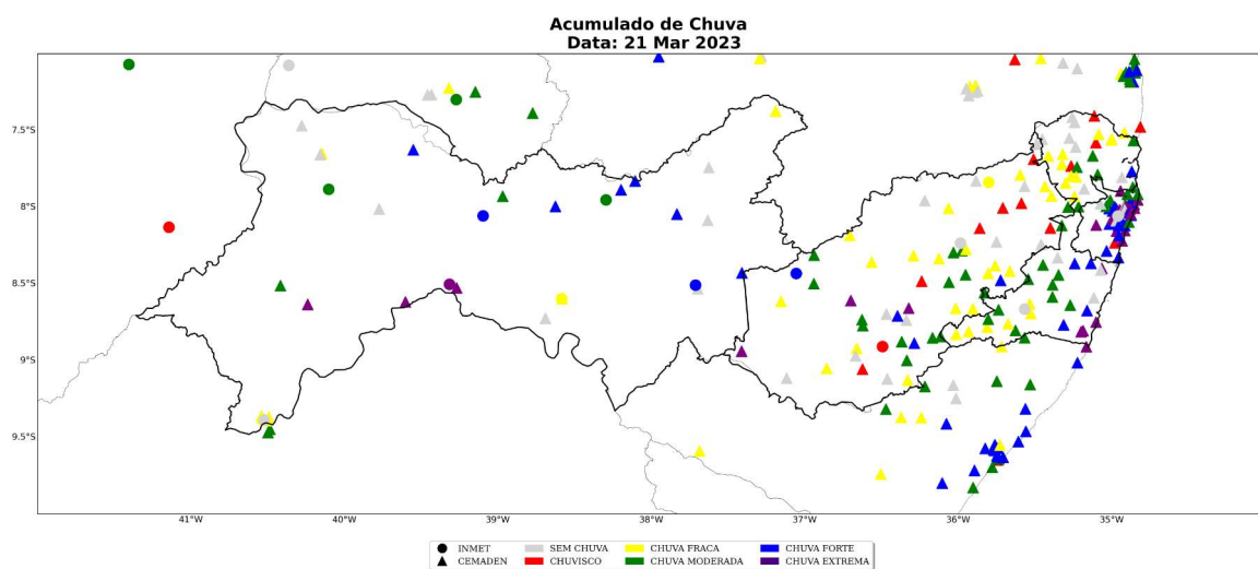
Figura 22: Acumulado diário de precipitação sobre o estado de Pernambuco para o dia 21 de março, baseado nas estações meteorológicas do INMET e CEMADEN
