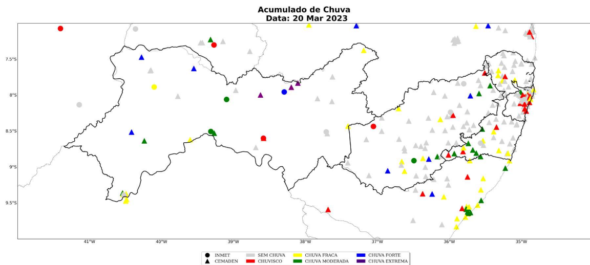
Figura 21: Acumulado diário de precipitação sobre o estado de Pernambuco para o dia 20 de março, baseado nas estações meteorológicas do INMET e CEMADEN
