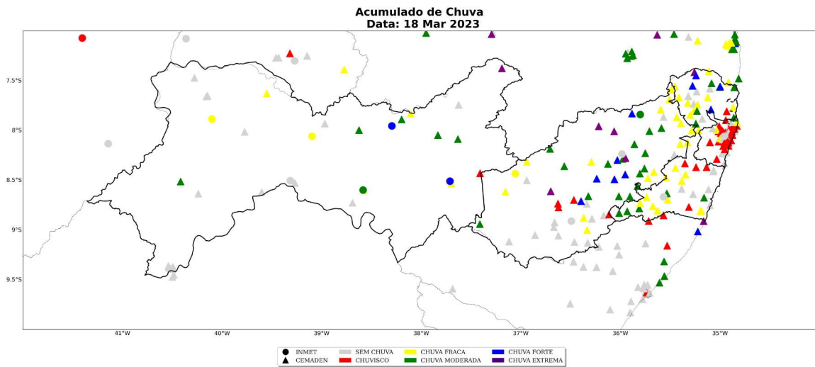
Figura 19: Acumulado diário de precipitação sobre o estado de Pernambuco para o dia 18 de março, baseado nas estações meteorológicas do INMET e CEMADEN
