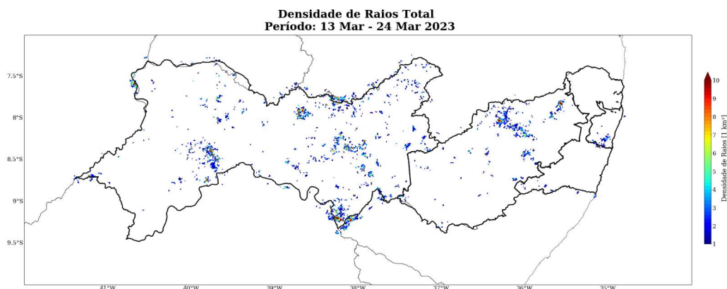
Figura 36: Densidade de descargas atmosféricas nuvem-solo detectadas pelo sistema Earth Networks para o período de 13 a 24 de março de 2023 sobre a área de concessão da Neoenergia - Pernambuco.
