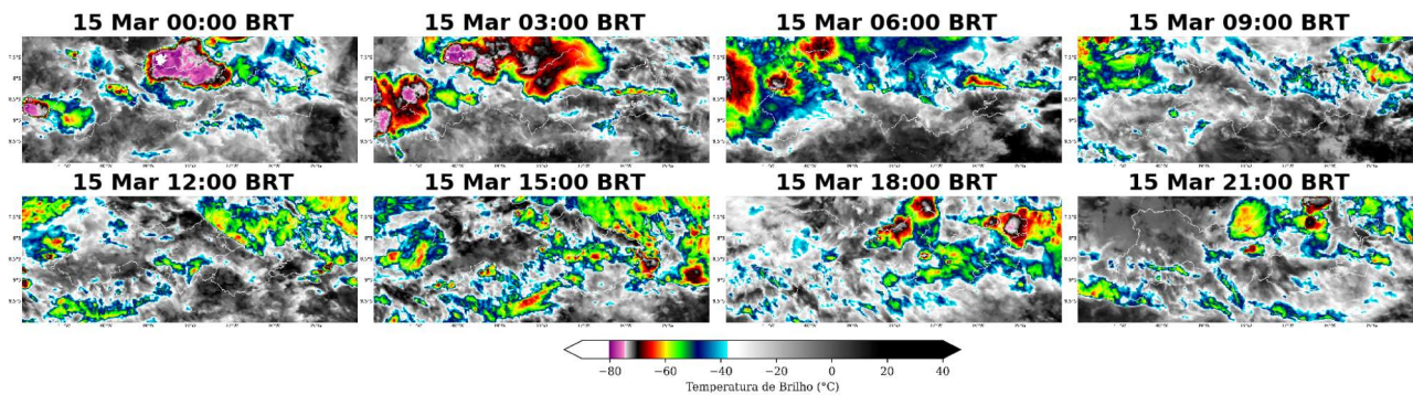
Figura 4: Imagens realçadas do satélite GOES-16 das 00 BRT até 21 BRT (a cada 3 horas) para o dia 15 de março.
