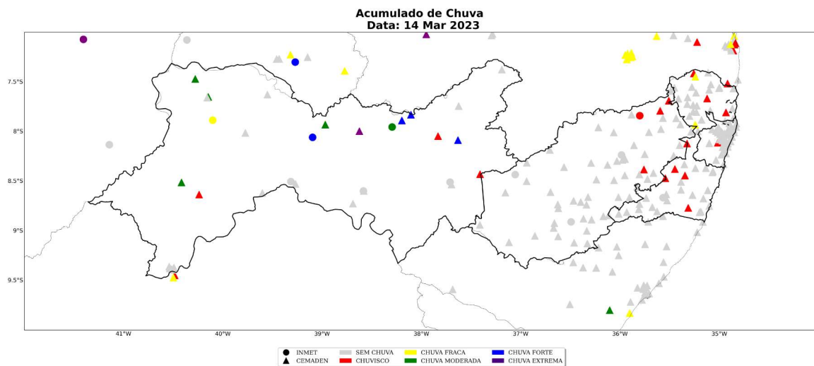
Figura 15: Acumulado diário de precipitação sobre o estado de Pernambuco para o dia 14 de março, baseado nas estações meteorológicas do INMET e CEMADEN
