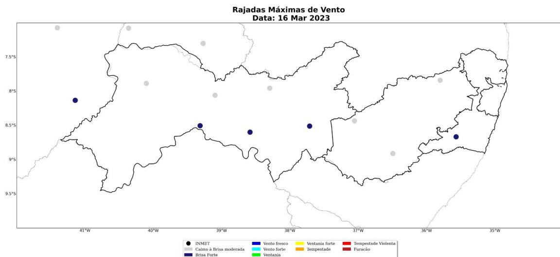
Figura 40: Rajada de vento sobre o estado de Pernambuco para o dia 16 de março, baseado nas estações meteorológicas do INMET
