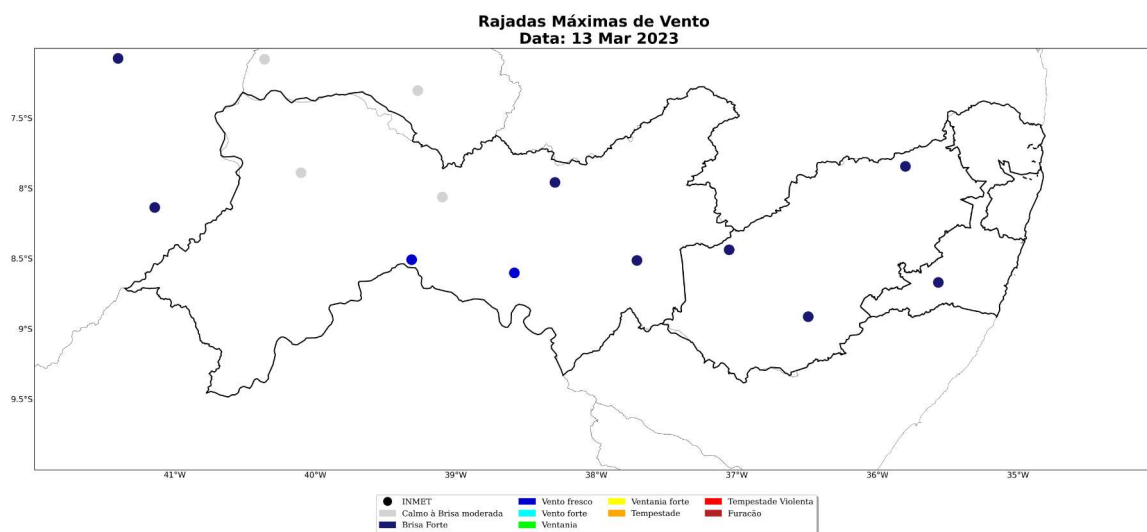
Figura 37: Rajada de vento sobre o estado de Pernambuco para o dia 13 de março, baseado nas estações meteorológicas do INMET
