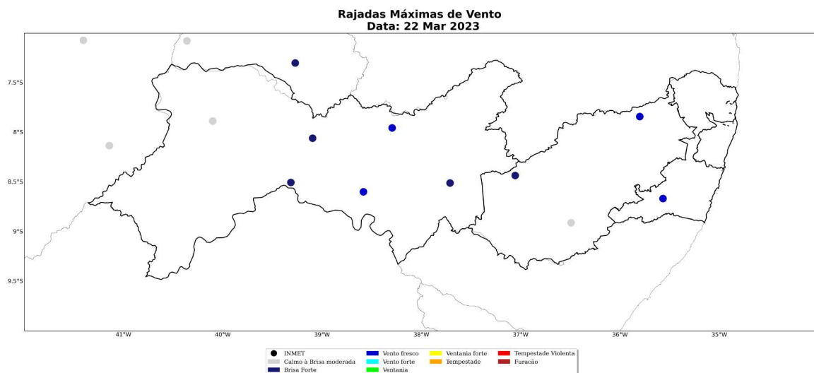
Figura 46: Rajada de vento sobre o estado de Pernambuco para o dia 22 de março, baseado nas estações meteorológicas do INMET
