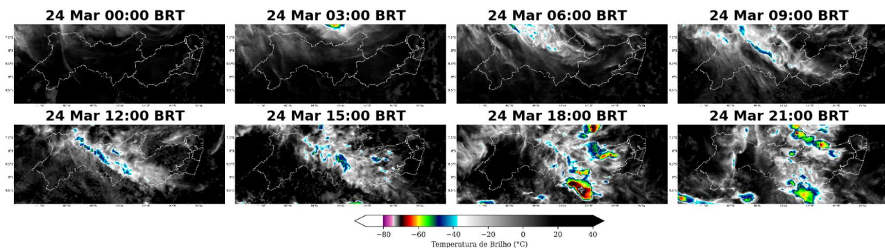
Figura 13: Imagens realçadas do satélite GOES-16 das 00 BRT até 21 BRT (a cada 3 horas) para o dia 24 de março.
