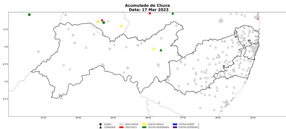
Figura 18: Acumulado diário de precipitação sobre o estado de Pernambuco para o dia 17 de março, baseado nas estações meteorológicas do INMET e CEMADEN
