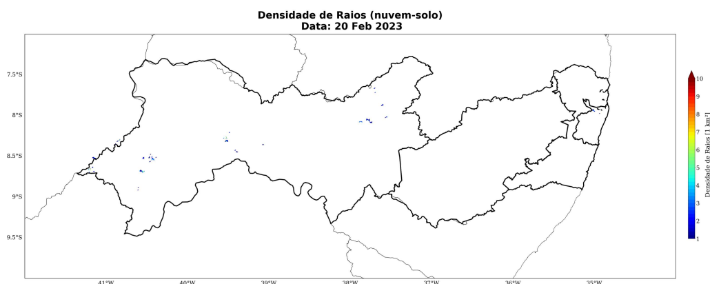
Figura 23: Densidade de descargas atmosféricas nuvem-solo detectadas pelo sistema Earth Networks para o dia 20 de fevereiro sobre a área de concessão da Neoenergia - Pernambuco.
