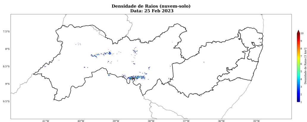
Figura 27: Densidade de descargas atmosféricas nuvem-solo detectadas pelo sistema Earth Networks para o dia 25 de fevereiro sobre a área de concessão da Neoenergia - Pernambuco.
