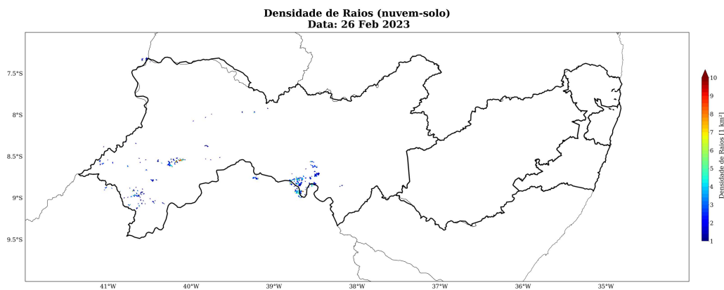
Figura 28: Densidade de descargas atmosféricas nuvem-solo detectadas pelo sistema Earth Networks para o dia 26 de fevereiro sobre a área de concessão da Neoenergia - Pernambuco.
