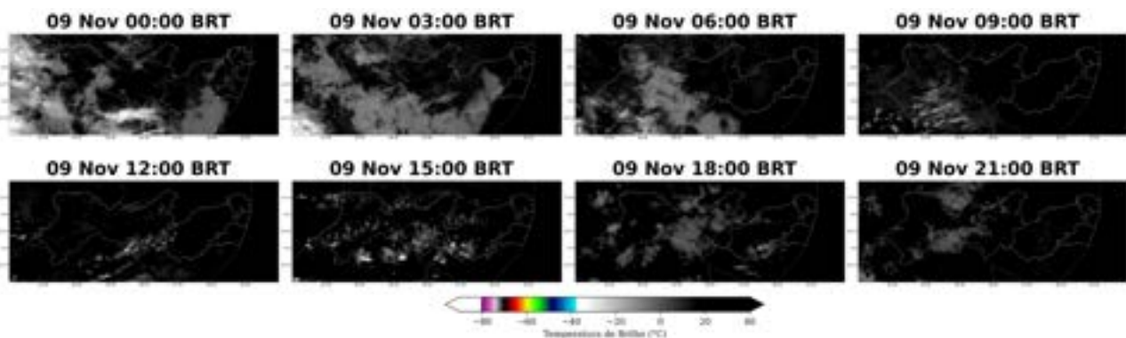
Figura 8: Imagens realçadas do satélite GOES-16 das 00 BRT até 21 BRT (a cada 3 horas) para o dia 09 de novembro.
