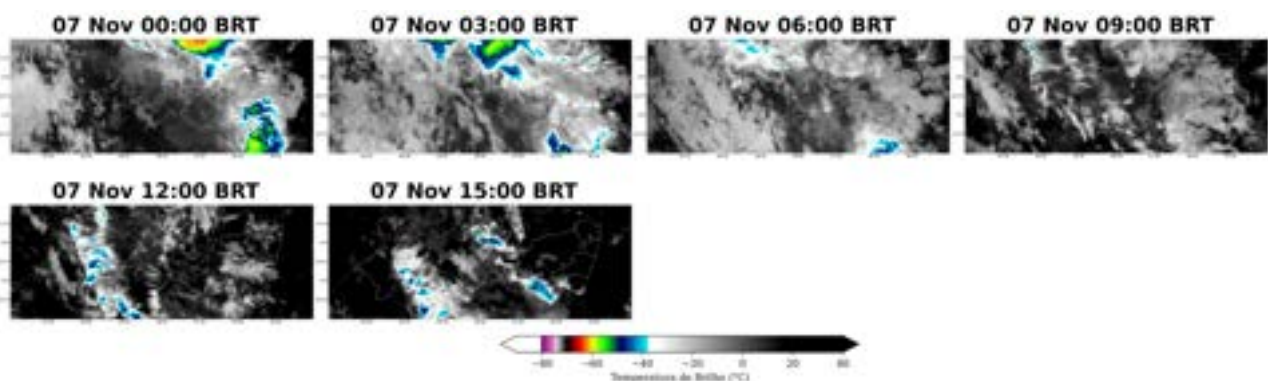
Figura 6: Imagens realçadas do satélite GOES-16 das 00 BRT até 21 BRT (a cada 3 horas) para o dia 07 de novembro.
