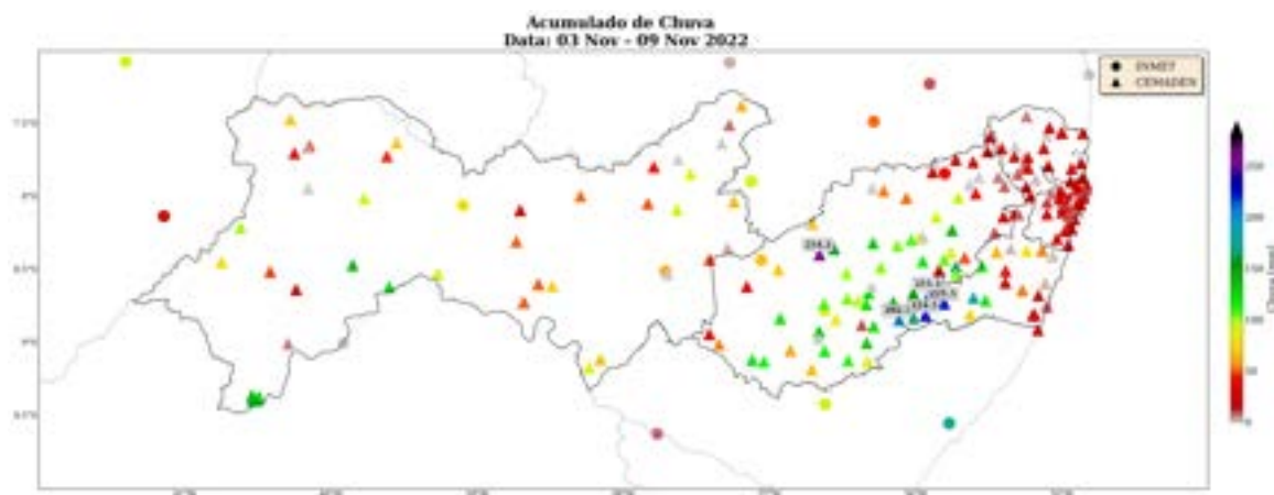
Figura 16: Acumulado de precipitação sobre o estado de Pernambuco para o período do evento (03 a 09 de novembro de 2022), baseado nas estações meteorológicas do INMET e CEMADEN.
