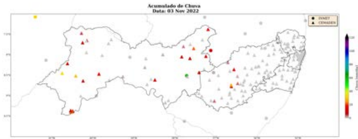
Figura 9: Acumulado diário de precipitação sobre o estado de Pernambuco para o dia 03 de novembro, baseado nas estações meteorológicas do INMET e CEMADEN
