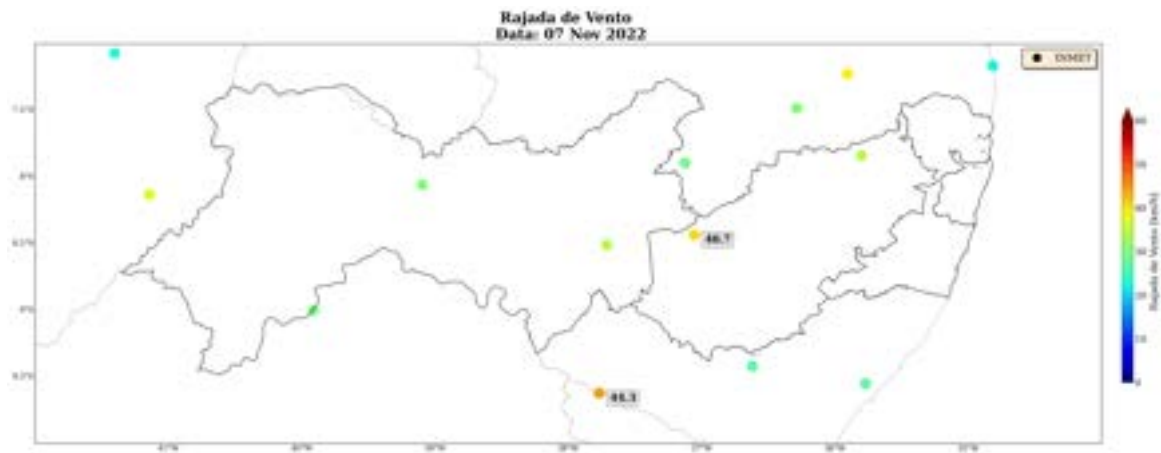
Figura 26: Rajada de vento sobre o estado de Pernambuco para o dia 07 de novembro, baseado nas estações meteorológicas do INMET
