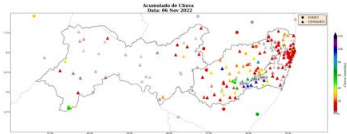
Figura 12: Acumulado diário de precipitação sobre o estado de Pernambuco para o dia 06 de novembro, baseado nas estações meteorológicas do INMET e CEMADEN
