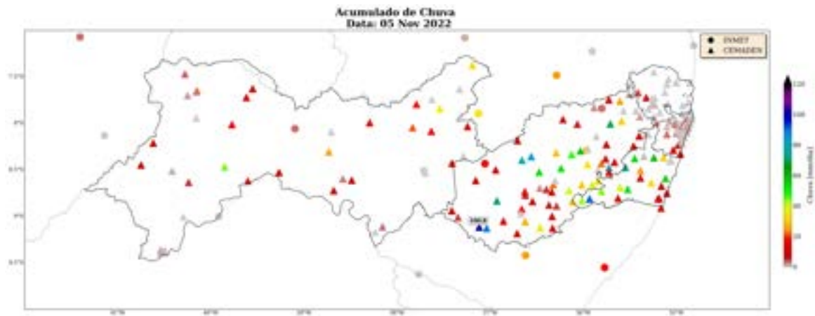
Figura 11: Acumulado diário de precipitação sobre o estado de Pernambuco para o dia 05 de novembro, baseado nas estações meteorológicas do INMET e CEMADEN
