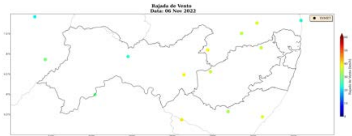
Figura 25: Rajada de vento sobre o estado de Pernambuco para o dia 06 de novembro, baseado nas estações meteorológicas do INMET
