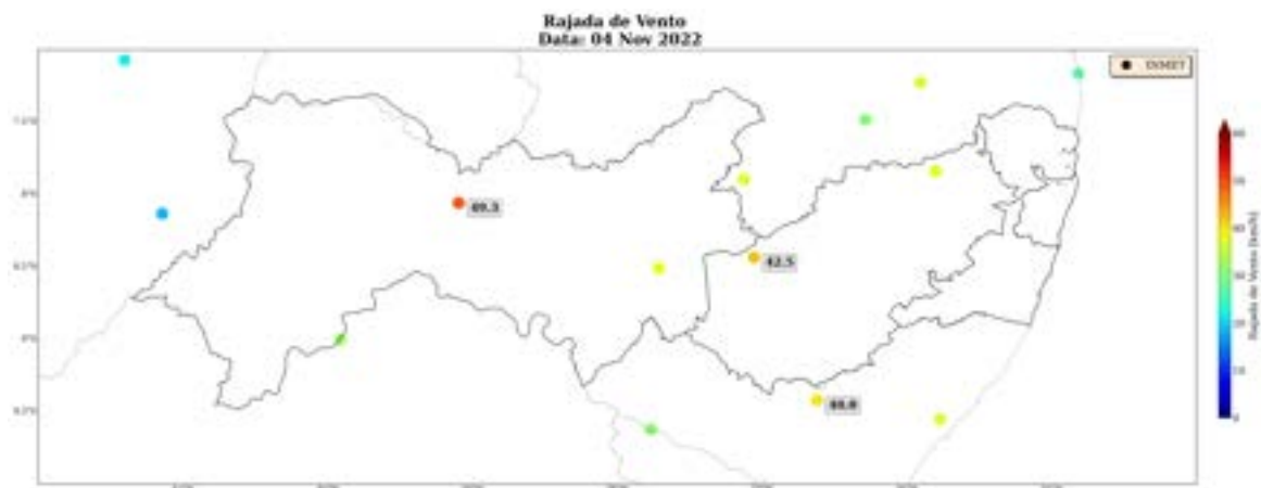
Figura 23: Rajada de vento sobre o estado de Pernambuco para o dia 04 de novembro, baseado nas estações meteorológicas do INMET
