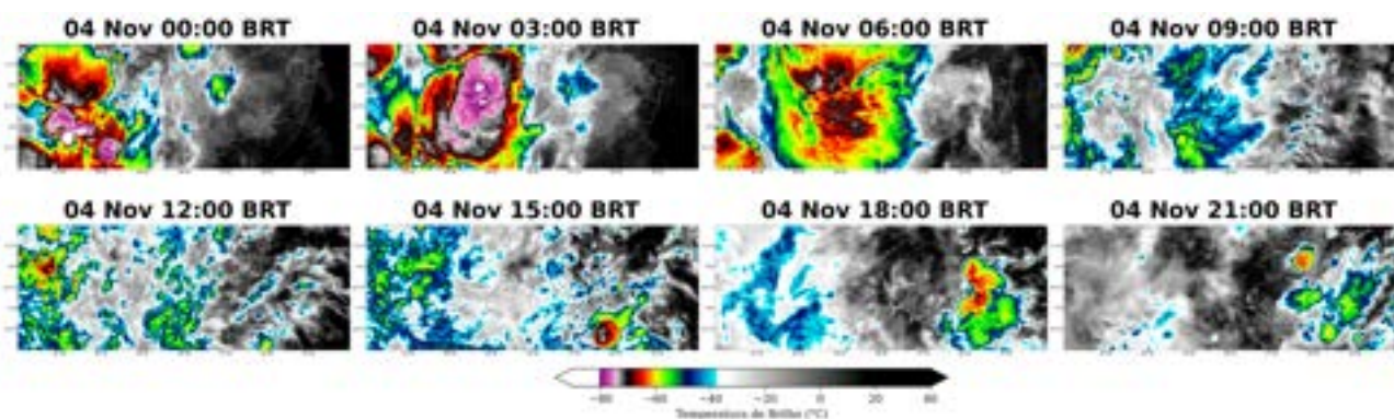
Figura 3: Imagens realçadas do satélite GOES-16 das 00 BRT até 21 BRT (a cada 3 horas) para o dia 04 de novembro.
