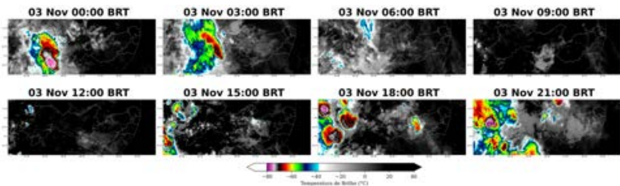
Figura 2: Imagens realçadas do satélite GOES-16 das 00 BRT até 21 BRT (a cada 3 horas) para o dia 03 de novembro.
