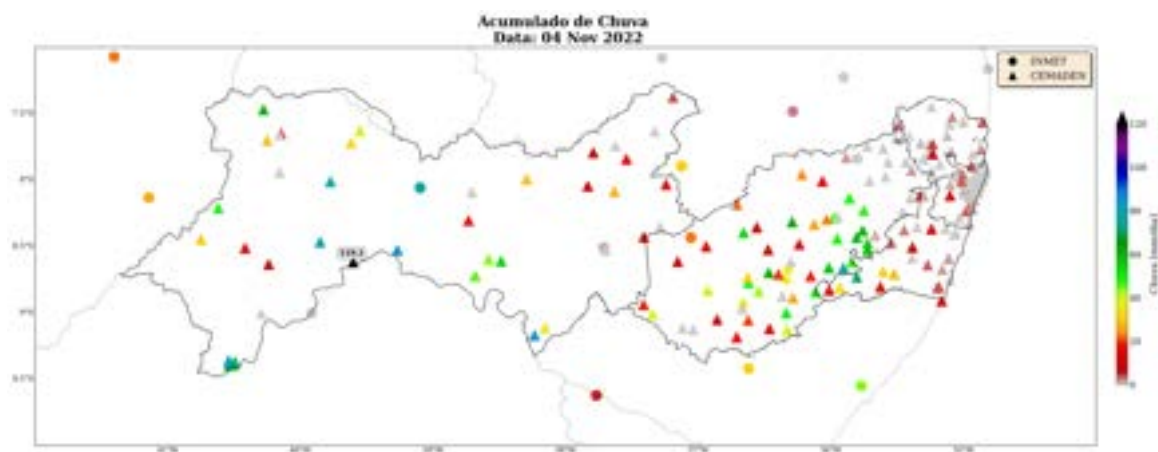
Figura 10: Acumulado diário de precipitação sobre o estado de Pernambuco para o dia 04 de novembro, baseado nas estações meteorológicas do INMET e CEMADEN
