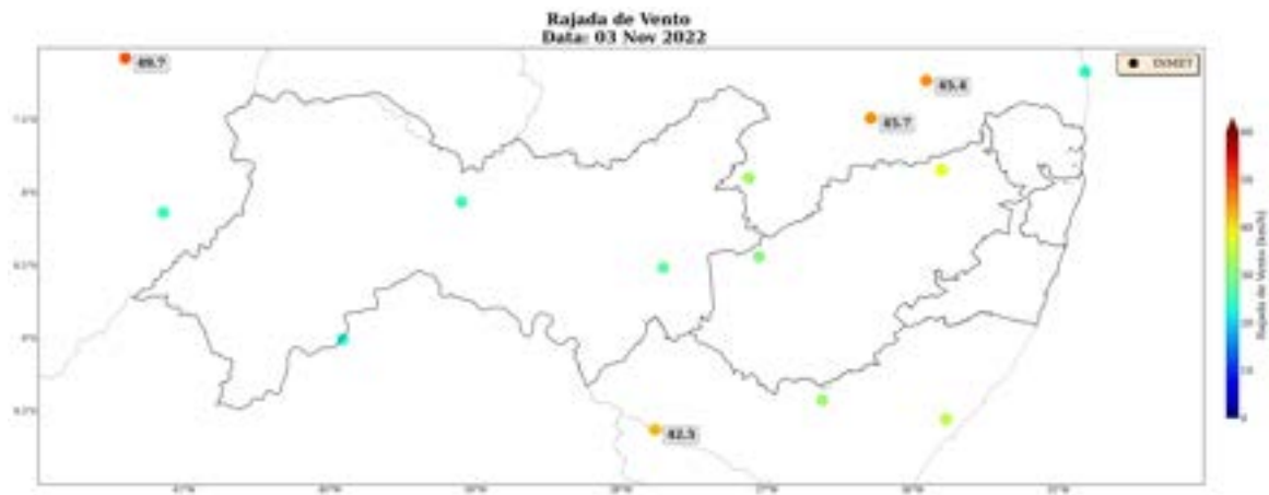
Figura 22: Rajada de vento sobre o estado de Pernambuco para o dia 03 de novembro, baseado nas estações meteorológicas do INMET
