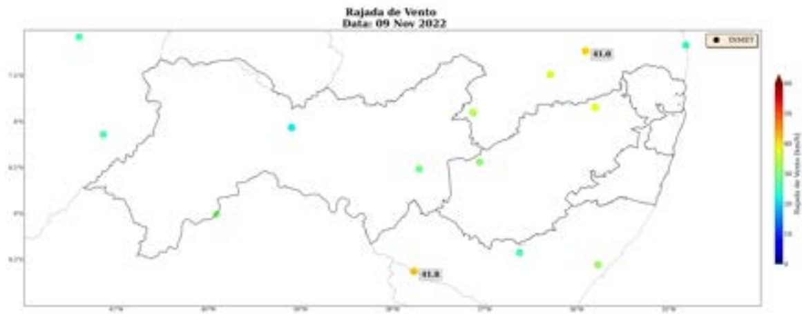
Figura 28: Rajada de vento sobre o estado de Pernambuco para o dia 09 de novembro, baseado nas estações meteorológicas do INMET
