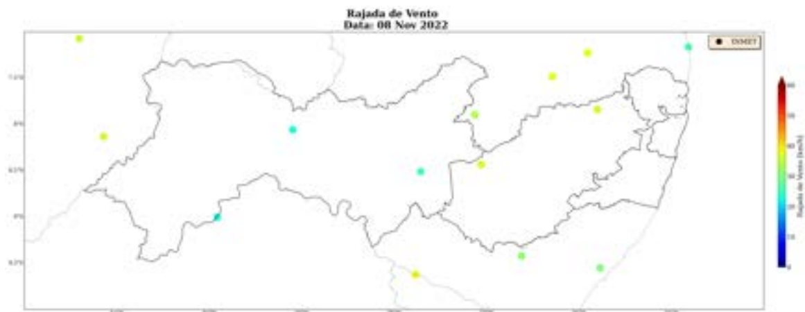
Figura 27: Rajada de vento sobre o estado de Pernambuco para o dia 08 de novembro, baseado nas estações meteorológicas do INMET
