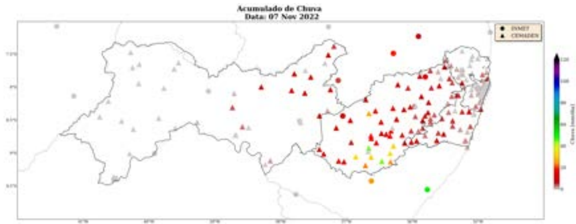
Figura 13: Acumulado diário de precipitação sobre o estado de Pernambuco para o dia 07 de novembro, baseado nas estações meteorológicas do INMET e CEMADEN
