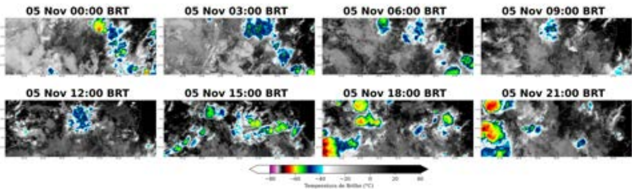
Figura 4: Imagens realçadas do satélite GOES-16 das 00 BRT até 21 BRT (a cada 3 horas) para o dia 05 de novembro.
