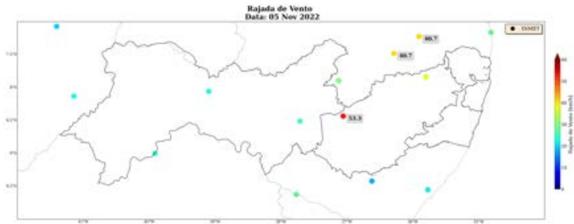
Figura 24: Rajada de vento sobre o estado de Pernambuco para o dia 05 de novembro, baseado nas estações meteorológicas do INMET
