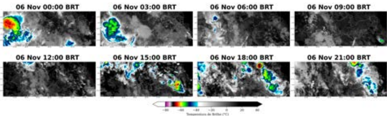
Figura 5: Imagens realçadas do satélite GOES-16 das 00 BRT até 21 BRT (a cada 3 horas) para o dia 06 de novembro.
