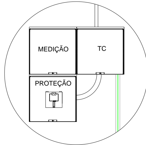
ILUSTRAÇÃO 12 ARRANJO DE CAIXAS DE POLICARBONATO FRONTAL EM ALVENARIA
