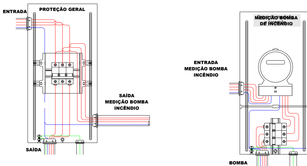
ILUSTRAÇÃO 9 PROTEÇÃO GERAL DESLOCADA COM BOMBA DE INCÊNDIO
