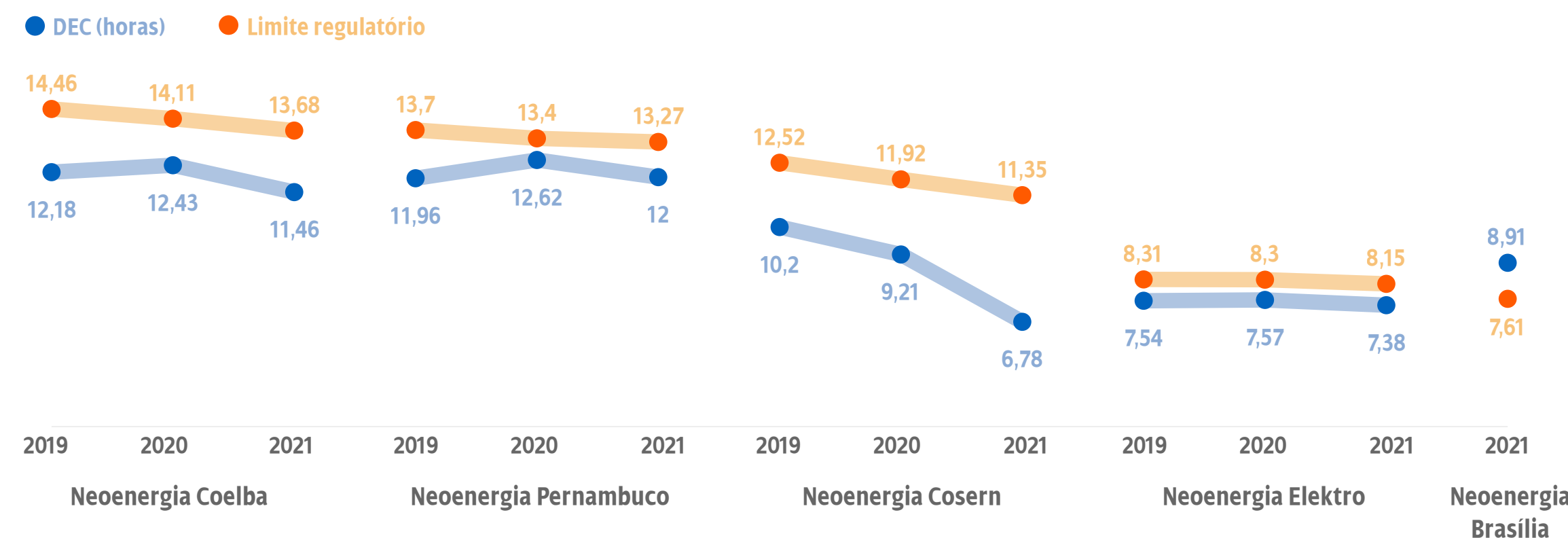
DURAÇÃO DE INTERRUPÇÕES – DEC (HORAS) | GRI EU29 | ■ ODS 1.4 ■ ODS 7.1 SASB IF-EU-550a
