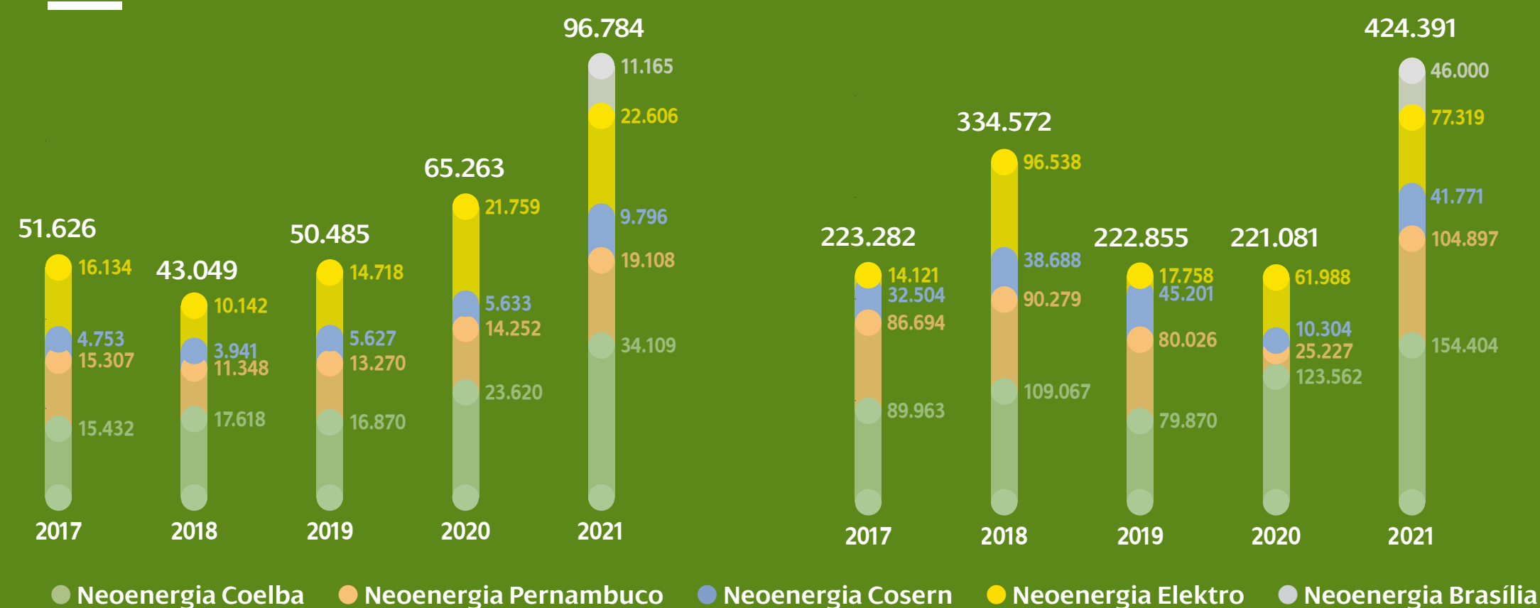
INVESTIMENTO EM EFICIÊNCIA ENERGÉTICA (R$ mil)
