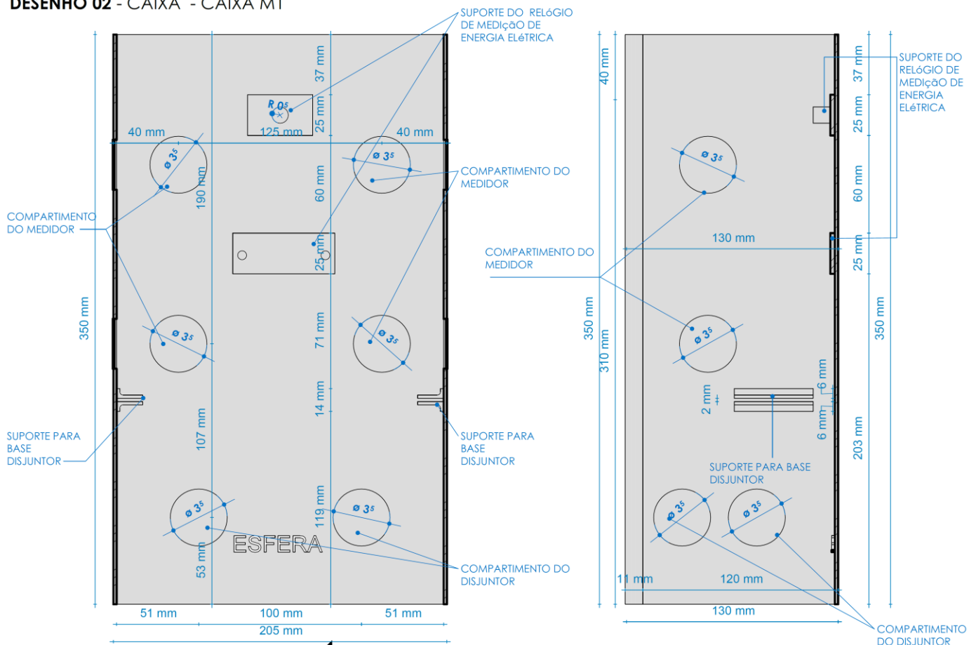
CORTE AA ESC: 1 : 3
