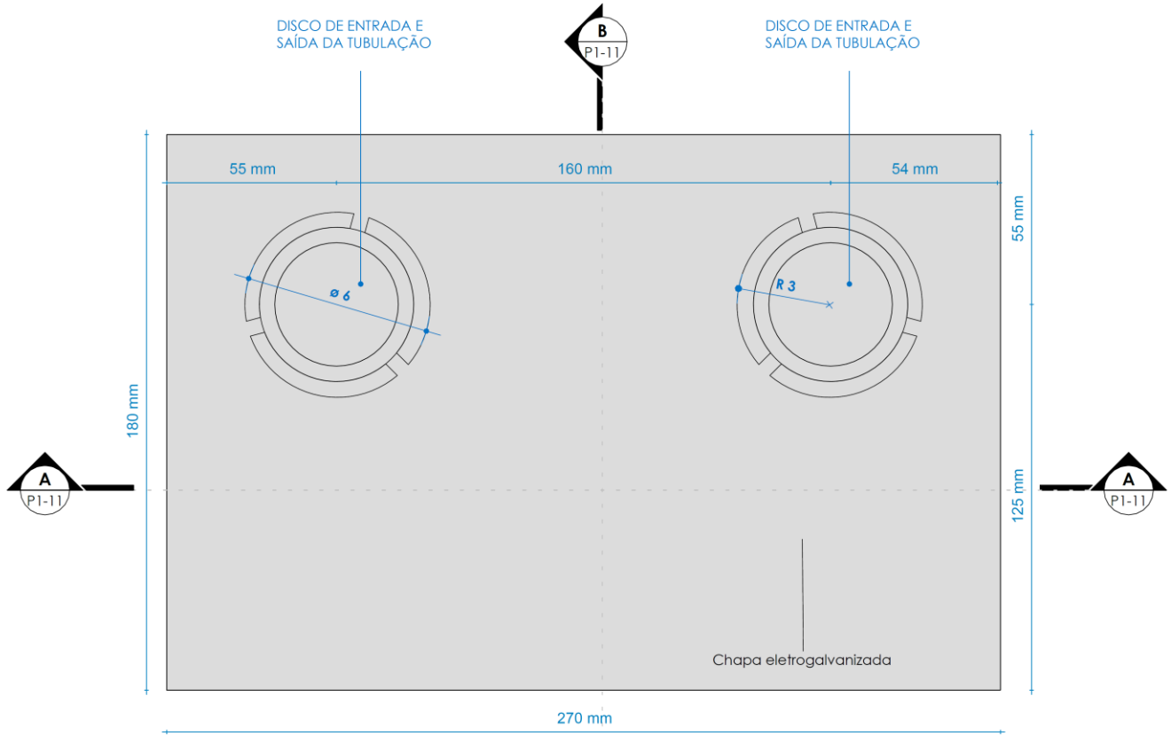
DESENHO 01 - TAMPA SUPERIOR - CAIXA P1
