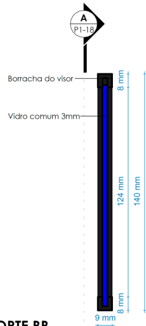
CORTE BB ESC: 1 : 2
