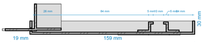
CORTE BB ESC: 1 : 2
