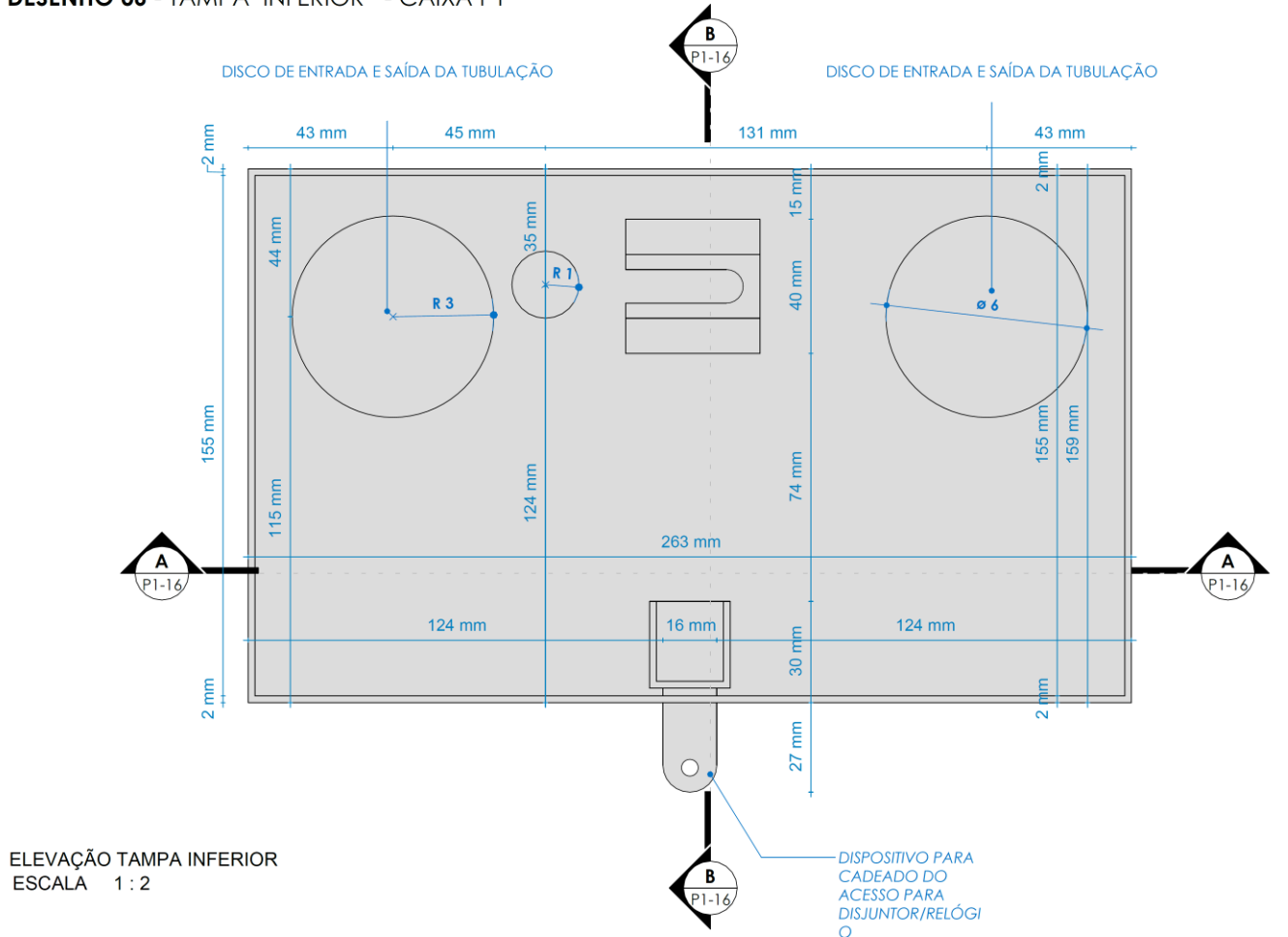
DESENHO 06 - TAMPA INFERIOR - CAIXA P1
