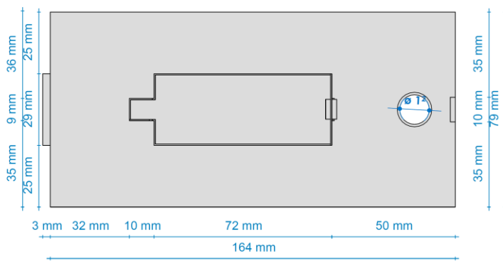
DETALHE A ESC: 1 : 2
