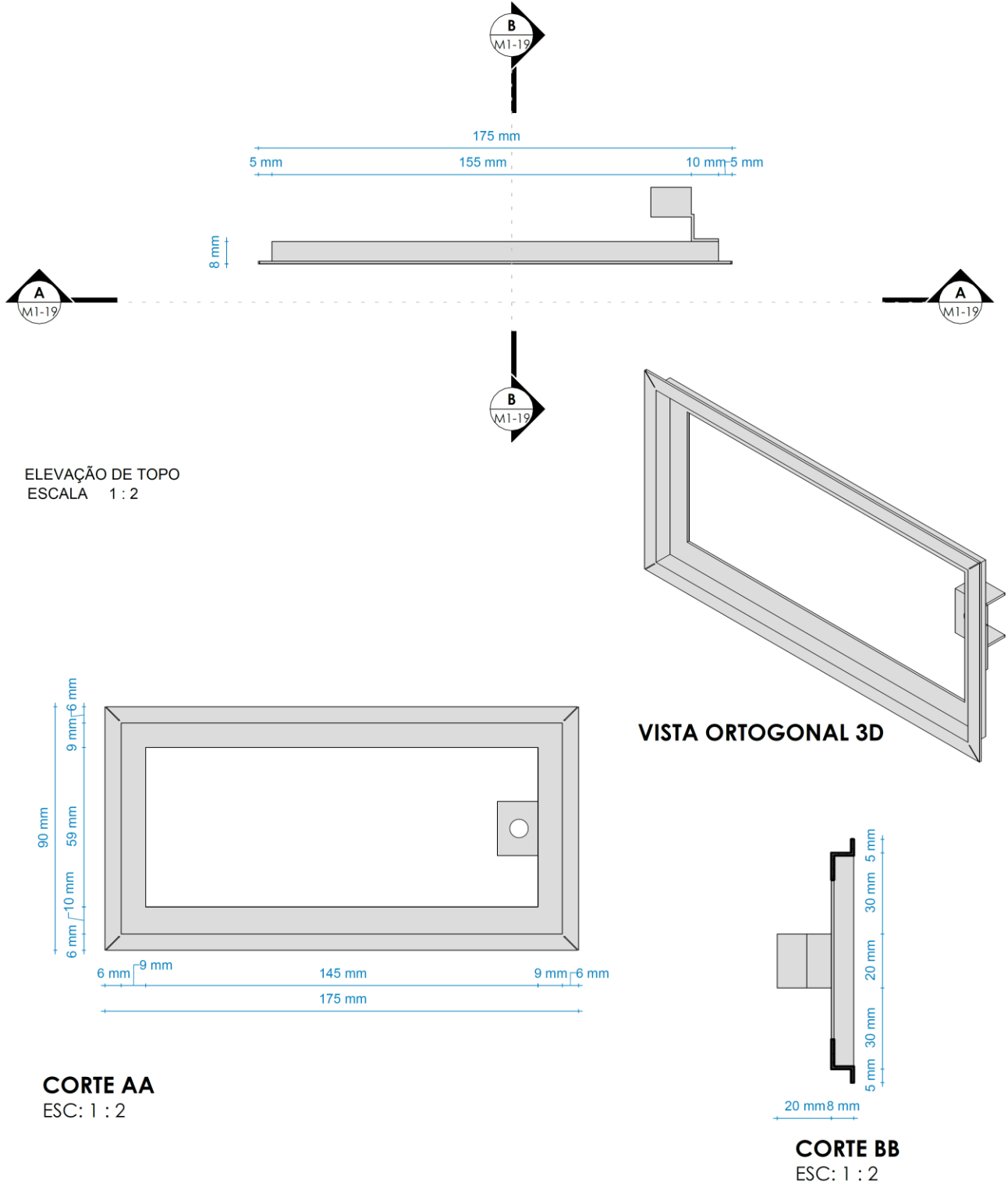
DESENHO 09 - TAMPA POSTERIOR DO ACESSO AO DJUNTOR CAIXA M1
