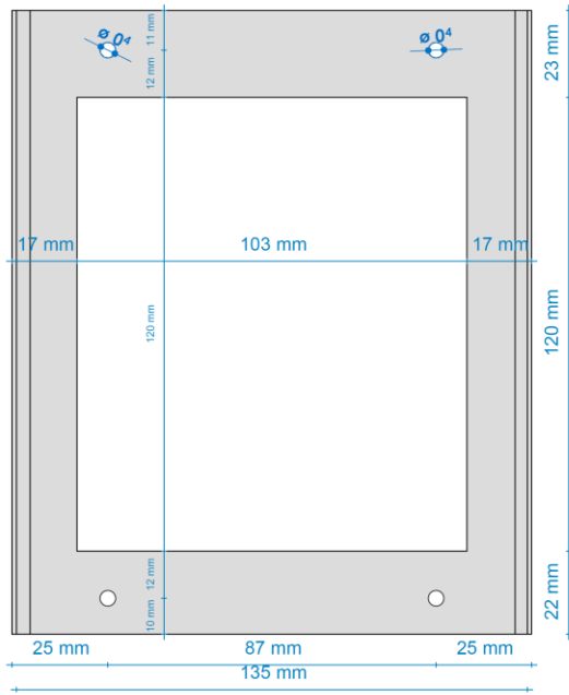
ELEVAÇÃO FRONTAL ESCALA 1 : 2
