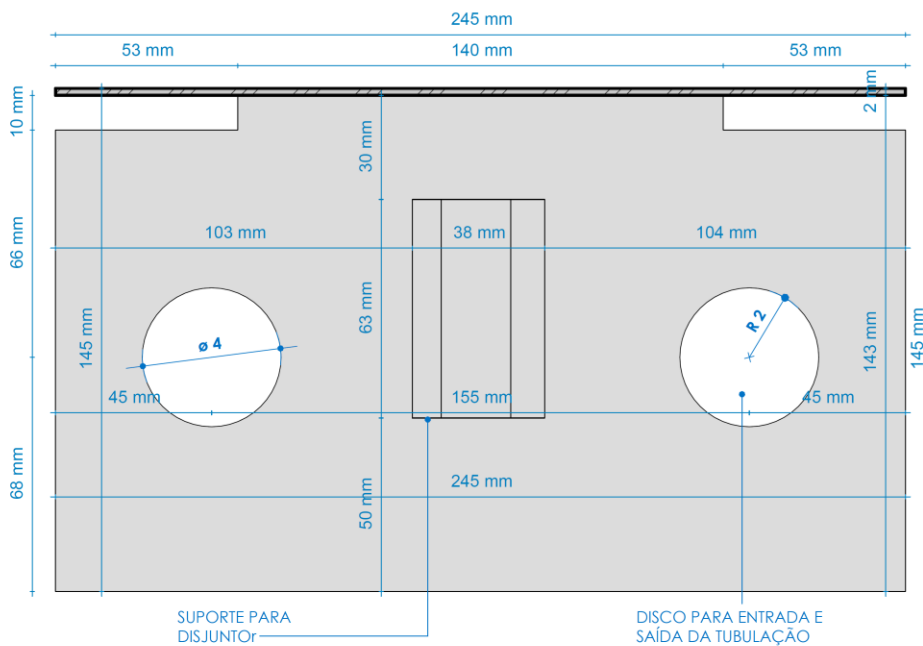
CORTE AA
