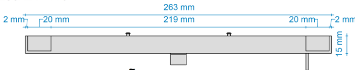
DETALHE ELEVAÇÃO DE TOPO ESC: 1 : 3
