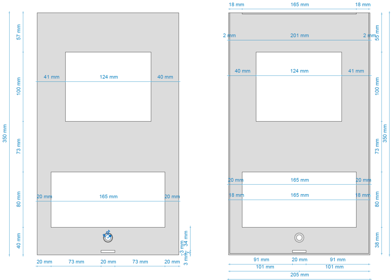
ELEVAÇÃO FRONTAL ESCALA 1 : 3
