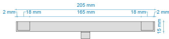
DETALHE ELEVAÇÃO DE TOPO ESC:1 : 3
