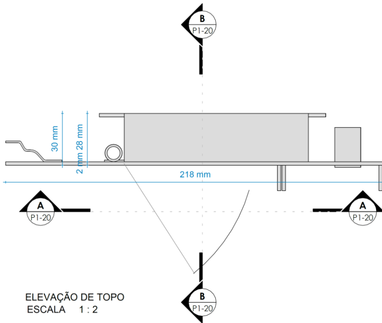
DESENHO 10 - TAMPA DE ACESSO DO DJUNTOR - CAIXA P1
