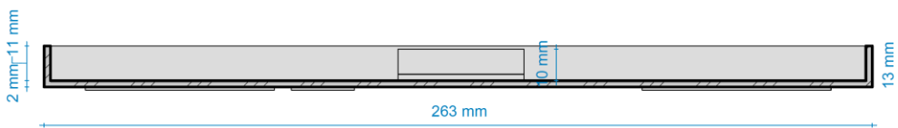
CORTE ÀA ESC: 1 : 2
