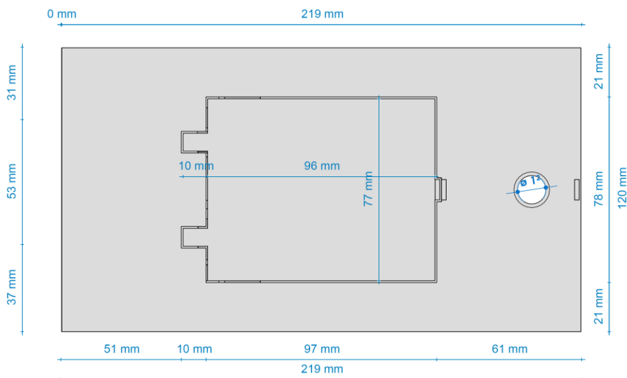
DETALHE A ESC: 1 : 2
