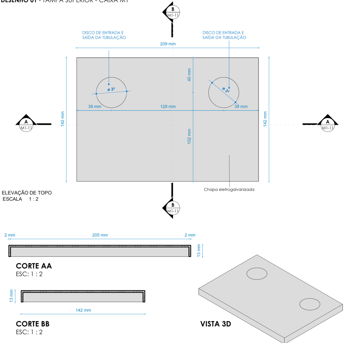
DESENHO 01 - TAMPA SUPERIOR - CAIXA M1
