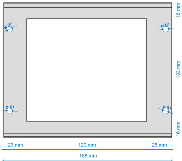
ELEVAÇÃO FRONTAL ESCALA 1 : 2
