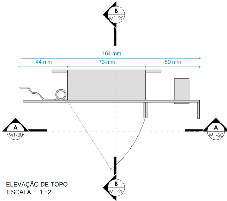
DESENHO 10 - TAMPA DE ACESSO AO DJUNTOR - CAIXA M1
