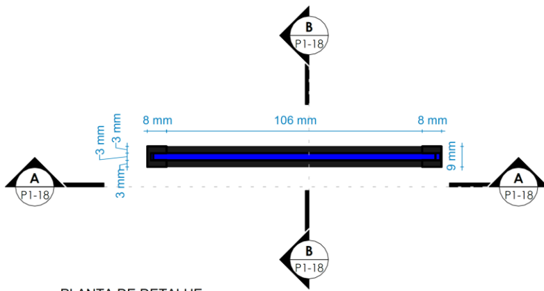
PLANTA DE DETALHE ESCALA 1 : 2
