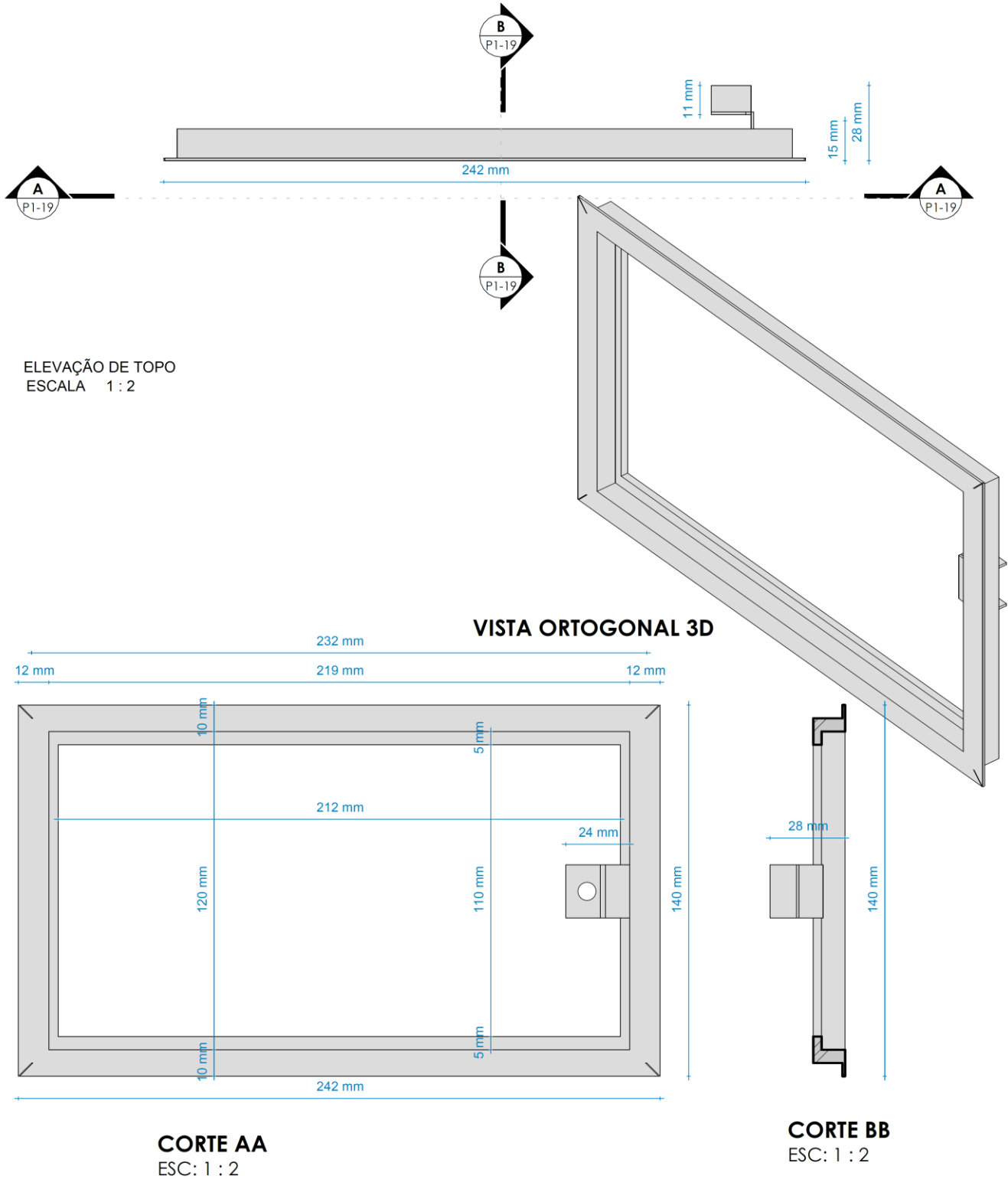
DESENHO 09 - TAMPA POSTERIOR DO ACESSO AO DJUNTOR CAIXA P1
