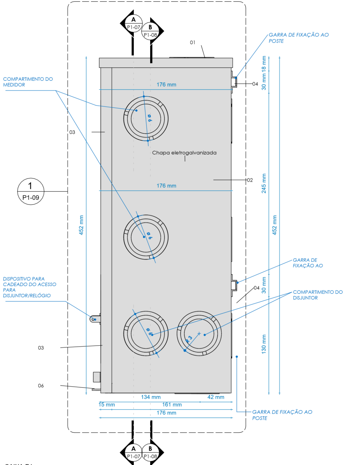
VISTA LATERAL - CAIXA P1
