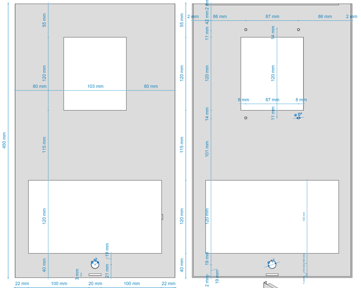
ELEVAÇÃO FRONTAL ESCALA 1 : 3
