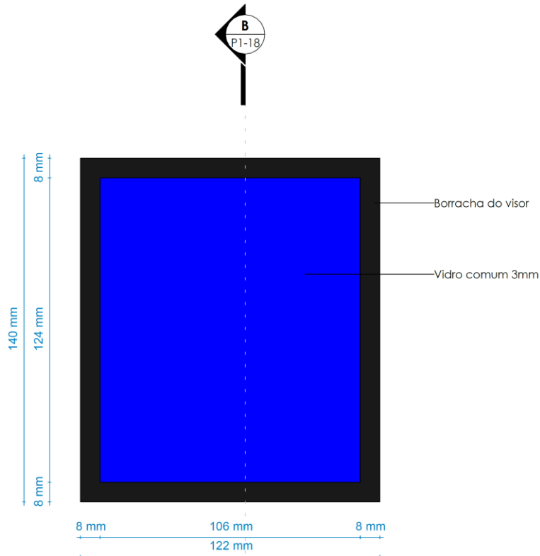
CORTE AA ESC: 1 : 2
