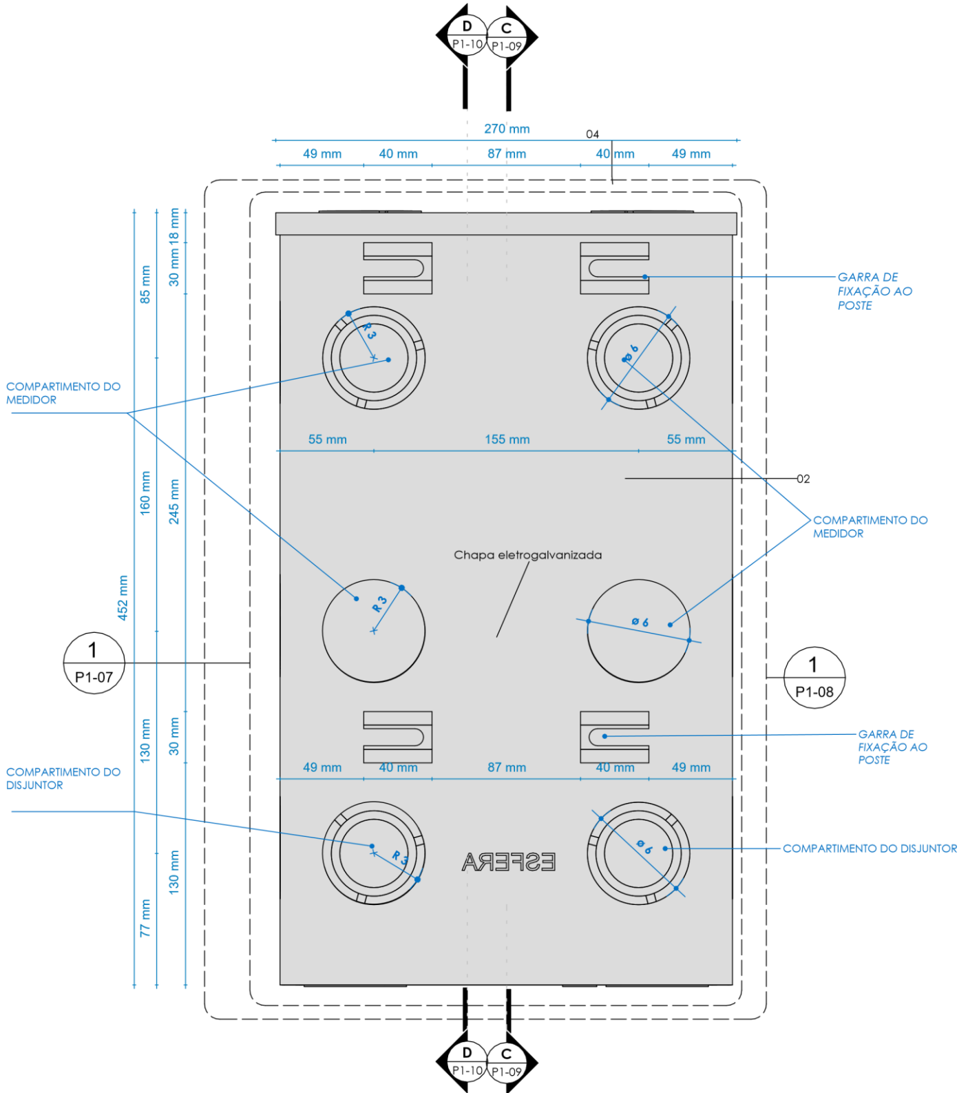
VISTA POSTERIOR - CAIXA P1 ESCALA 1:3
