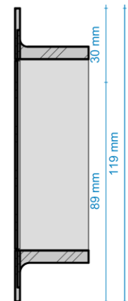
DETALHE B ESC: 1 : 2
