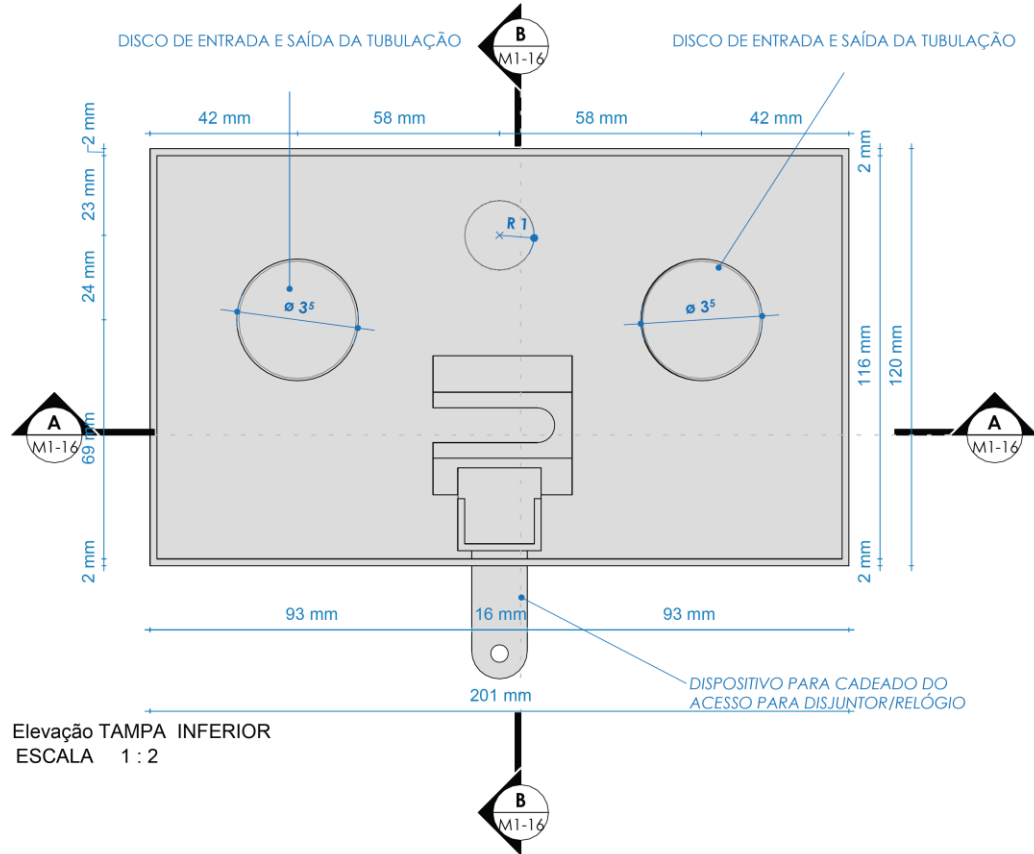
DESENHO 06 - TAMPA INFERIOR - CAIXA M1
