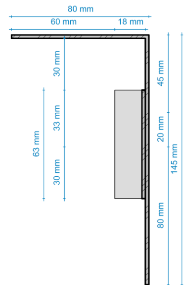
CORTE B
