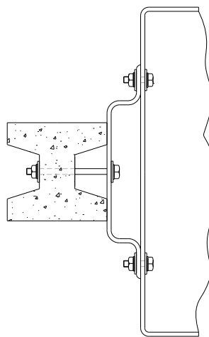
Corte B-B
