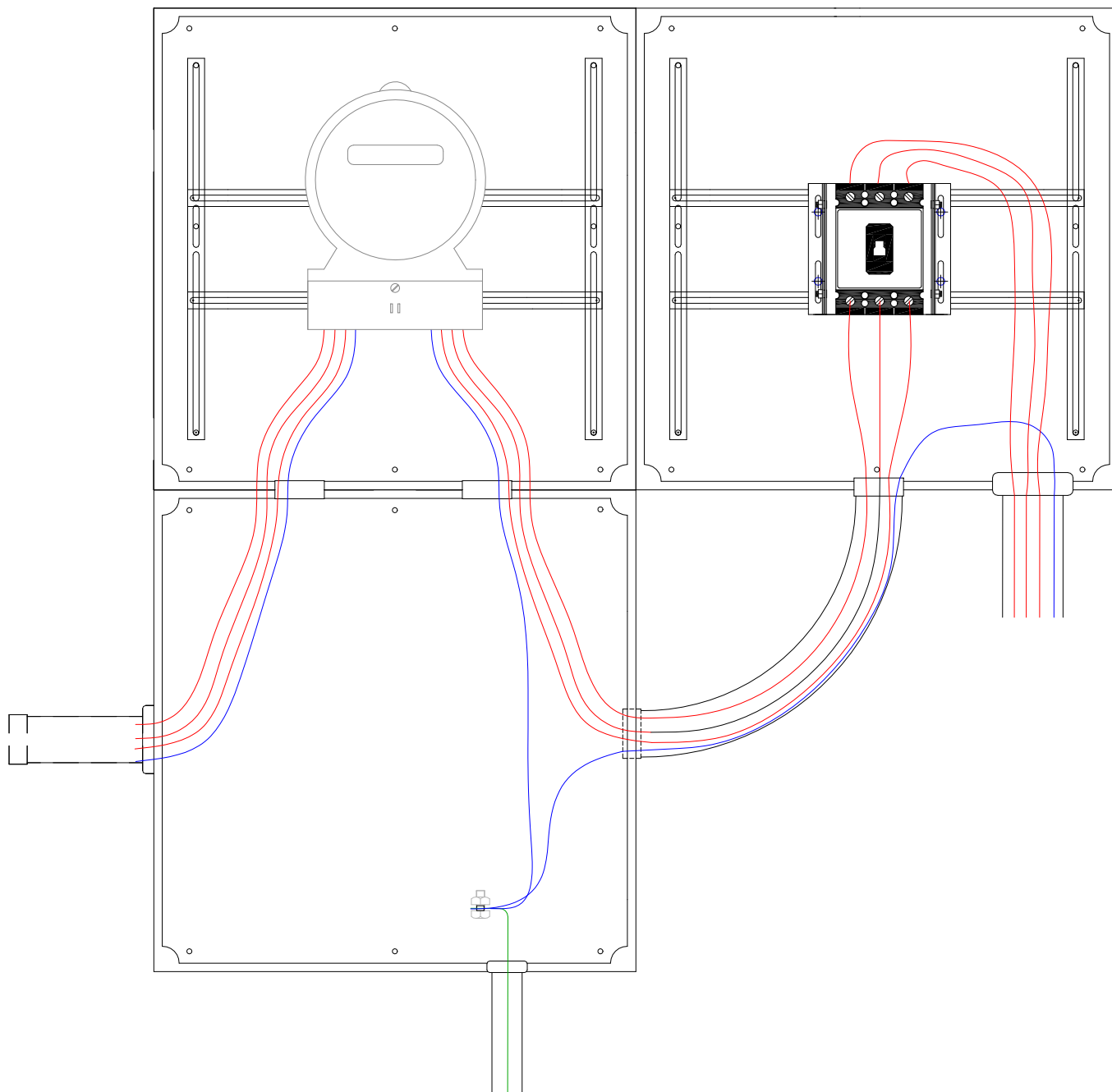
Figura 16c – Detalhes de Ligação do Medidor Polifásico – 3/3
