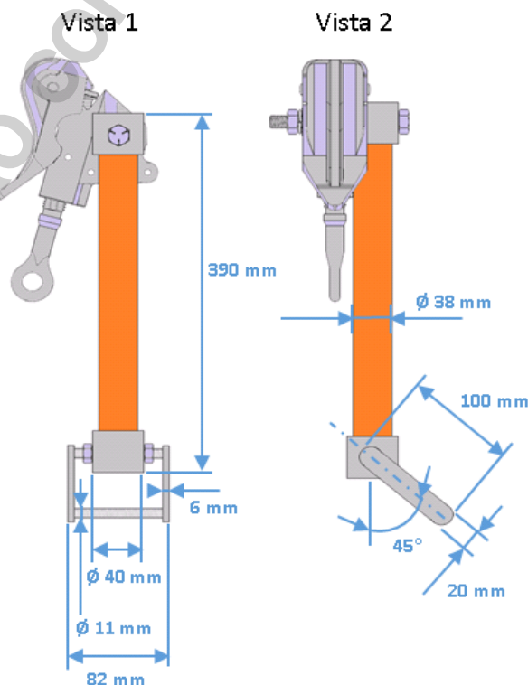
Suporte de 390 mm
