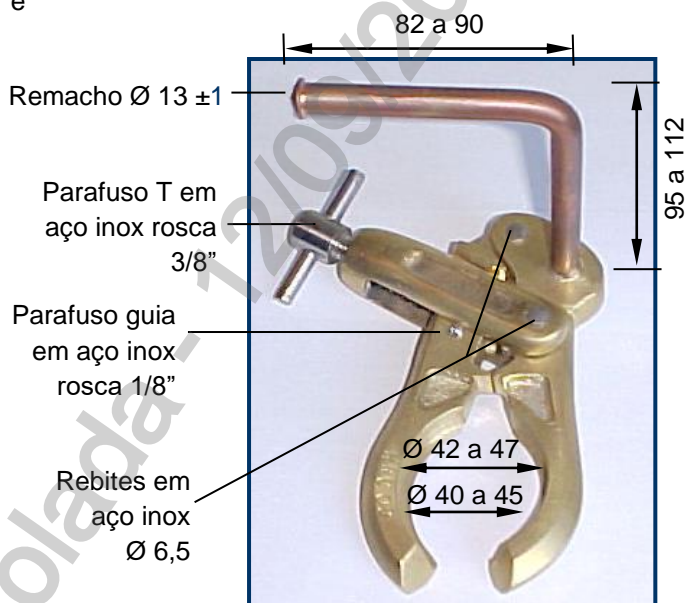
*Dimensões em milímetros.
