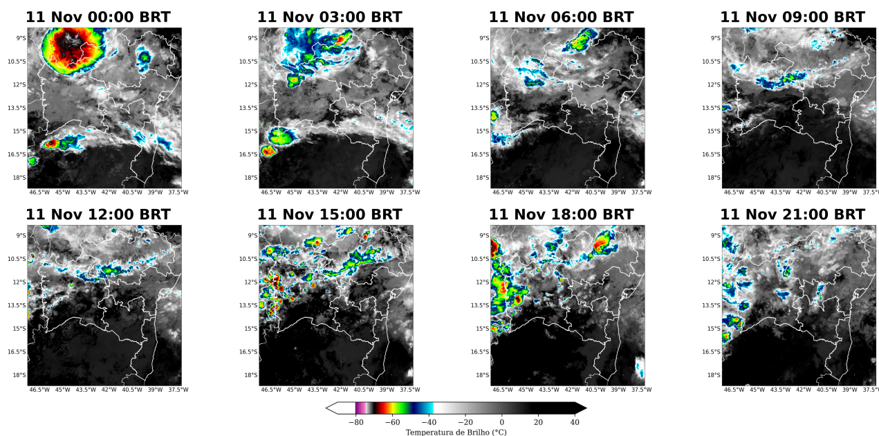
Figura 6: Imagens realçadas do satélite GOES-16 das 00 BRT até 21 BRT (a cada 3 horas) para o dia 11 de novembro.
