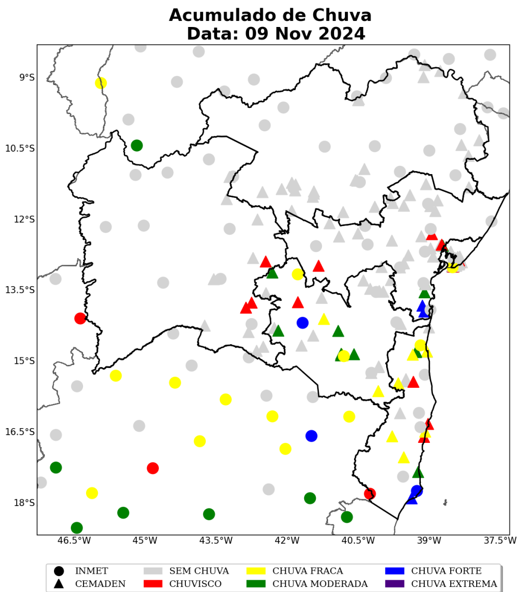
Figura 21: Acumulado diário de precipitação sobre o estado de Bahia para o dia 09 de novembro, baseado nas estações meteorológicas do INMET e CEMADEN.
