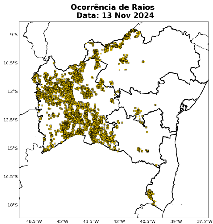
Figura 4 – Mapa de descargas atmosféricas sobre o estado da Bahia no dia 13 de novembro.
