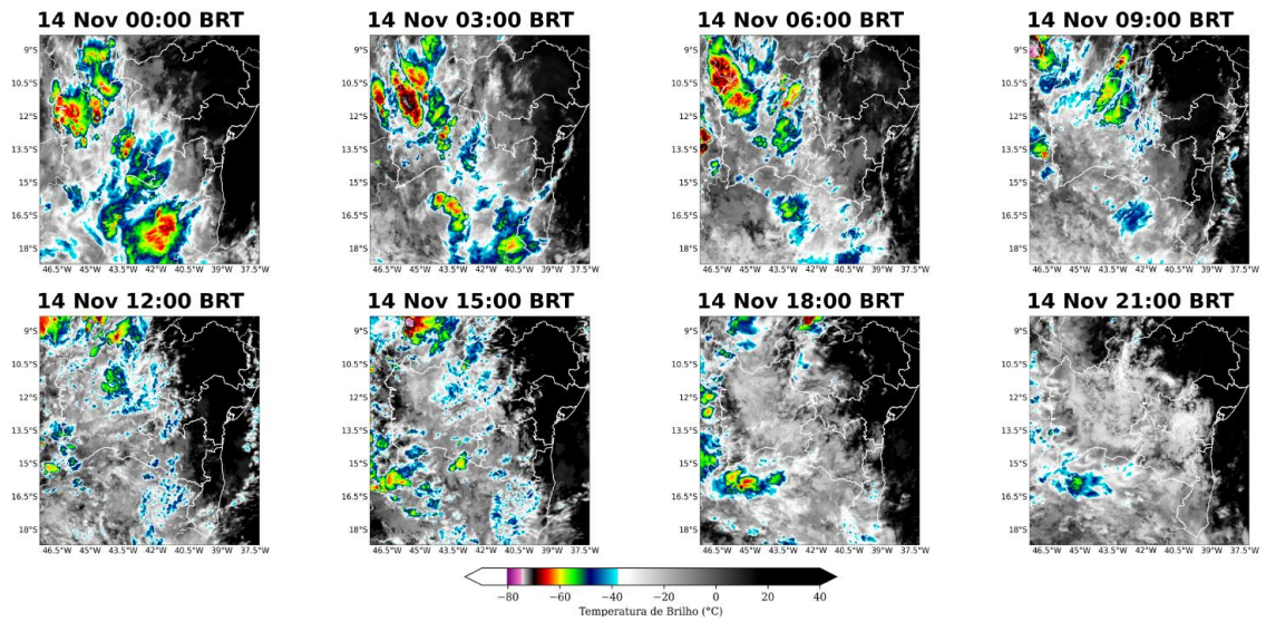
Figura 13 – Imagens realçadas do satélite GOES-16 das 00h00, 03h00, 06h00, 09h00, 12h00, 15h00, 18h00, e 21h00 do dia 14 de novembro de 2024. Fonte: Climatempo
