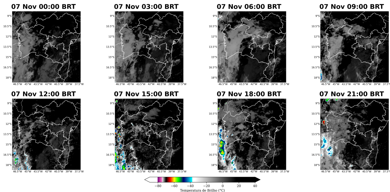
Figura 2: Imagens realçadas do satélite GOES-16 das 00 BRT até 21 BRT (a cada 3 horas) para o dia 07 de novembro.
