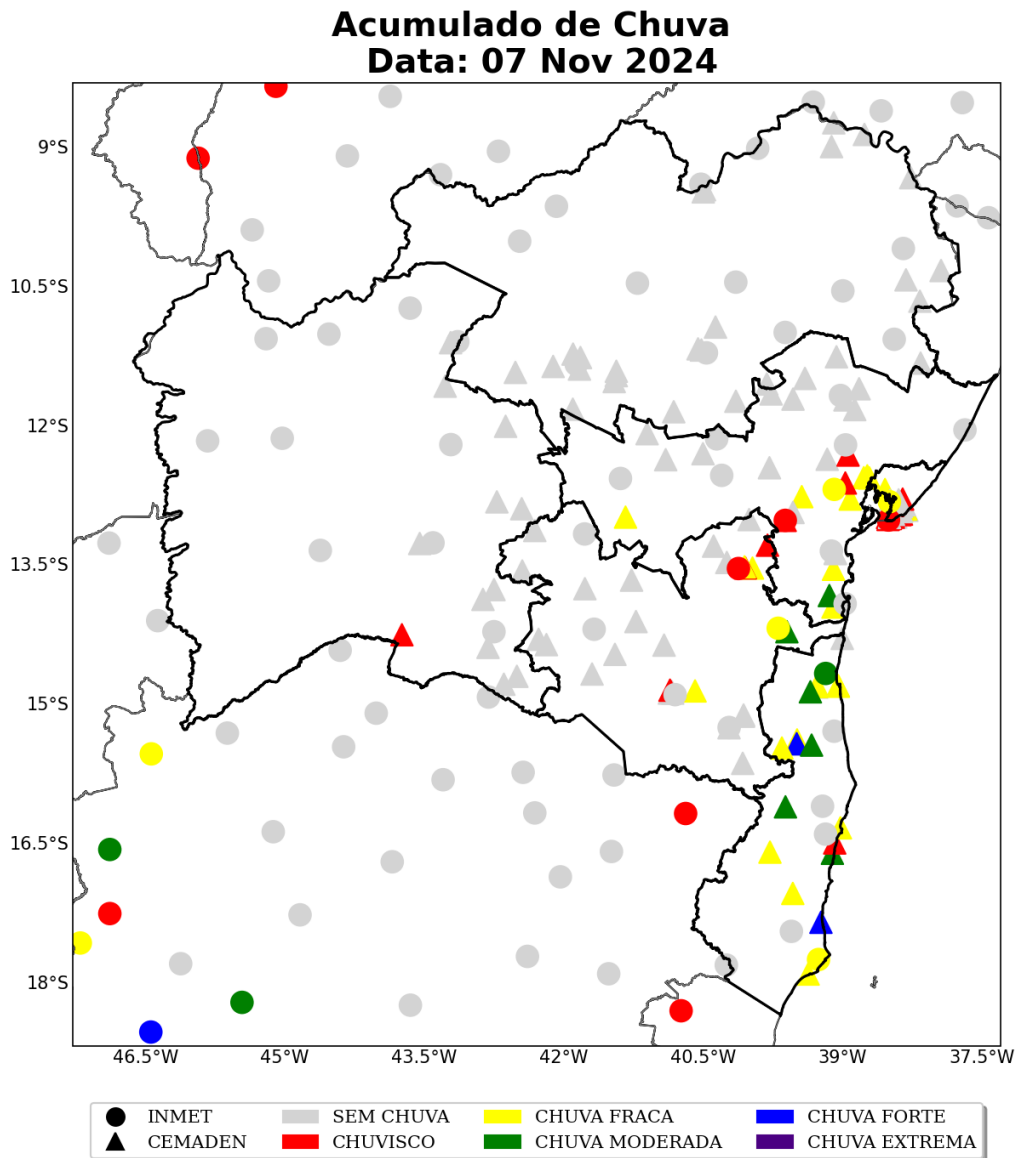
Figura 19: Acumulado diário de precipitação sobre o estado de Bahia para o dia 07 de novembro, baseado nas estações meteorológicas do INMET e CEMADEN.
