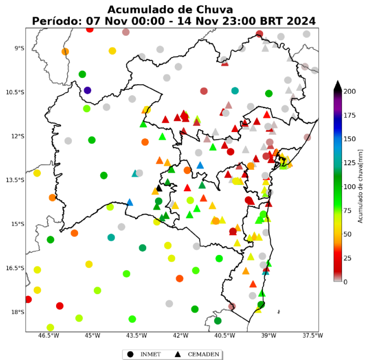
Figura 7 – Mapa de precipitação acumulada de 07 a 14 de novembro.
