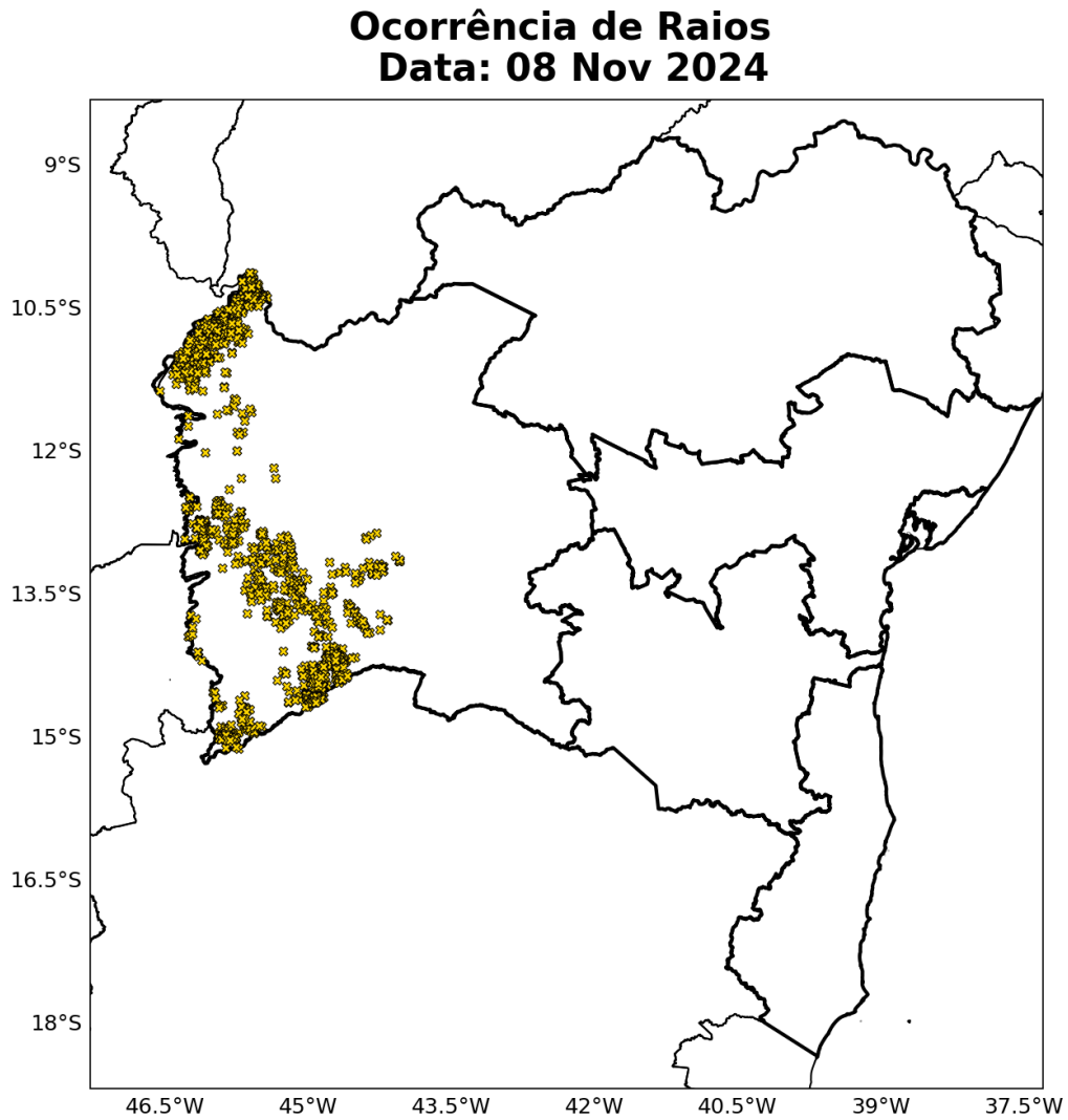
Figura 11: Ocorrência de descargas atmosféricas nuvem-solo detectadas pelo sistema Earth Networks para o dia 08 de novembro sobre a área de concessão da Neoenergia-COELBA.
