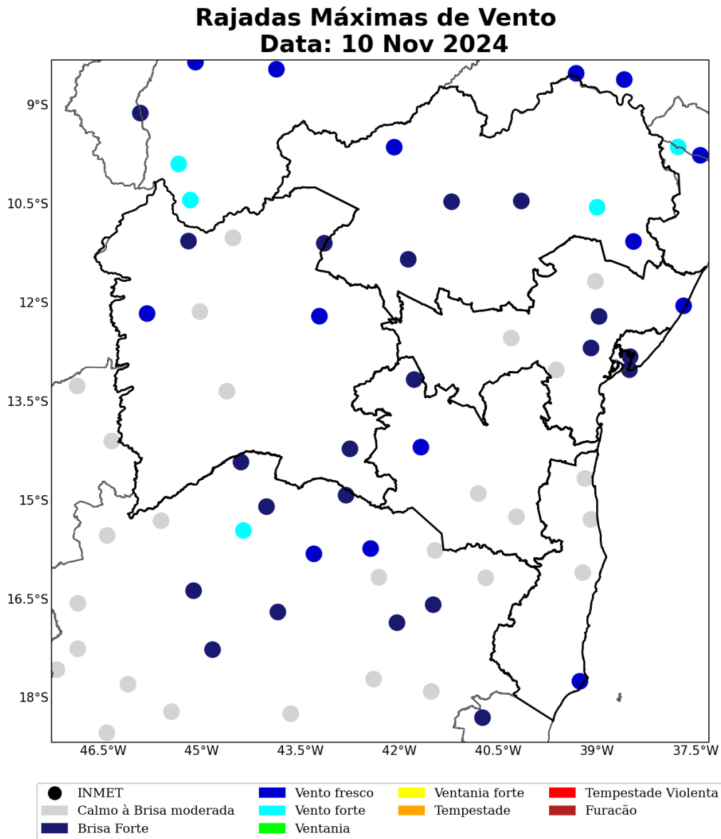
Figura 31: Rajada de vento sobre o estado de Bahia para o dia 10 de novembro, baseado nas estações meteorológicas do INMET.
