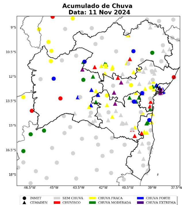
Figura 2 – Mapa de precipitação sobre o estado da Bahia no dia 11 de novembro.
