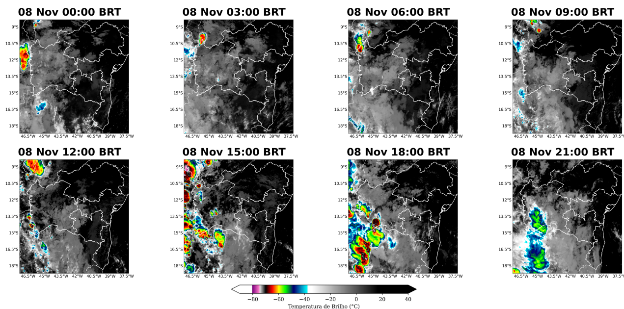
Figura 3: Imagens realçadas do satélite GOES-16 das 00 BRT até 21 BRT (a cada 3 horas) para o dia 08 de novembro.
