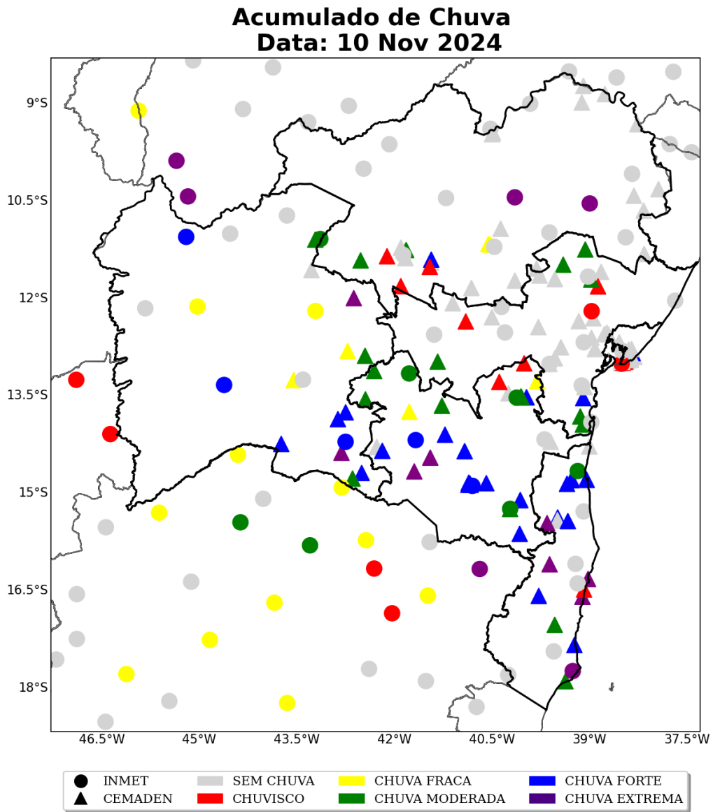
Figura 22: Acumulado diário de precipitação sobre o estado de Bahia para o dia 10 de novembro, baseado nas estações meteorológicas do INMET e CEMADEN.
