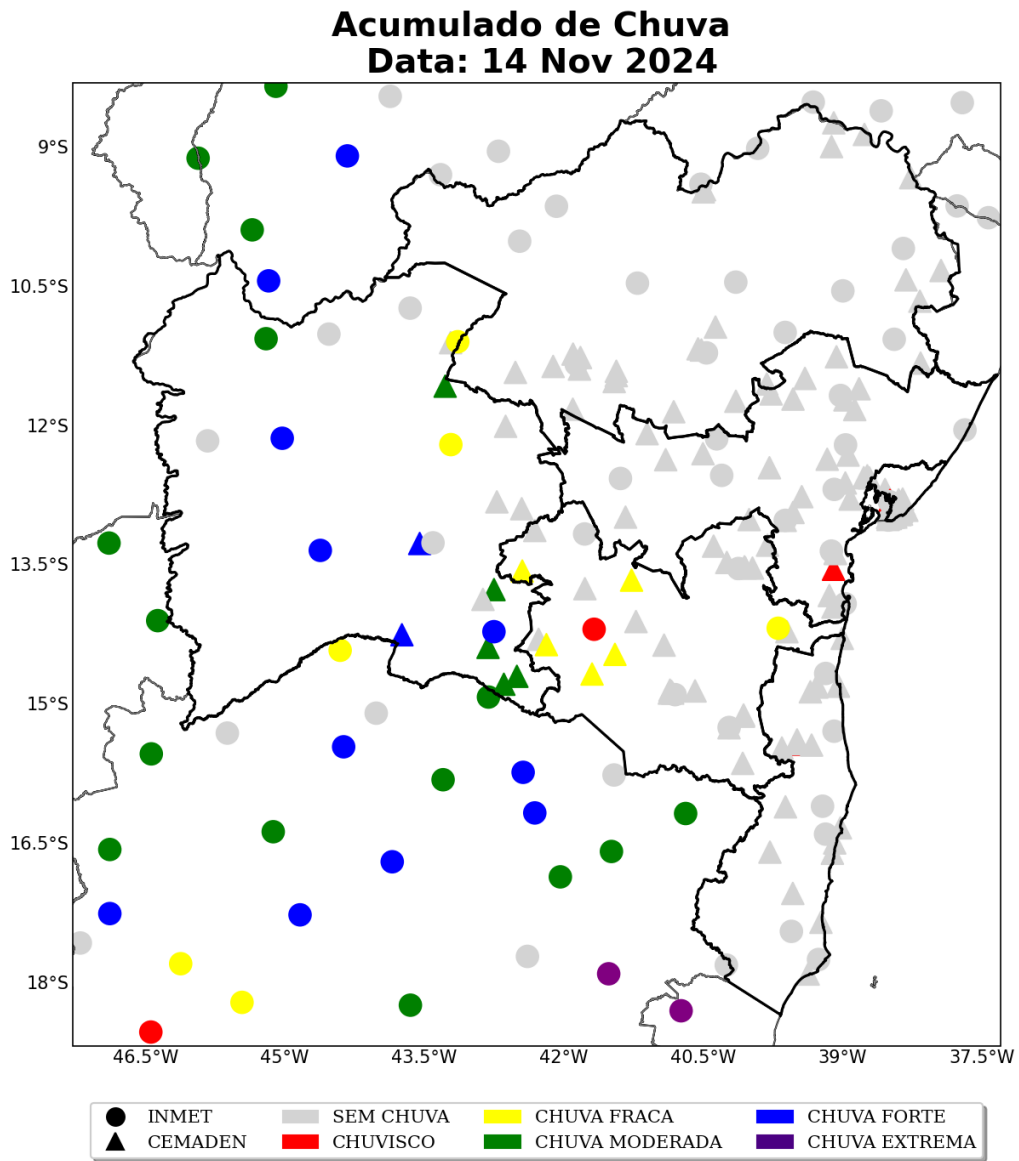
Figura 26: Acumulado diário de precipitação sobre o estado de Bahia para o dia 14 de novembro, baseado nas estações meteorológicas do INMET e CEMADEN.
