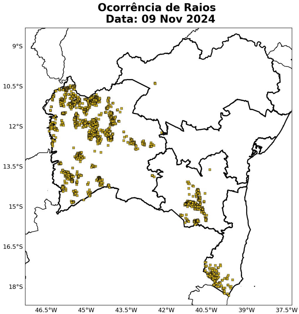
Figura 12: Ocorrência de descargas atmosféricas nuvem-solo detectadas pelo sistema Earth Networks para o dia 09 de novembro sobre a área de concessão da Neoenergia-COELBA.
