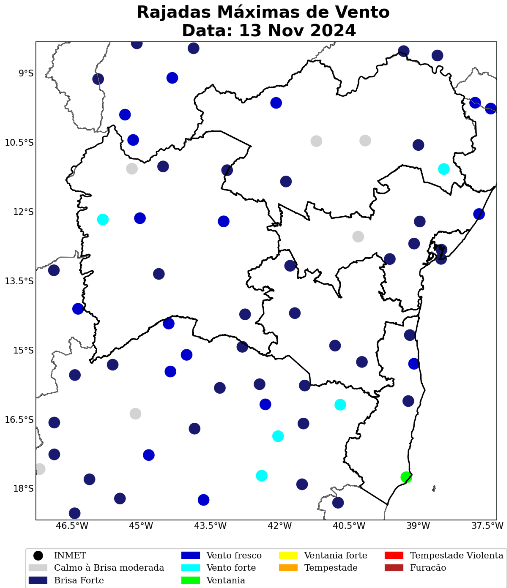
Figura 34: Rajada de vento sobre o estado de Bahia para o dia 13 de novembro, baseado nas estações meteorológicas do INMET.
