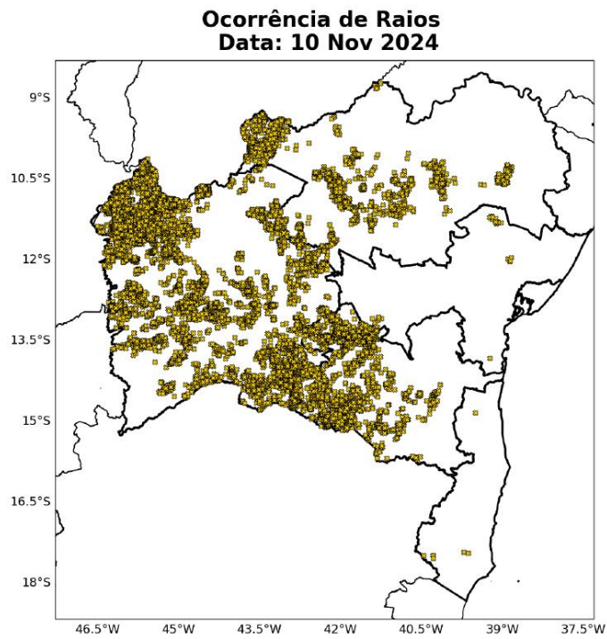
Figura 3 – Mapa de descargas atmosféricas sobre o estado da Bahia no dia 10 de novembro.
