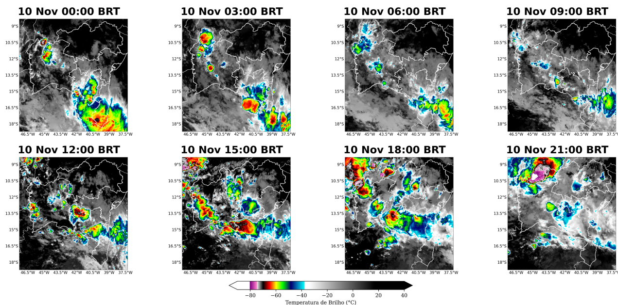
Figura 5: Imagens realçadas do satélite GOES-16 das 00 BRT até 21 BRT (a cada 3 horas) para o dia 10 de novembro.
