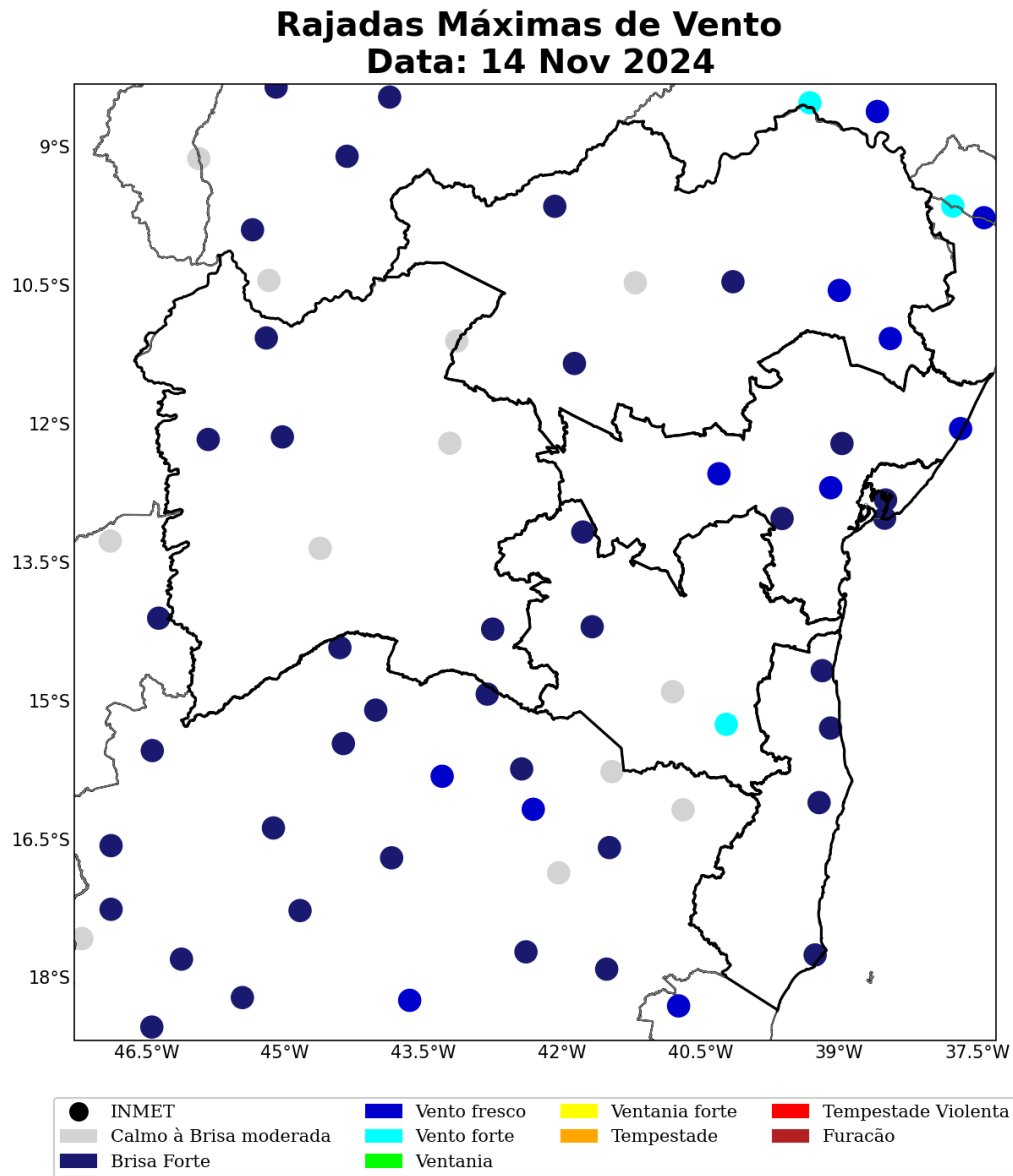
Figura 35: Rajada de vento sobre o estado de Bahia para o dia 14 de novembro, baseado nas estações meteorológicas do INMET.
