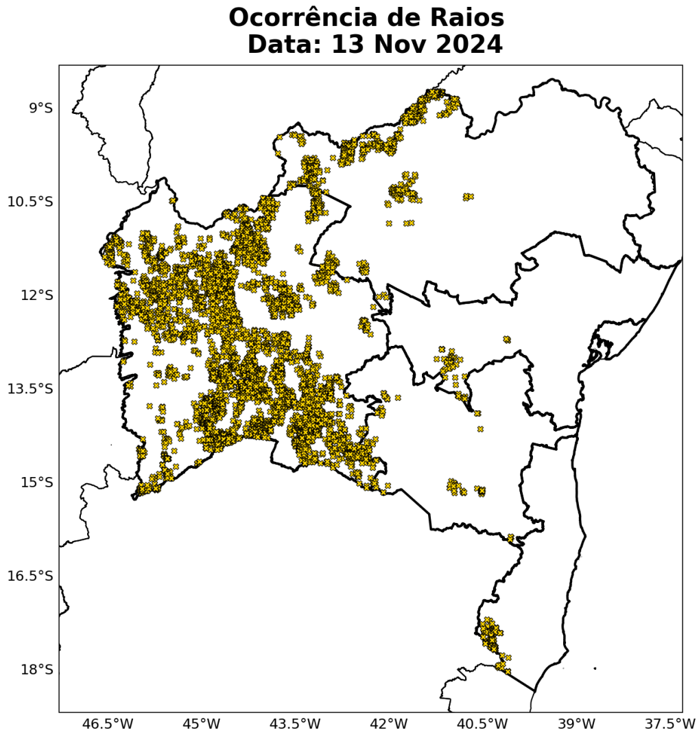
Figura 16: Ocorrência de descargas atmosféricas nuvem-solo detectadas pelo sistema Earth Networks para o dia 13 de novembro sobre a área de concessão da Neoenergia-COELBA.
