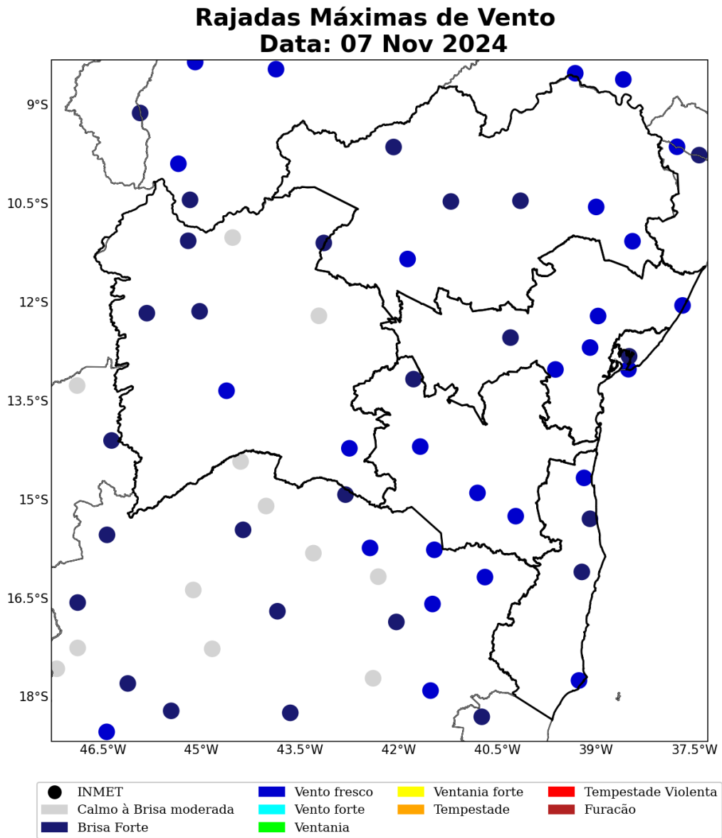
Figura 28: Rajada de vento sobre o estado de Bahia para o dia 07 de novembro, baseado nas estações meteorológicas do INMET.
