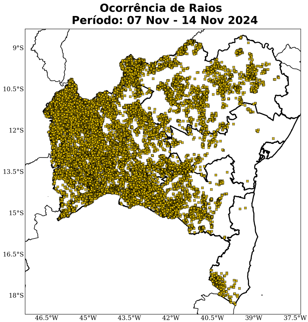
Figura 18: Ocorrência de descargas atmosféricas nuvem-solo detectadas pelo sistema Earth Networks para o período de 07 a 14 de novembro de 2024 sobre a área de concessão da Neoenergia-COELBA.
