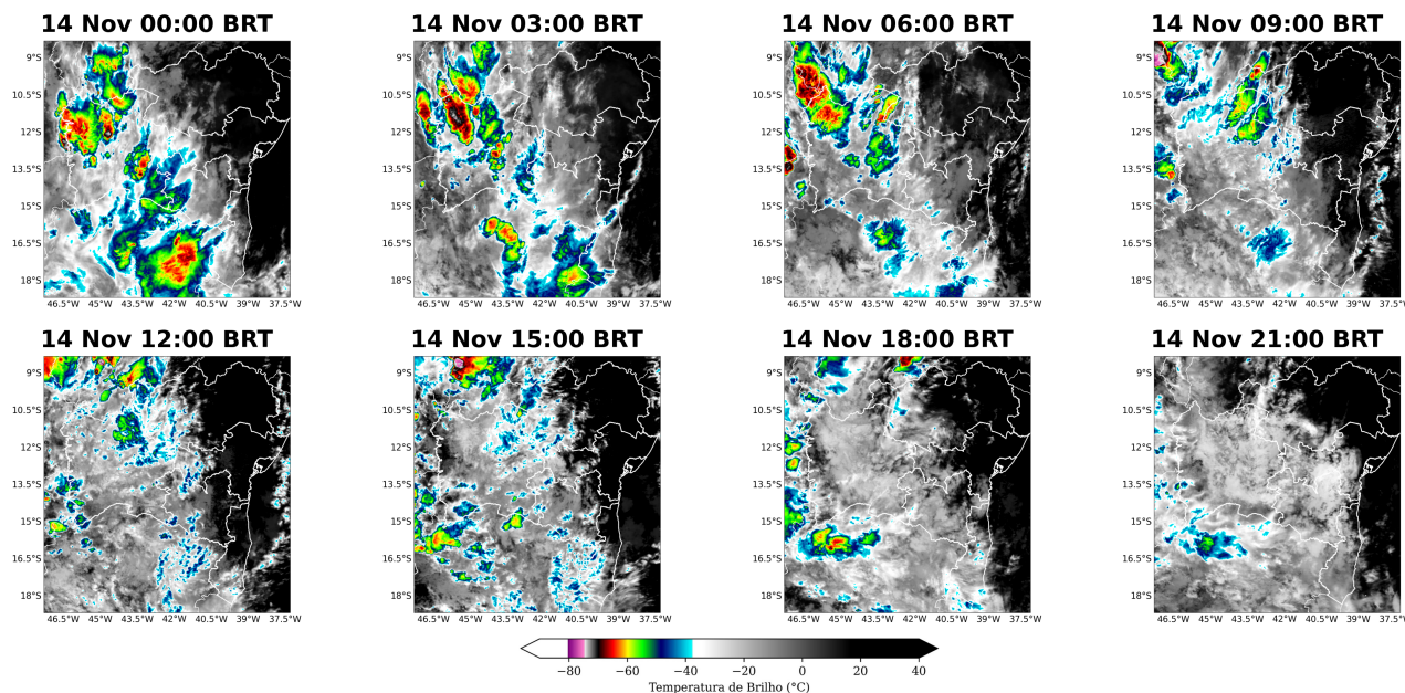
Figura 9: Imagens realçadas do satélite GOES-16 das 00 BRT até 21 BRT (a cada 3 horas) para o dia 14 de novembro.
