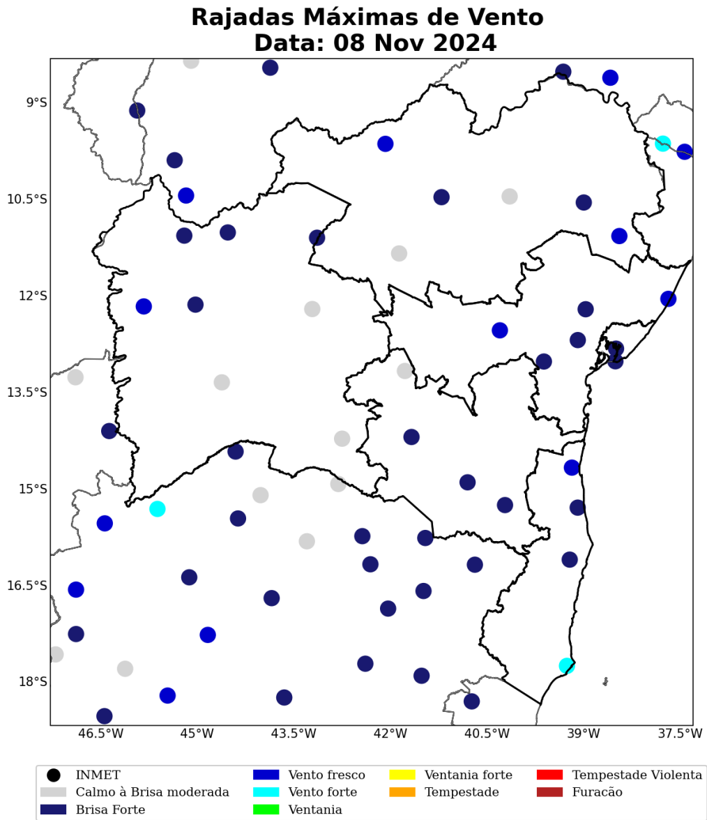
Figura 29: Rajada de vento sobre o estado de Bahia para o dia 08 de novembro, baseado nas estações meteorológicas do INMET.
