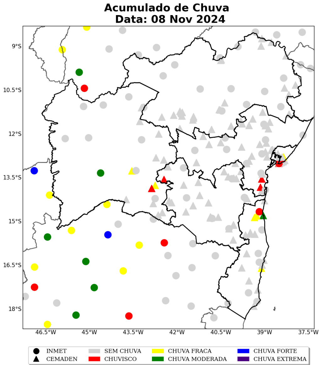
Figura 20: Acumulado diário de precipitação sobre o estado de Bahia para o dia 08 de novembro, baseado nas estações meteorológicas do INMET e CEMADEN.
