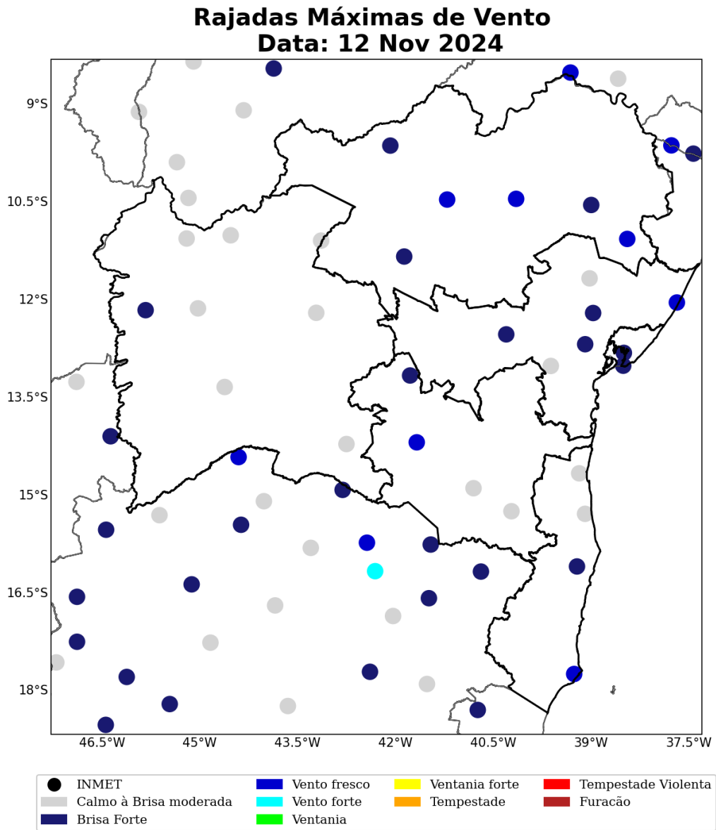
Figura 33: Rajada de vento sobre o estado de Bahia para o dia 12 de novembro, baseado nas estações meteorológicas do INMET.
