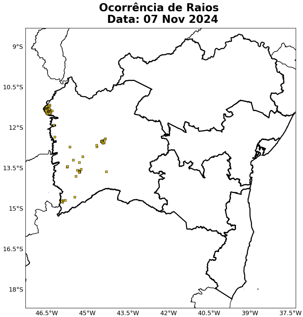
Figura 10: Ocorrência de descargas atmosféricas nuvem-solo detectadas pelo sistema Earth Networks para o dia 07 de novembro sobre a área de concessão da Neoenergia-COELBA.
