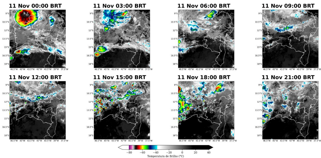
Figura 10 – Imagens realçadas do satélite GOES-16 das 00h00, 03h00, 06h00, 09h00, 12h00, 15h00, 18h00, e 21h00 do dia 11 de novembro de 2024. Fonte: Climatempo
