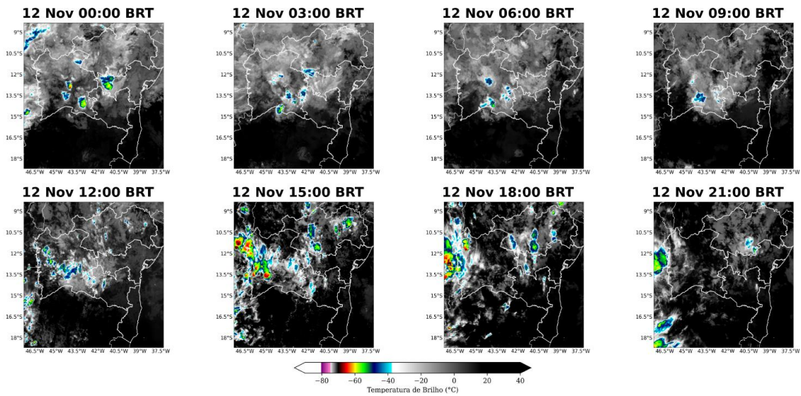
Figura 11 – Imagens realçadas do satélite GOES-16 das 00h00, 03h00, 06h00, 09h00, 12h00, 15h00, 18h00, e 21h00 do dia 12 de novembro de 2024. Fonte: Climatempo
