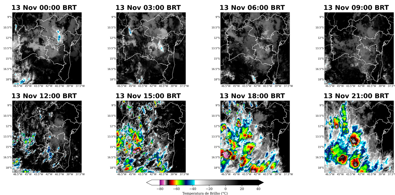
Figura 8: Imagens realçadas do satélite GOES-16 das 00 BRT até 21 BRT (a cada 3 horas) para o dia 13 de novembro.
