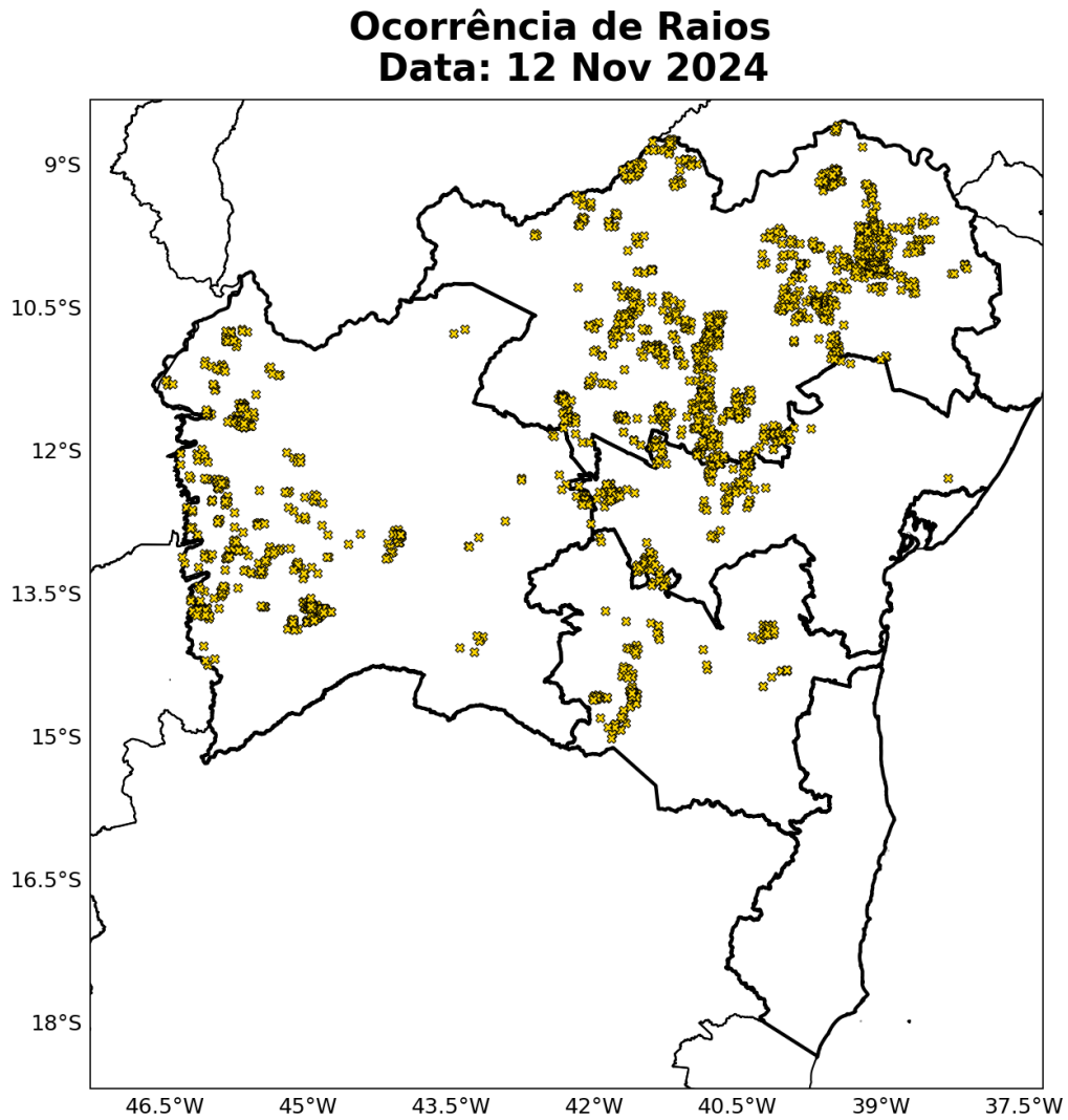
Figura 15: Ocorrência de descargas atmosféricas nuvem-solo detectadas pelo sistema Earth Networks para o dia 12 de novembro sobre a área de concessão da Neoenergia-COELBA.
