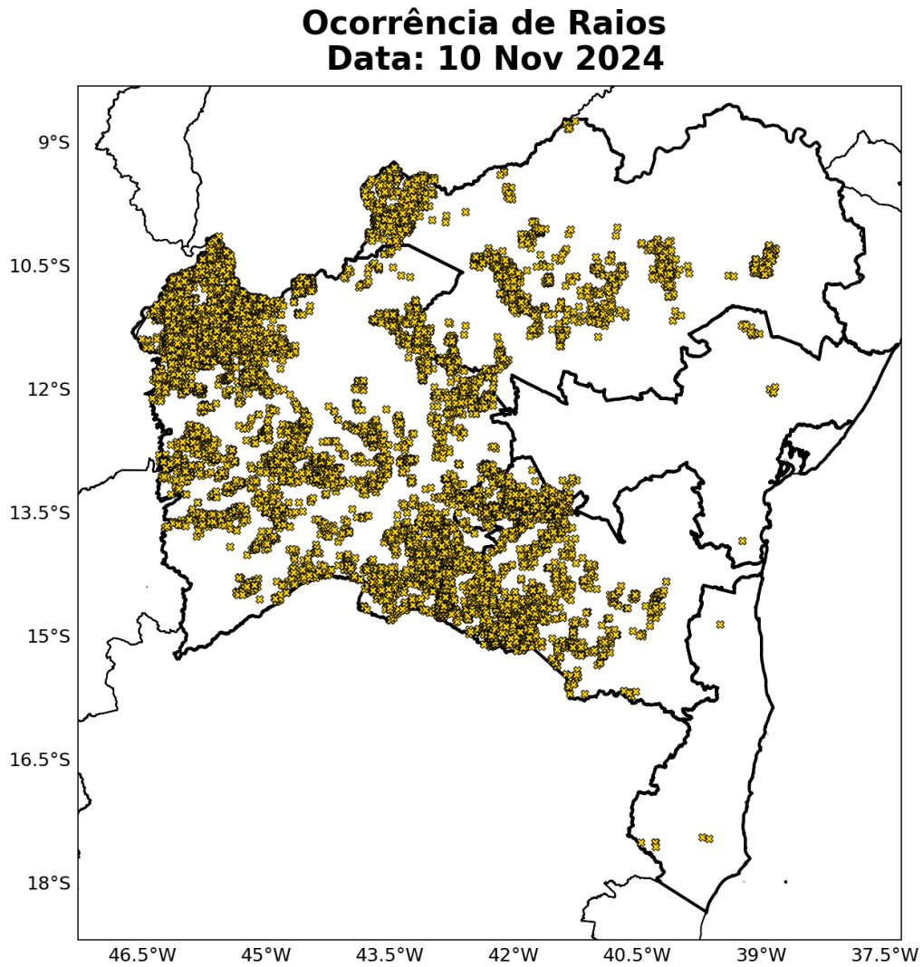
Figura 13: Ocorrência de descargas atmosféricas nuvem-solo detectadas pelo sistema Earth Networks para o dia 10 de novembro sobre a área de concessão da Neoenergia-COELBA.
