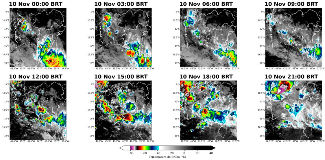
Figura 9 – Imagens realçadas do satélite GOES-16 das 00h00, 03h00, 06h00, 09h00, 12h00, 15h00, 18h00, e 21h00 do dia 10 de novembro de 2024. Fonte: Climatempo
