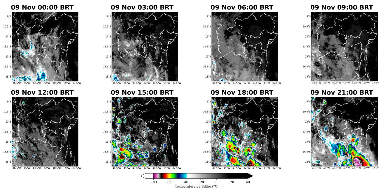
Figura 4: Imagens realçadas do satélite GOES-16 das 00 BRT até 21 BRT (a cada 3 horas) para o dia 09 de novembro.
