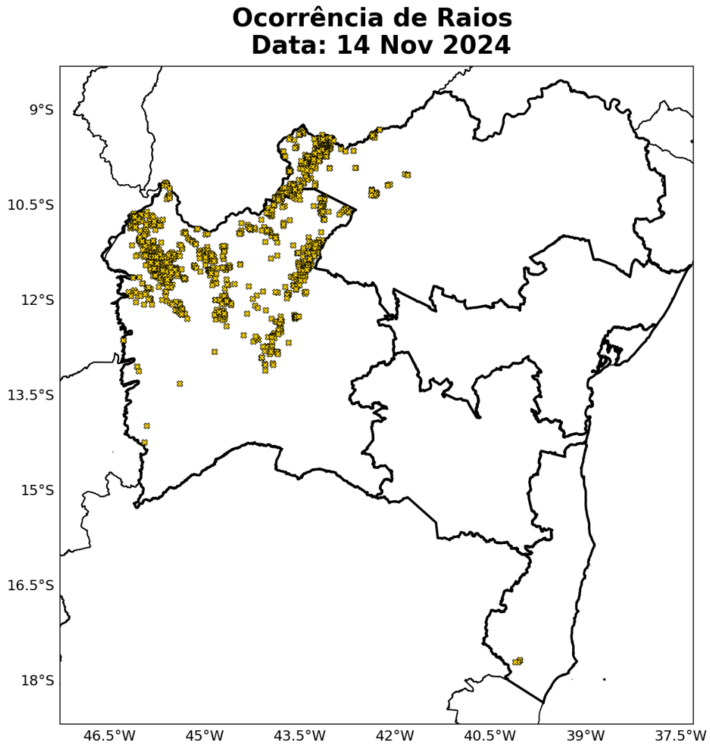
Figura 17: Ocorrência de descargas atmosféricas nuvem-solo detectadas pelo sistema Earth Networks para o dia 14 de novembro sobre a área de concessão da Neoenergia-COELBA.
