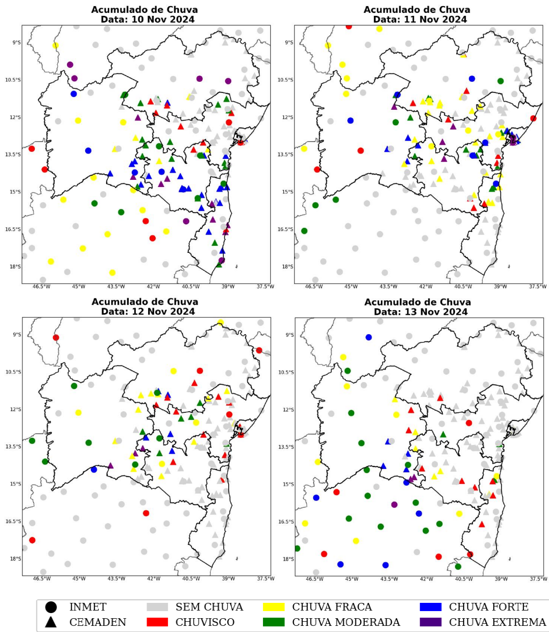
Figura 6 – Mapa de precipitação dos dias 10, 11, 12 e 13 de novembro.
