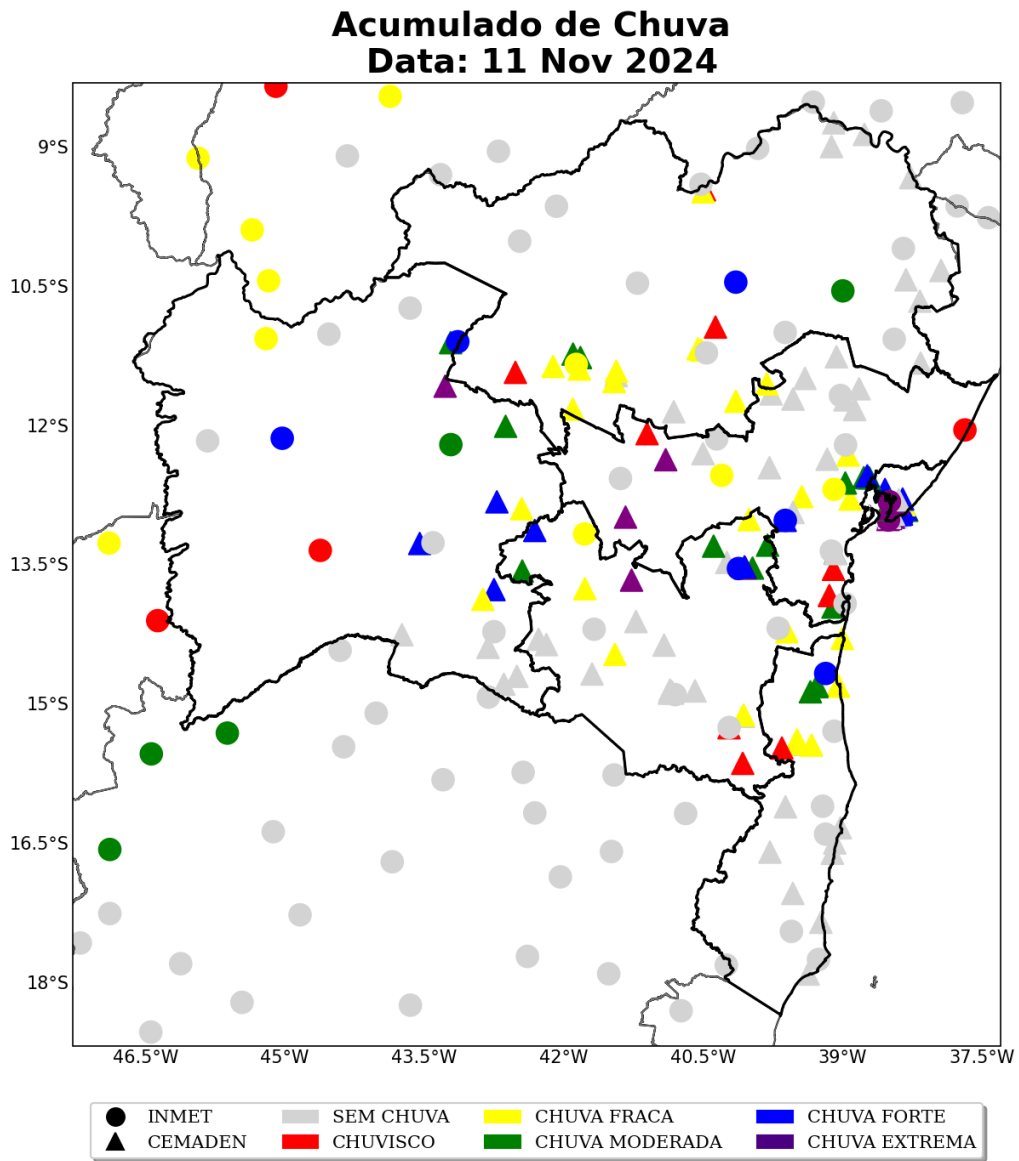
Figura 23: Acumulado diário de precipitação sobre o estado de Bahia para o dia 11 de novembro, baseado nas estações meteorológicas do INMET e CEMADEN.
