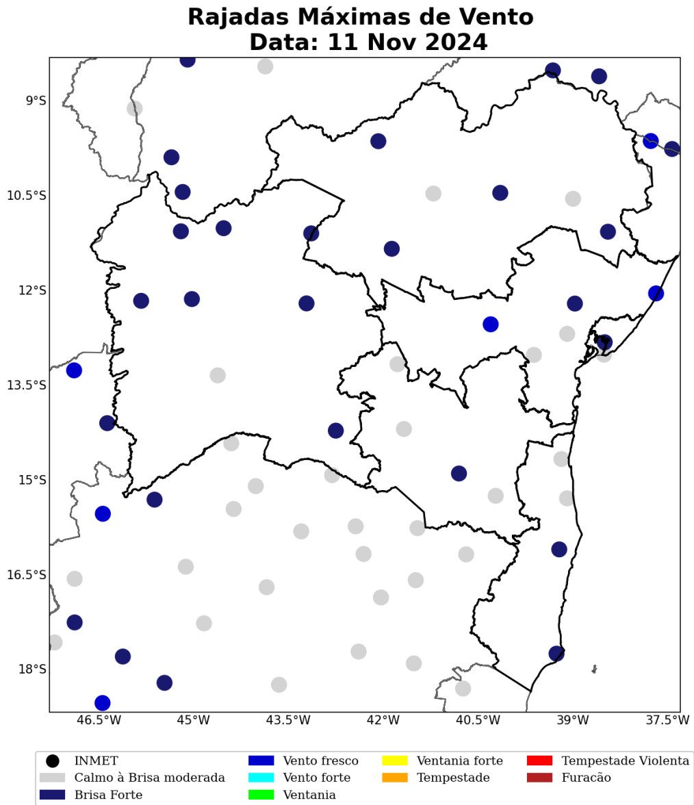
Figura 32: Rajada de vento sobre o estado de Bahia para o dia 11 de novembro, baseado nas estações meteorológicas do INMET.
