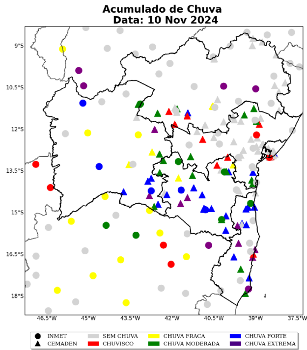
Figura 1 – Mapa de precipitação sobre o estado da Bahia no dia 10 de novembro.
