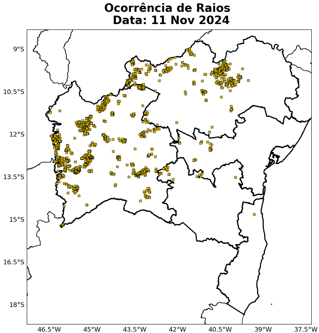
Figura 14: Ocorrência de descargas atmosféricas nuvem-solo detectadas pelo sistema Earth Networks para o dia 11 de novembro sobre a área de concessão da Neoenergia-COELBA.
