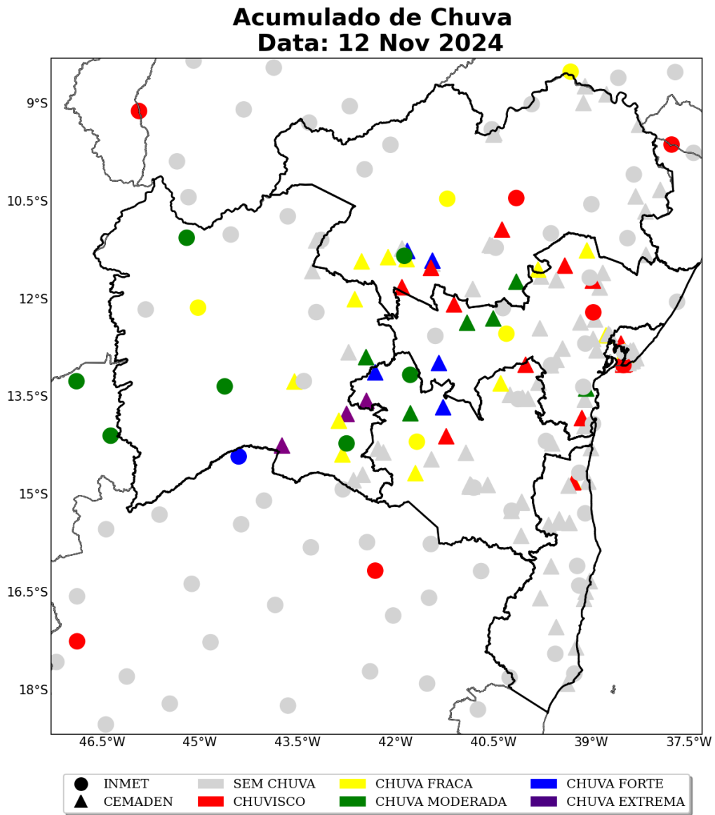
Figura 24: Acumulado diário de precipitação sobre o estado de Bahia para o dia 12 de novembro, baseado nas estações meteorológicas do INMET e CEMADEN.
