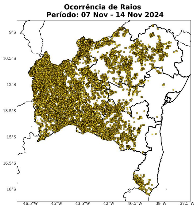
Figura 8 – Mapa de ocorrência de raios acumulado de 07 a 14 de novembro.
