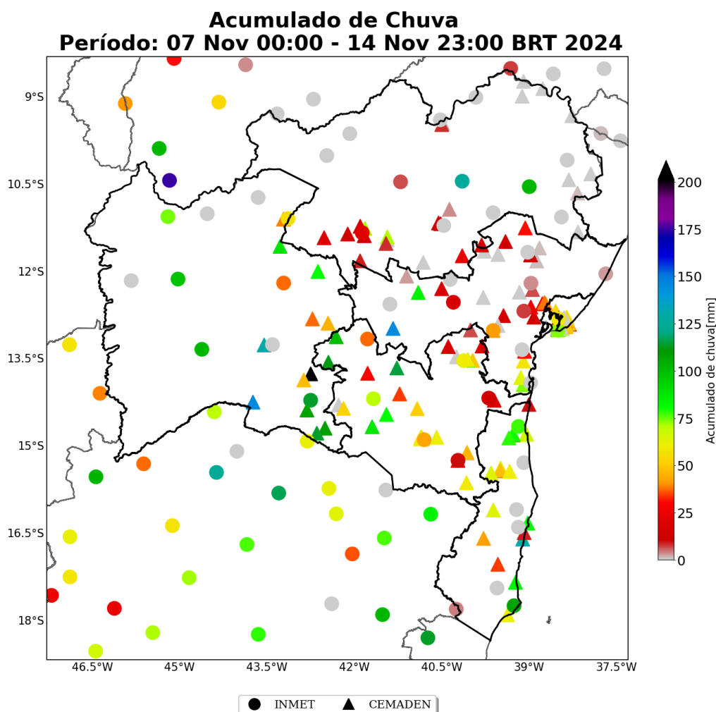
Figura 27: Acumulado de precipitação sobre o estado de Bahia para o período de 07 a 14 de novembro de 2024, baseado nas estações meteorológicas do INMET e CEMADEN.
