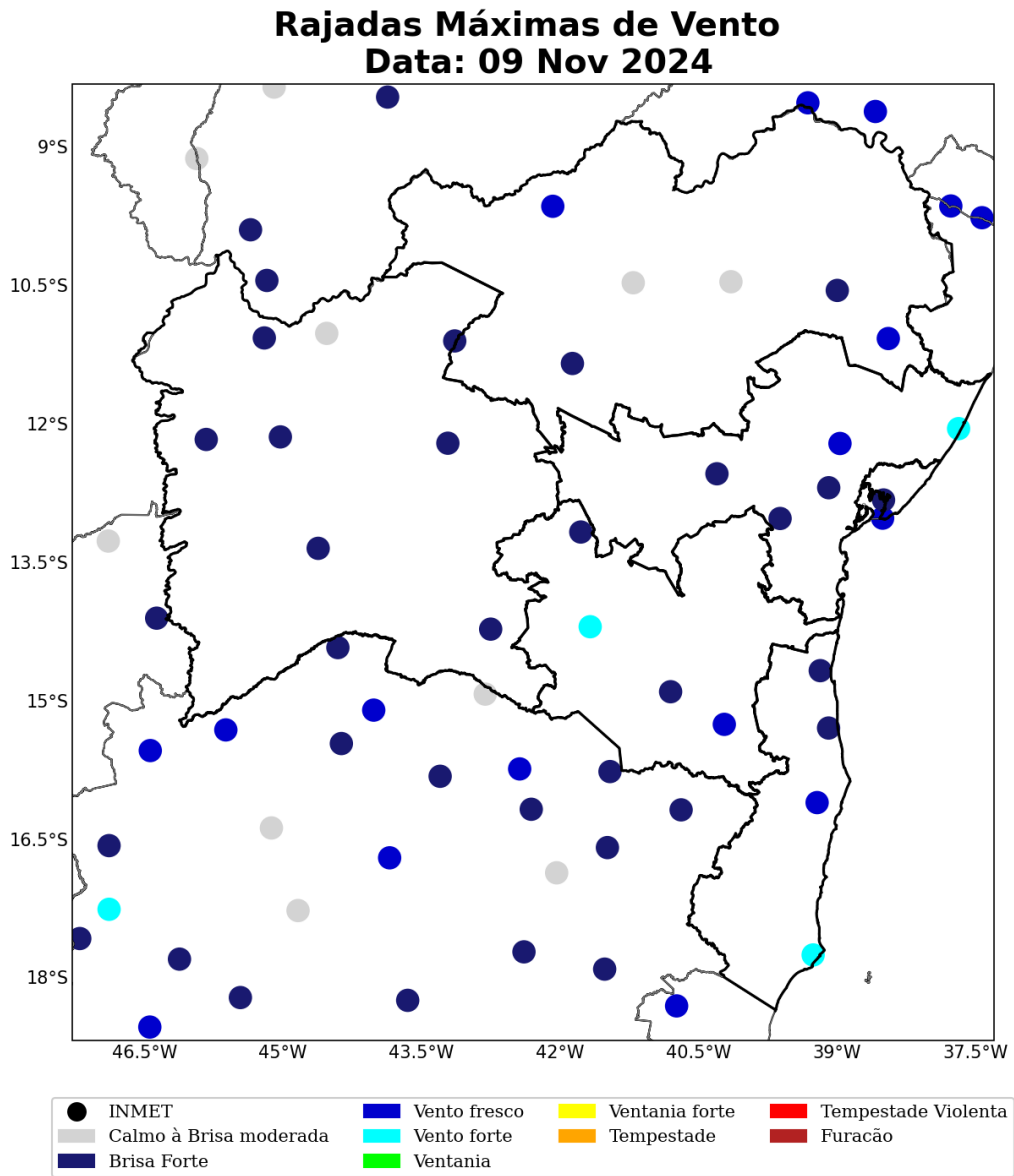
Figura 30: Rajada de vento sobre o estado de Bahia para o dia 09 de novembro, baseado nas estações meteorológicas do INMET.
