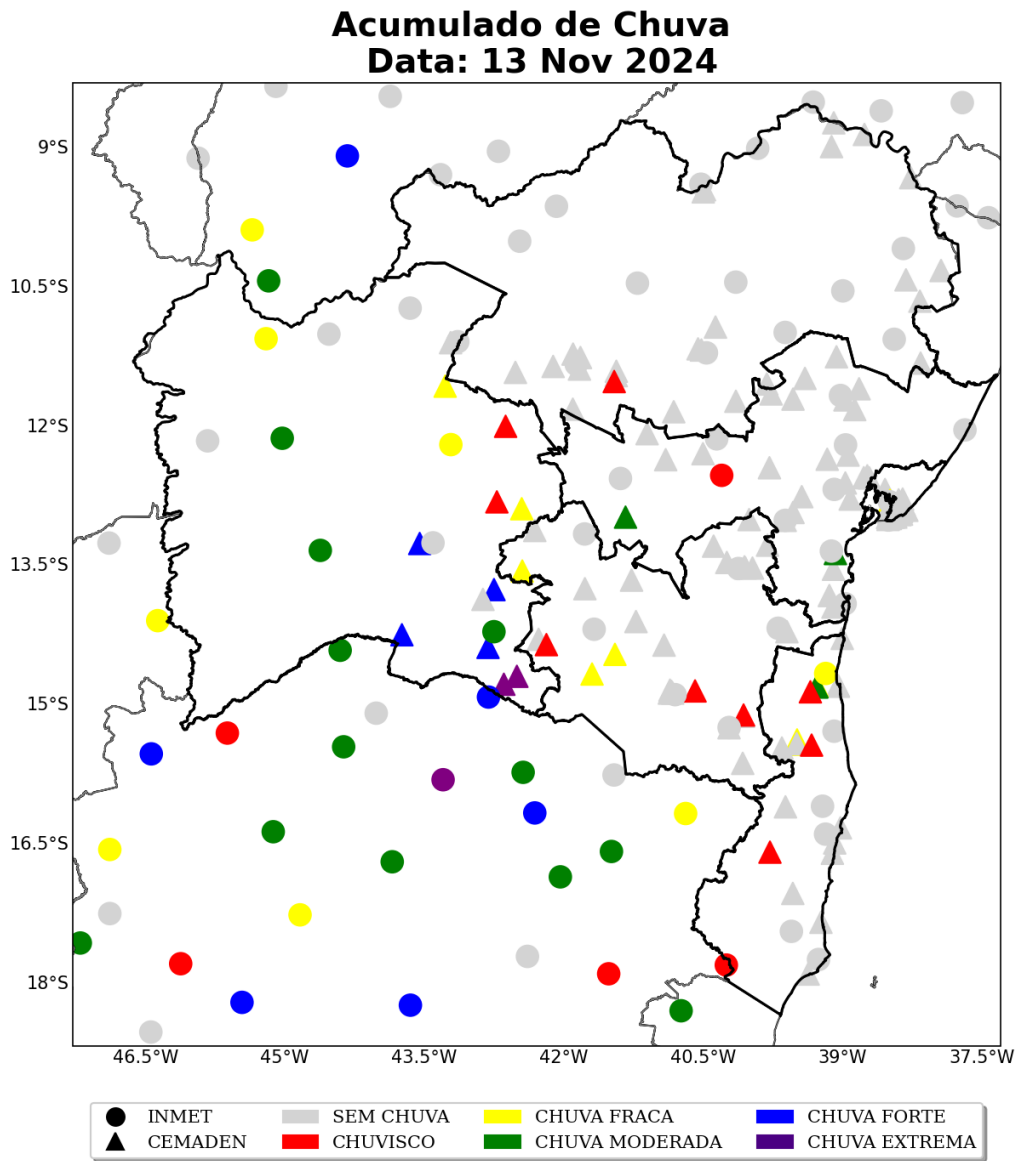
Figura 25: Acumulado diário de precipitação sobre o estado de Bahia para o dia 13 de novembro, baseado nas estações meteorológicas do INMET e CEMADEN.
