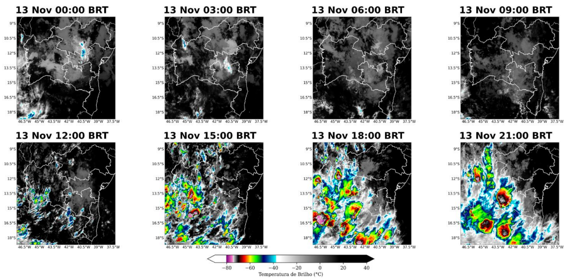
Figura 12 – Imagens realçadas do satélite GOES-16 das 00h00, 03h00, 06h00, 09h00, 12h00, 15h00, 18h00, e 21h00 do dia 13 de novembro de 2024. Fonte: Climatempo
