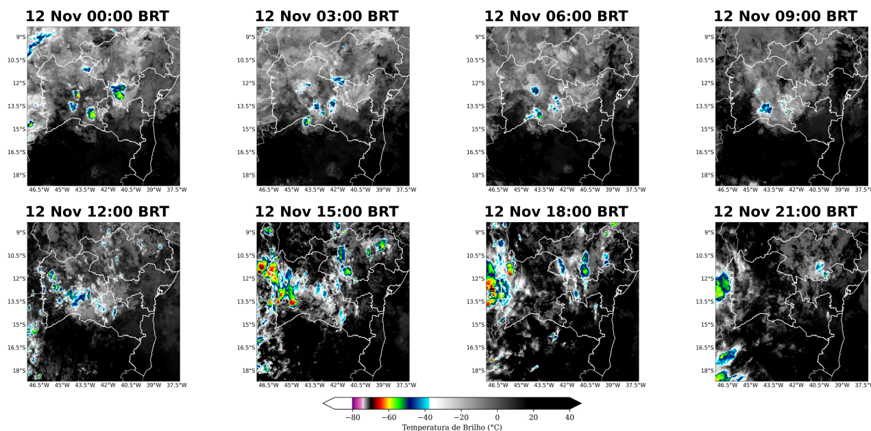
Figura 7: Imagens realçadas do satélite GOES-16 das 00 BRT até 21 BRT (a cada 3 horas) para o dia 12 de novembro.
