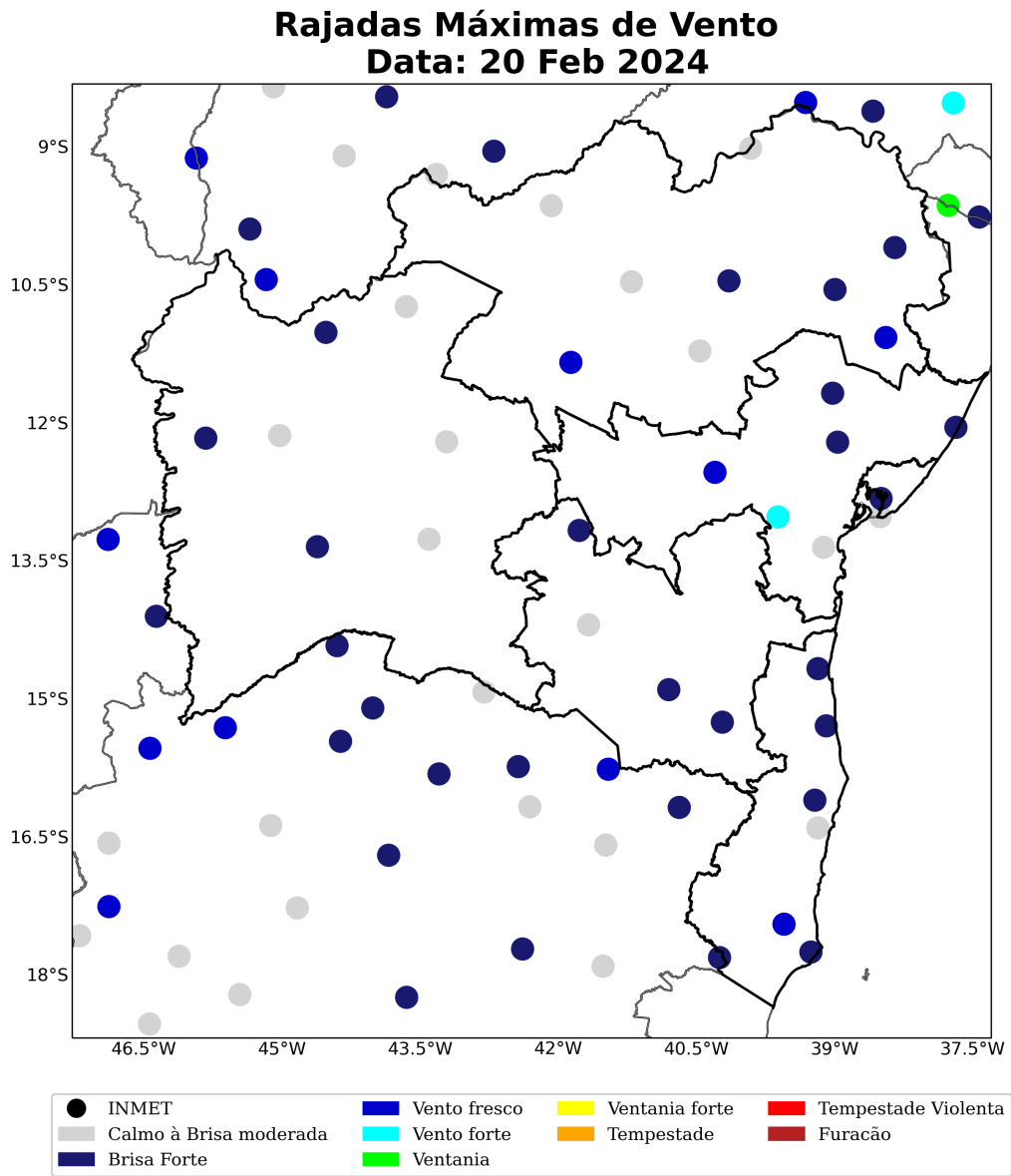
Figura 35: Rajada de vento sobre o estado de Bahia para o dia 20 de fevereiro, baseado nas estações meteorológicas do INMET.
