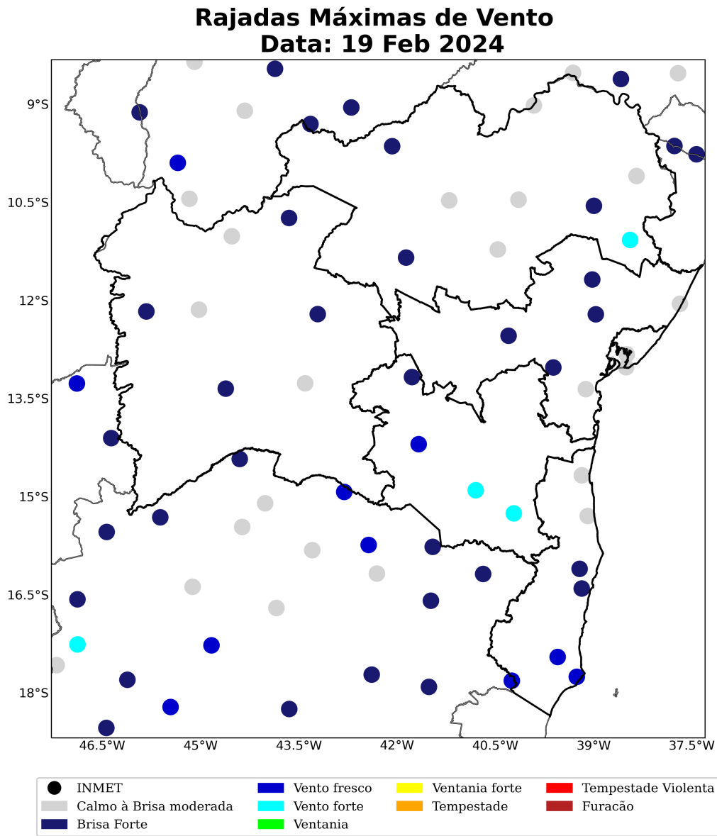
Figura 34: Rajada de vento sobre o estado de Bahia para o dia 19 de fevereiro, baseado nas estações meteorológicas do INMET.
