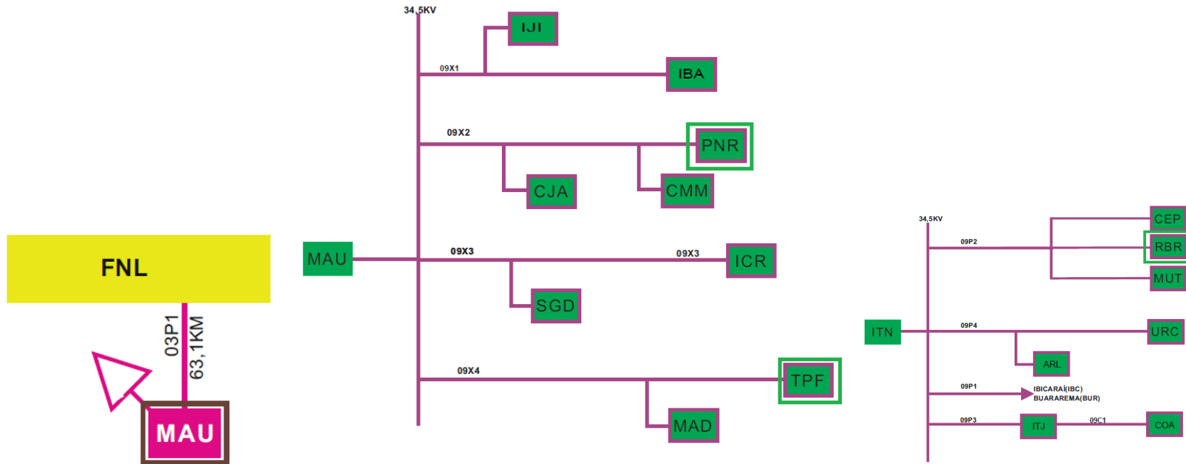
Figura 122 - Diagrama Unifilar Subtransmissão Funil CHESF (FNL)
