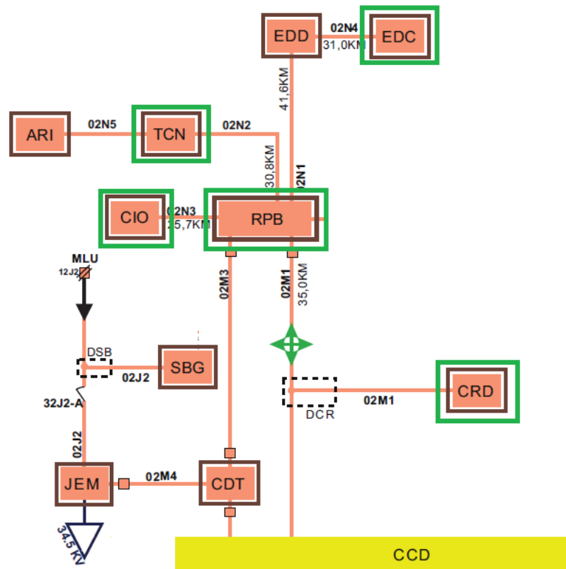
Figura 129 - Diagrama Unifilar Subtransmissão Cicero Dantas CHESF (CCD)
