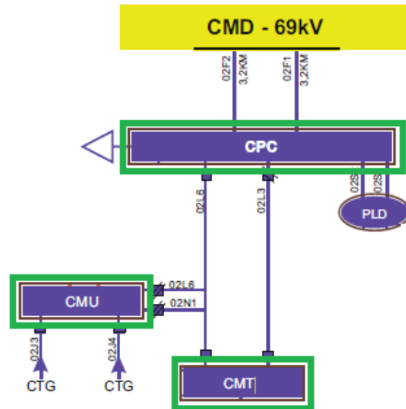
Figura 115 - Diagrama Unifilar Subtransmissão Camaçari II CHESF (CMD)
