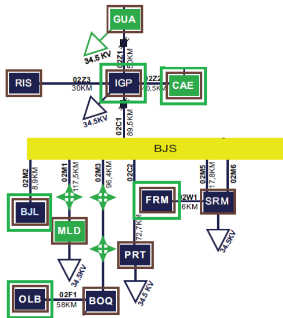
Figura 124 - Diagrama Unifilar Subtransmissão Bom Jesus da Lapa CHESF (BJS)
