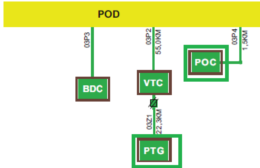
Figura 120 - Diagrama Unifilar Subtransmissão Poções II CHESF (POD)
