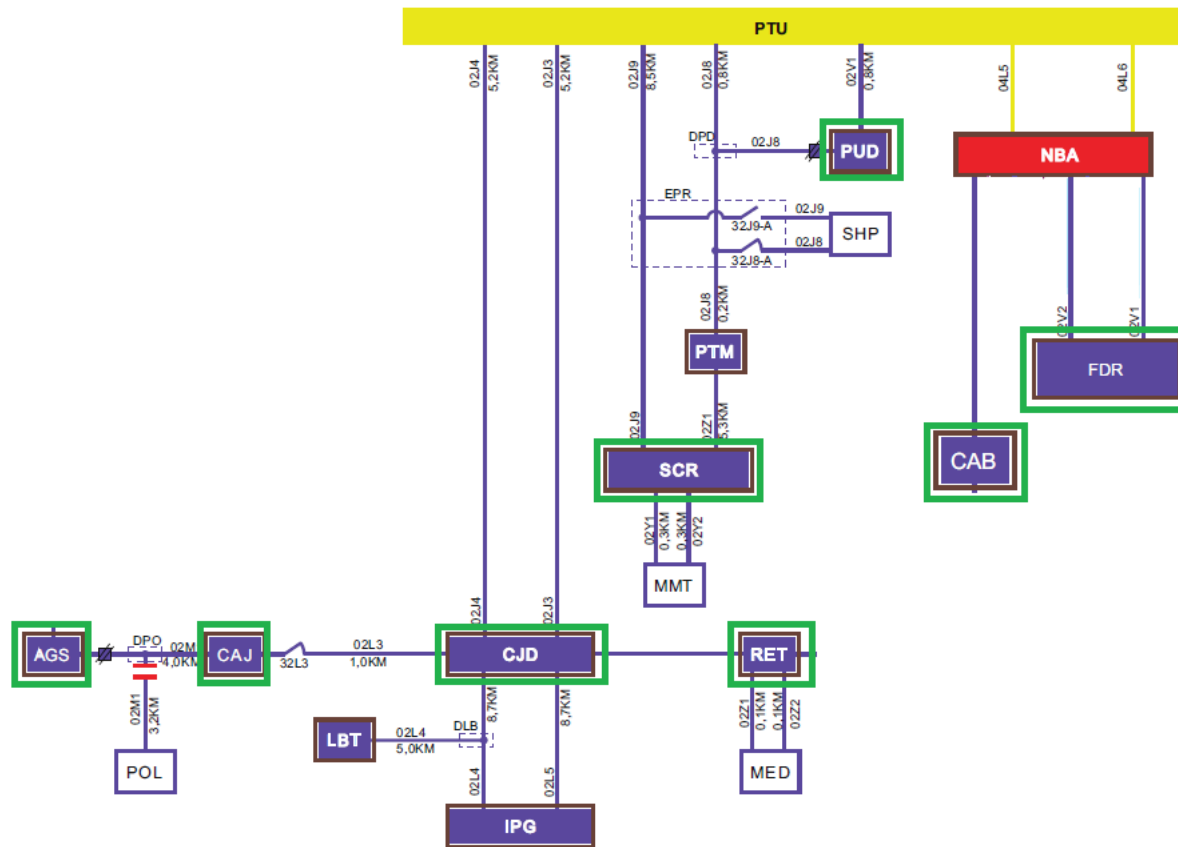
Figura 117 - Diagrama Unifilar Subtransmissão Pituáçu (PTU)
