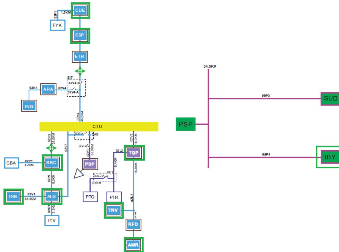
Figura 116 - Diagrama Unifilar Subtransmissão Catu CHESF (CTU)
