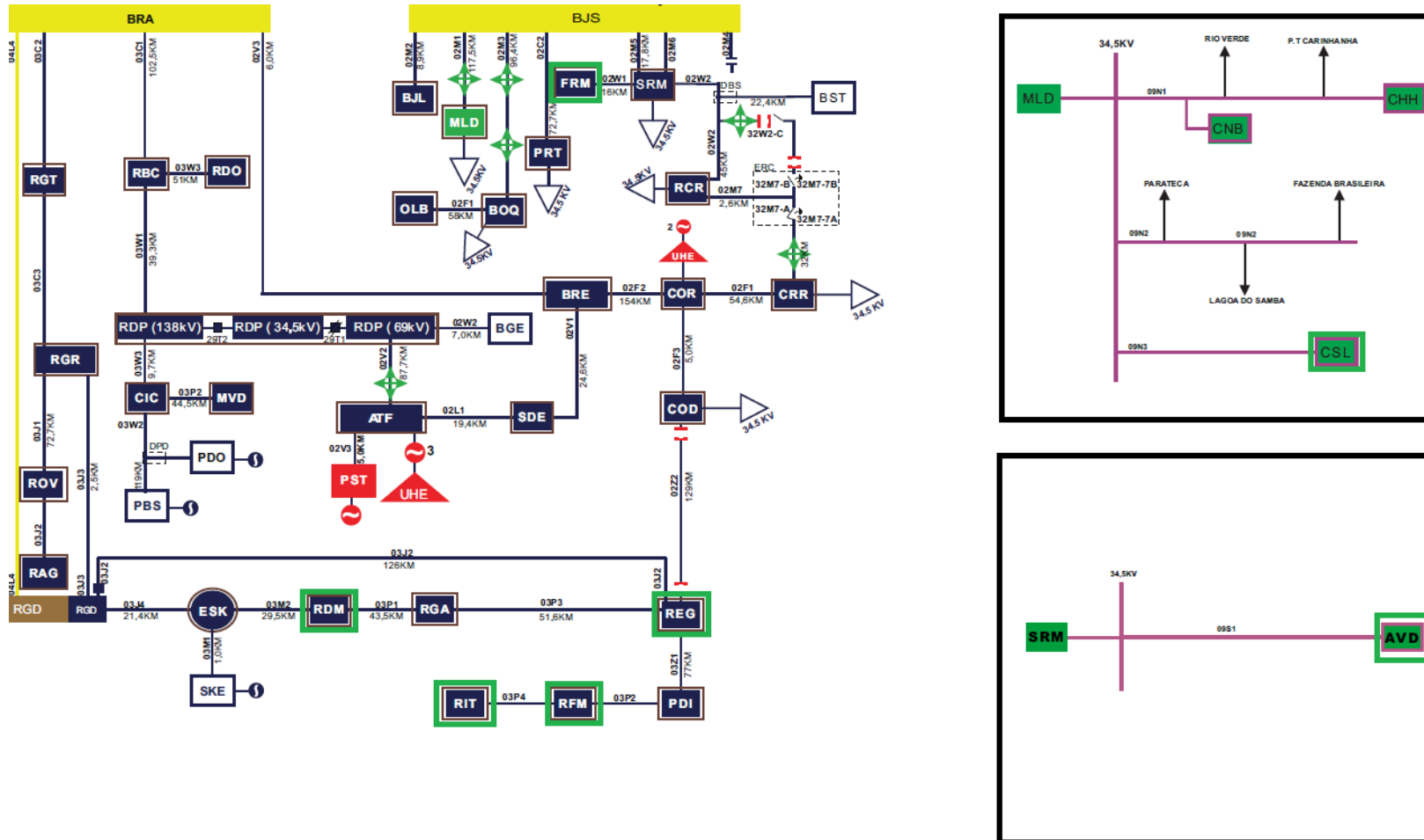
Figura 14 - Diagrama Unifilar Subtransmissão Barreiras CHESF (BRA) e Bom Jesus da Lapa CHESF (BJS)
