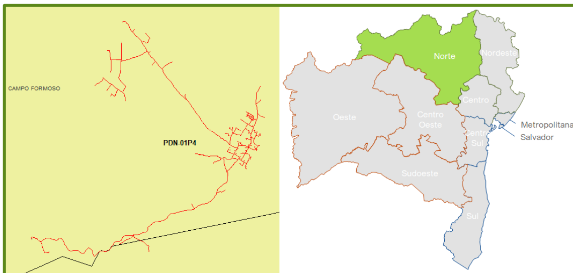
Figura 27 – Alimentador atingido da subestação Pedrinhas (PDN)
