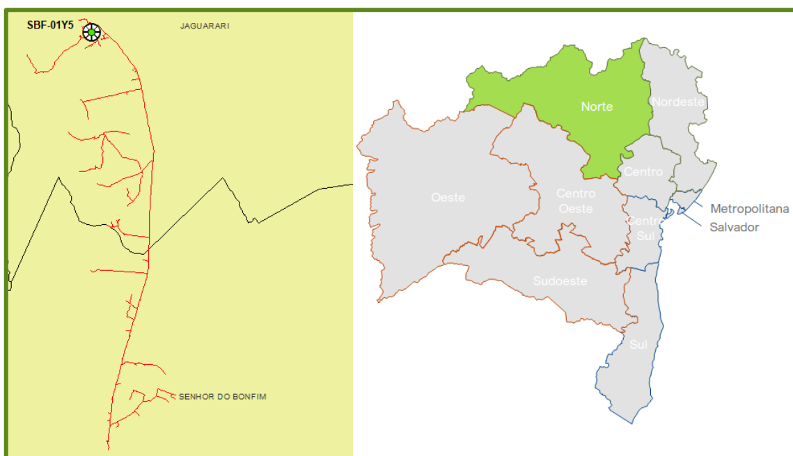
Figura 32 - Alimentador atingido da subestação Senhor do Bonfim (SBF)
