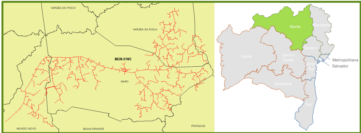
Figura 23 – Alimentador atingido da subestação Mundo Novo (MUN)
