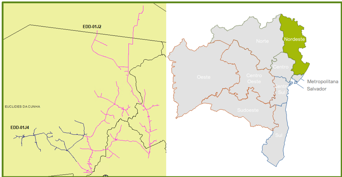
Figura 11 - Alimentadores atingidos da subestação Euclides da Cunha II (EDD)
