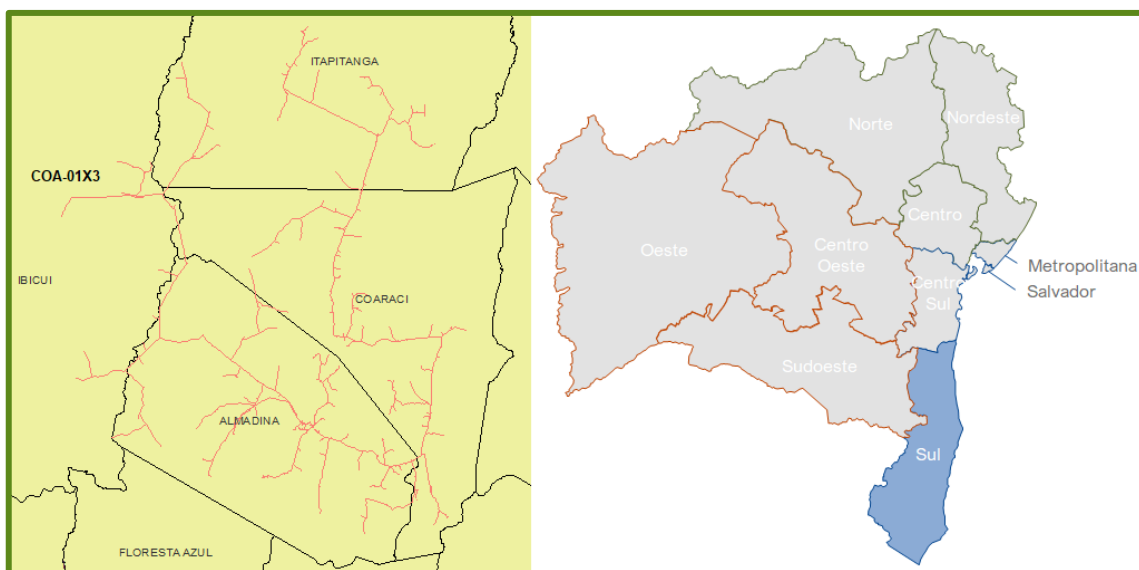
Figura 9 – Alimentador atingido da subestação Coaraci (COA)
