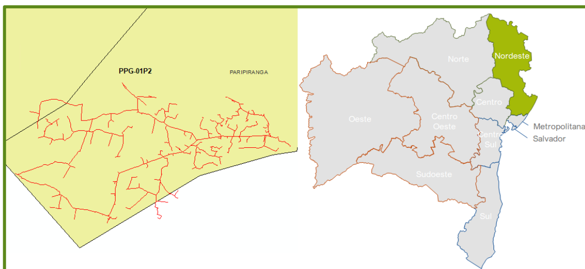
Figura 28 – Alimentador atingido da subestação Paripiranga (PPG)
