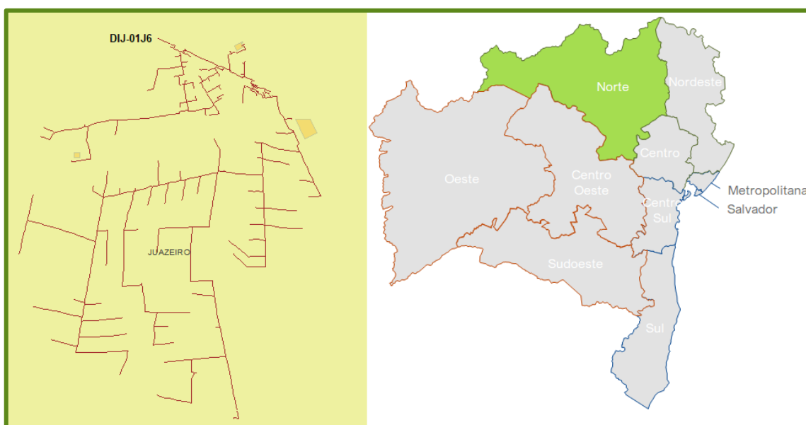
Figura 10 – Alimentador atingido da subestação Distrito Industrial de Juazeiro (DIJ)
