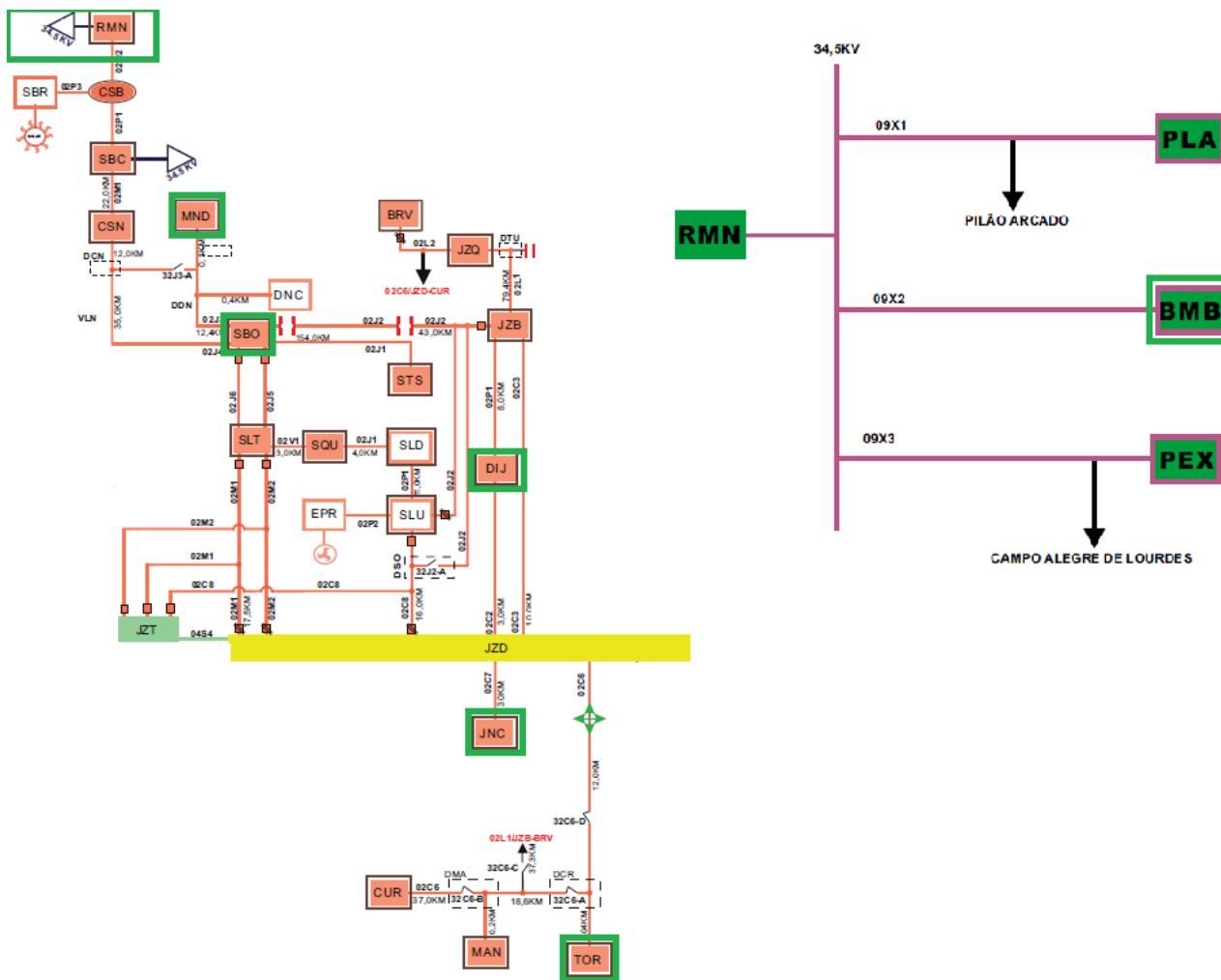
Figura 45 – Diagrama Unifilar Subtransmissão Juazeiro II CHESF (JZD)
