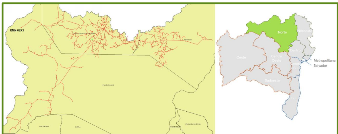
Figura 30 – Alimentador atingido da subestação Remanso (RMN)
