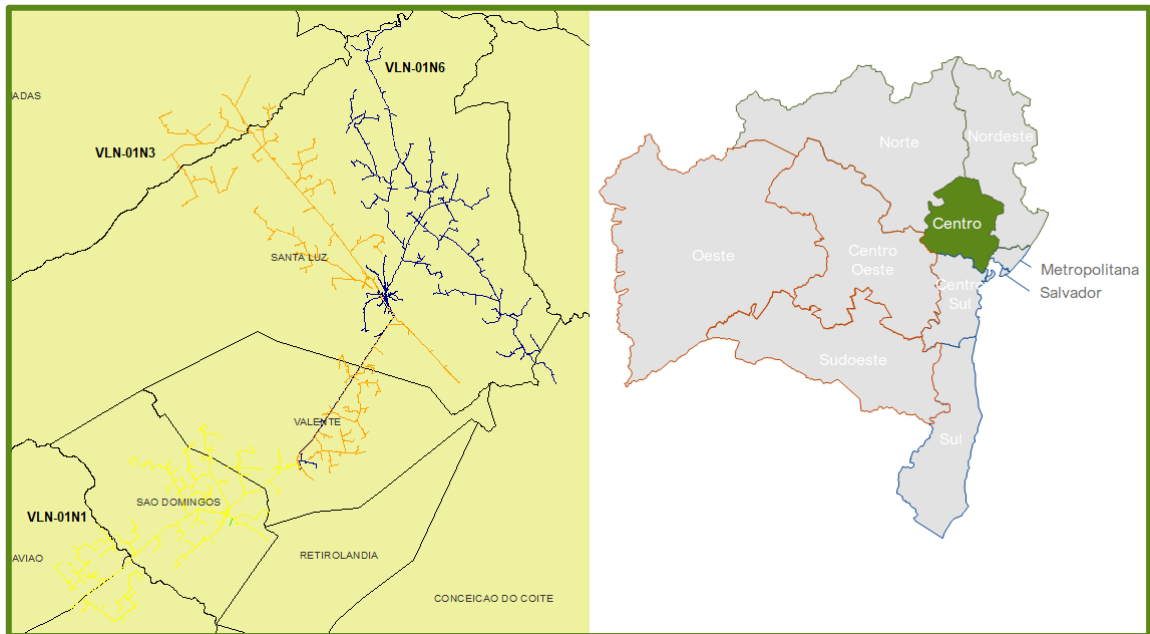
Figura 39 – Alimentador atingido da subestação Valente (VLN)
