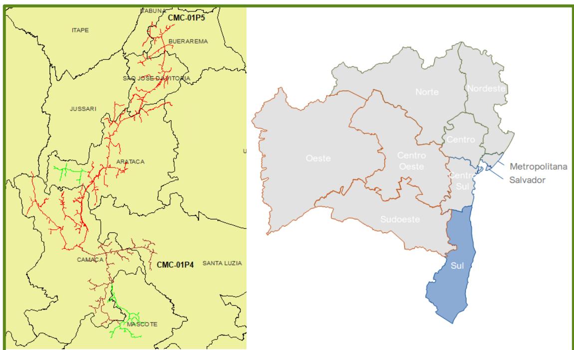
Figura 8 – Alimentadores atingidos da subestação Camaca (CMC)
