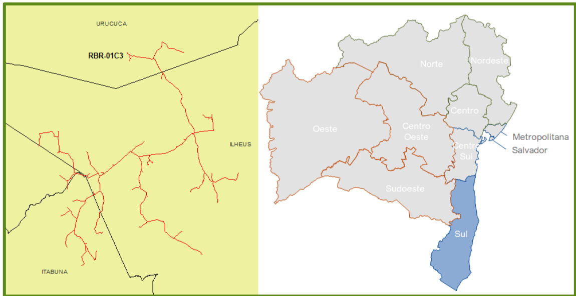
Figura 29 – Alimentador atingido da subestação Rio do Braço (RBR)
