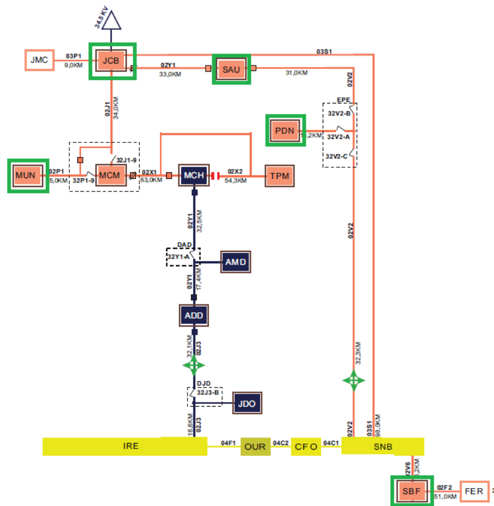
Figura 47 – Diagrama Unifilar Subtransmissão Senhor do Bonfim CHESF (SNB) e Irecê CHESF (IRE)
