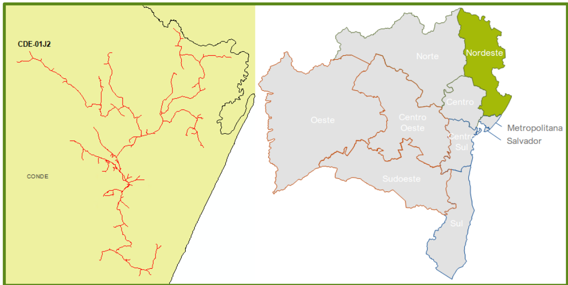
Figura 7 – Alimentador atingido da subestação Conde (CDE)
