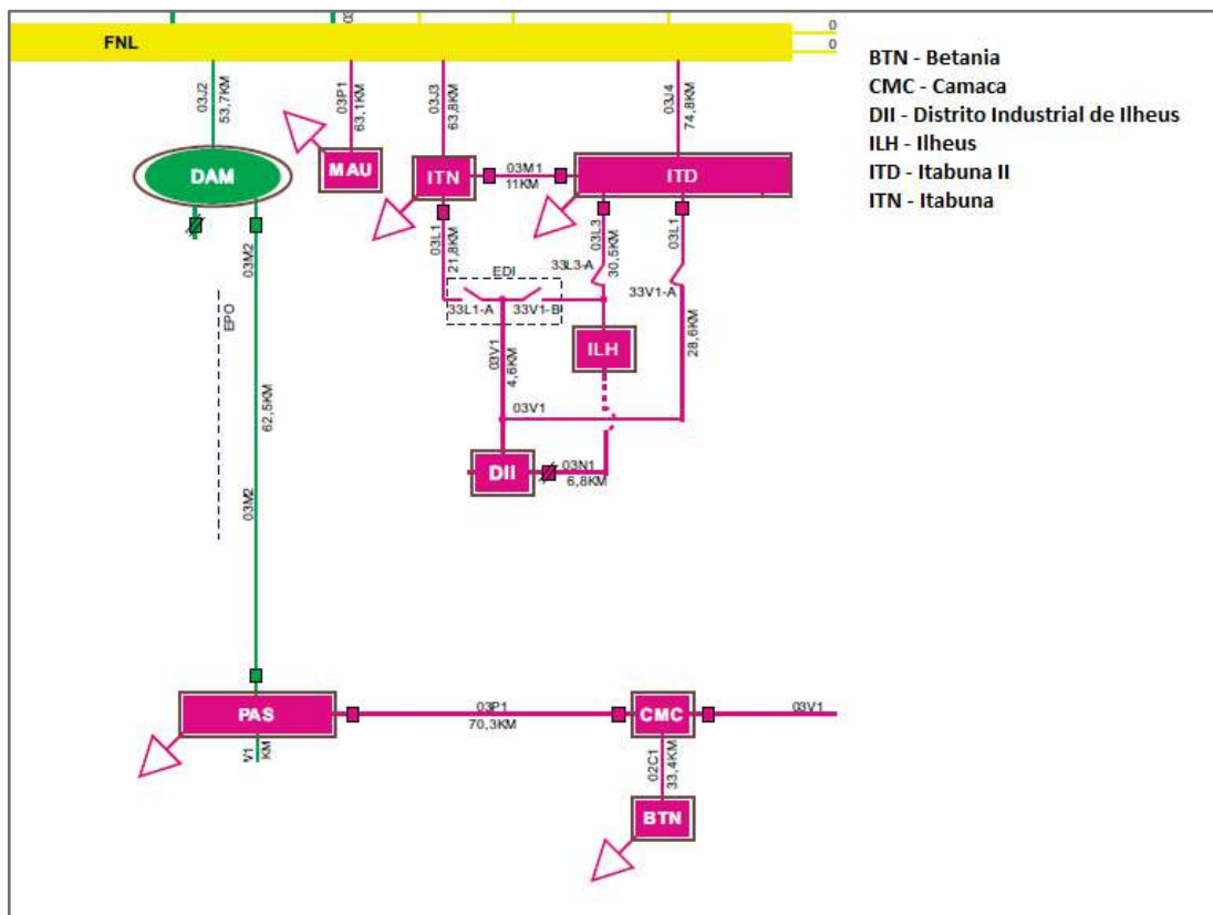
Figura 12 - Sistema de Alimentação da Região de Itabuna
