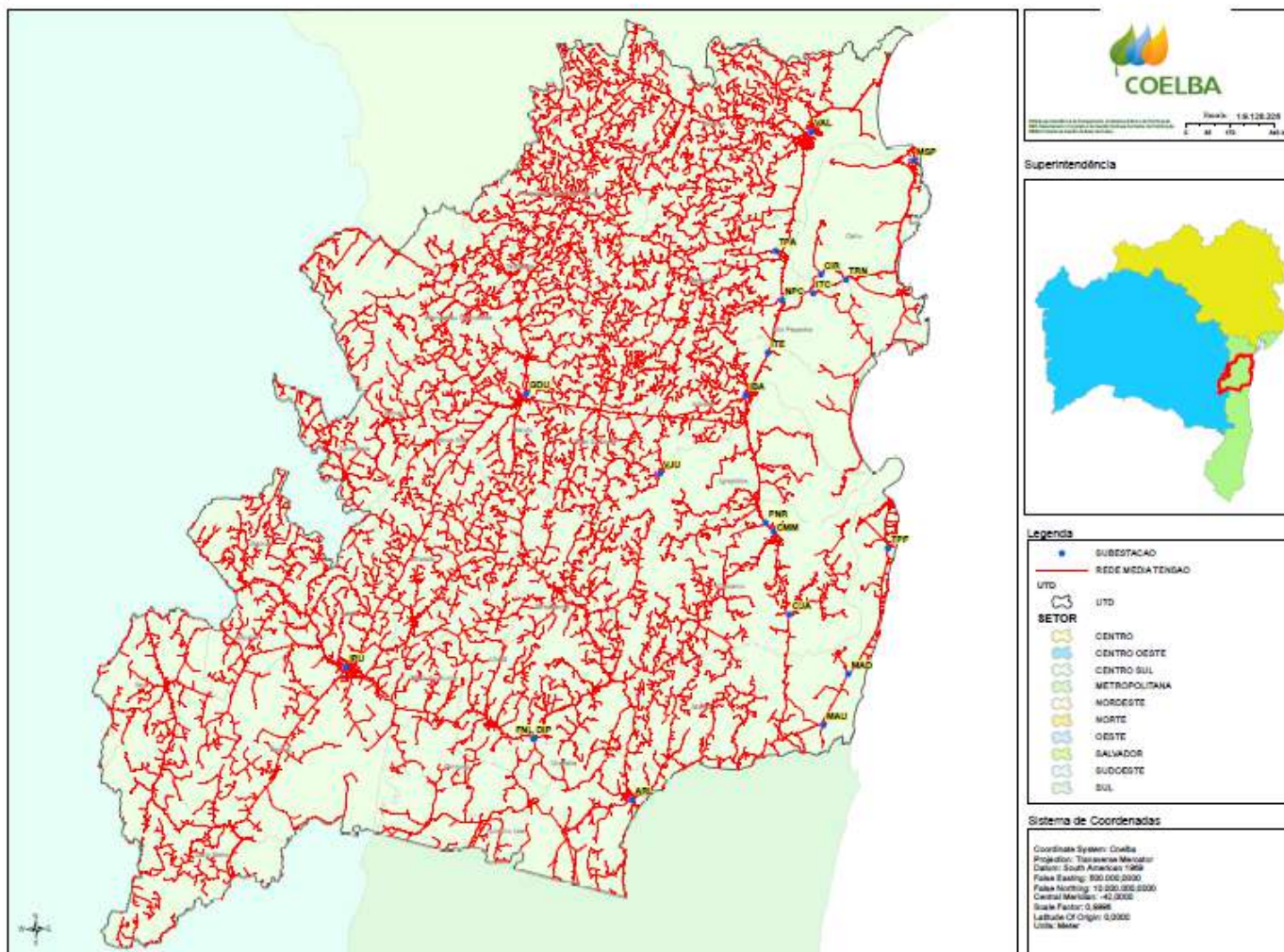
Figura 7 - Mapa Geométrico da Região de Valença
