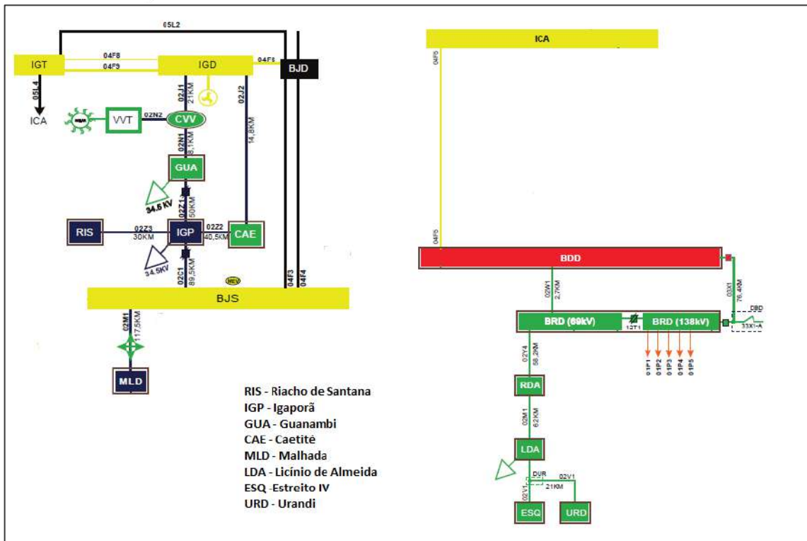
Figura 11 - Sistema de Alimentação da Região de Guanambi
