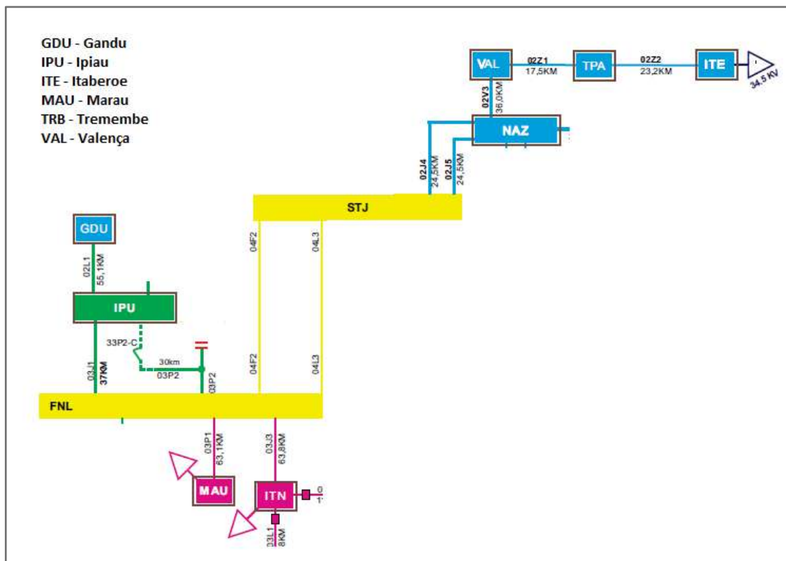
Figura 14 - Sistema de Alimentação da Região de Valença
