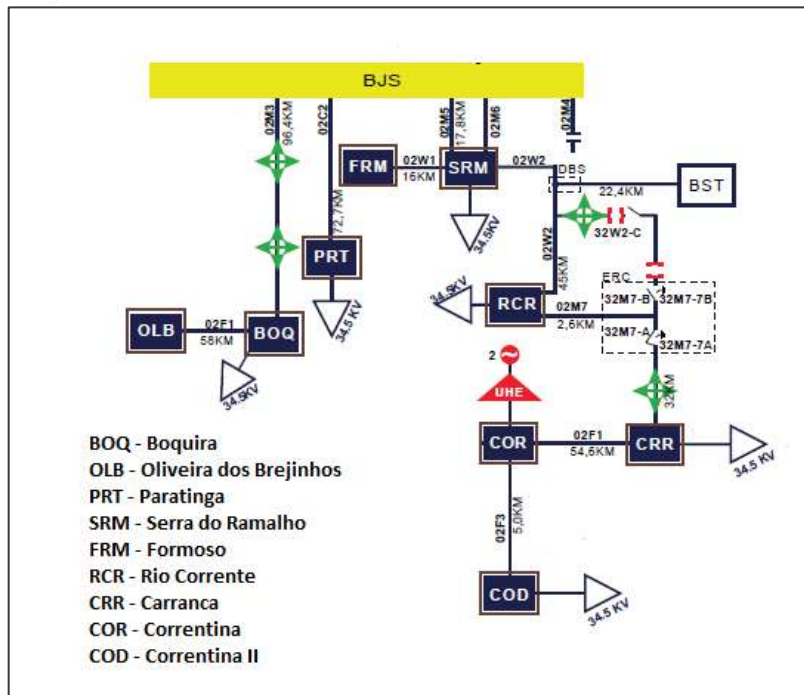
Figura 9 - Sistema de Alimentação da Região de Bom Jesus da Lapa
