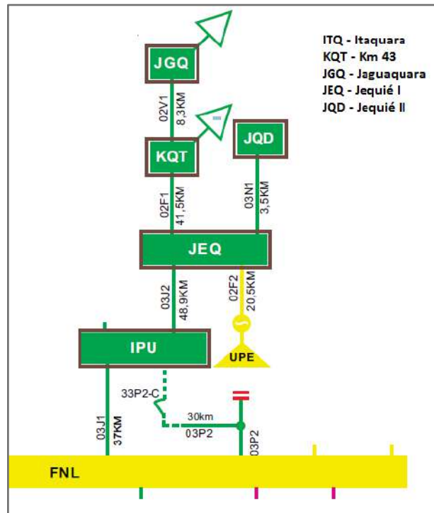
Figura 13 - Sistema de Alimentação da Região de Jequié
