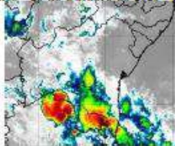
Figura 7 - Imagens realizadas do satélite GOES-16 das 23h00 do dia 25 de Outubro de 2020. FONTE: Cptec/INPE.
