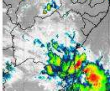
Figura 10 - Imagens realçadas do satélite GOES-16 das 5h00 do dia 26 de Outubro de 2020. FONTE: Cptec/INPE.
