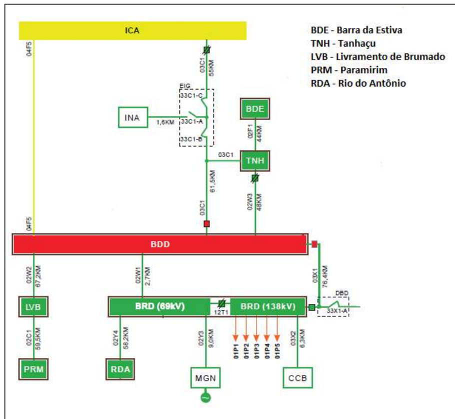
Figura 10 - Sistema de Alimentação da Região de Brumado
