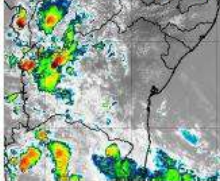
Figura 4 - Imagens realizadas do satélite GOES-16 das 15h00 do dia 25 de Outubro de 2020. FONTE: Cptec/INPE.
